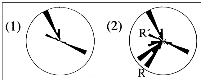
Abb. 9. Bruch- und Störungsflächen wurden in eine Rose eingetragen. Es treten dabei deutlich die konjugierten Scherflächensysteme heraus, die auch im Kartenbild zu sehen sind. Die Flächen der späteren Phase (frühe Phase siehe Abb. 7) der 1. Deformationsphase (Oligozän) zeigt eine SE/NW-Einengung (1). In der Rose (2) der 2. Deformationsphase (Miozän) kommt es zu sinistralen SW/NE verlaufenden Blattverschiebungen. Es können auf der 2. Rose die Riedl- und Antiriedlflächen dieser Phase erkannt werden. Die Flächen der 1. Deformationsphase wurden in die Rose (2) einbezogen, da diese wiederbetätigt wurden. Sigma 1 liegt bei dieser Phase WSW-ENE. Die Dehnung in NNW-SSE-Richtung konnte im Gelände durch das Aufgehen von im Oligozän gebildeten Stylolithenflächen sowie an Klüften belegt werden.
