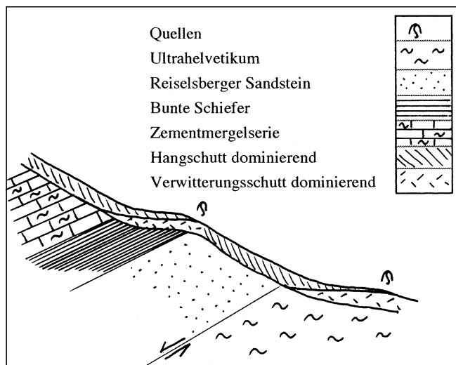
Abb. 5. Hydrogeologisches Modell für die Erklärung der Quellbildung im Zusammenhang mit mergel- und tonmergelreichen Gesteinen.
