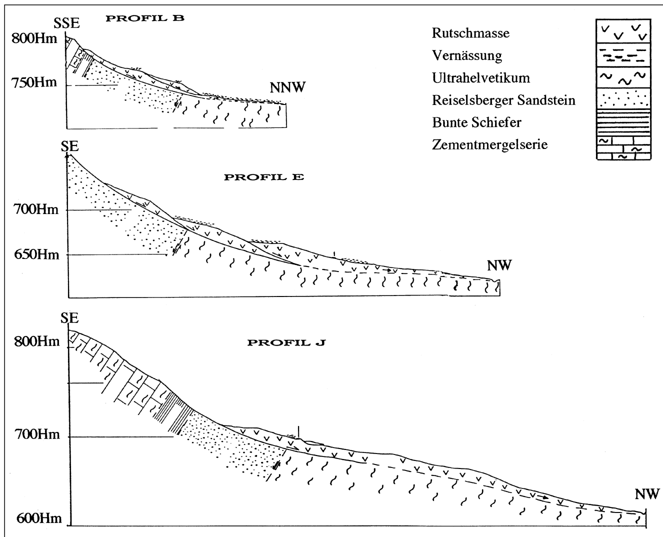
Abb. 7. Geomorphologische Profile der Erd- und Schuttströme B, E und J.
