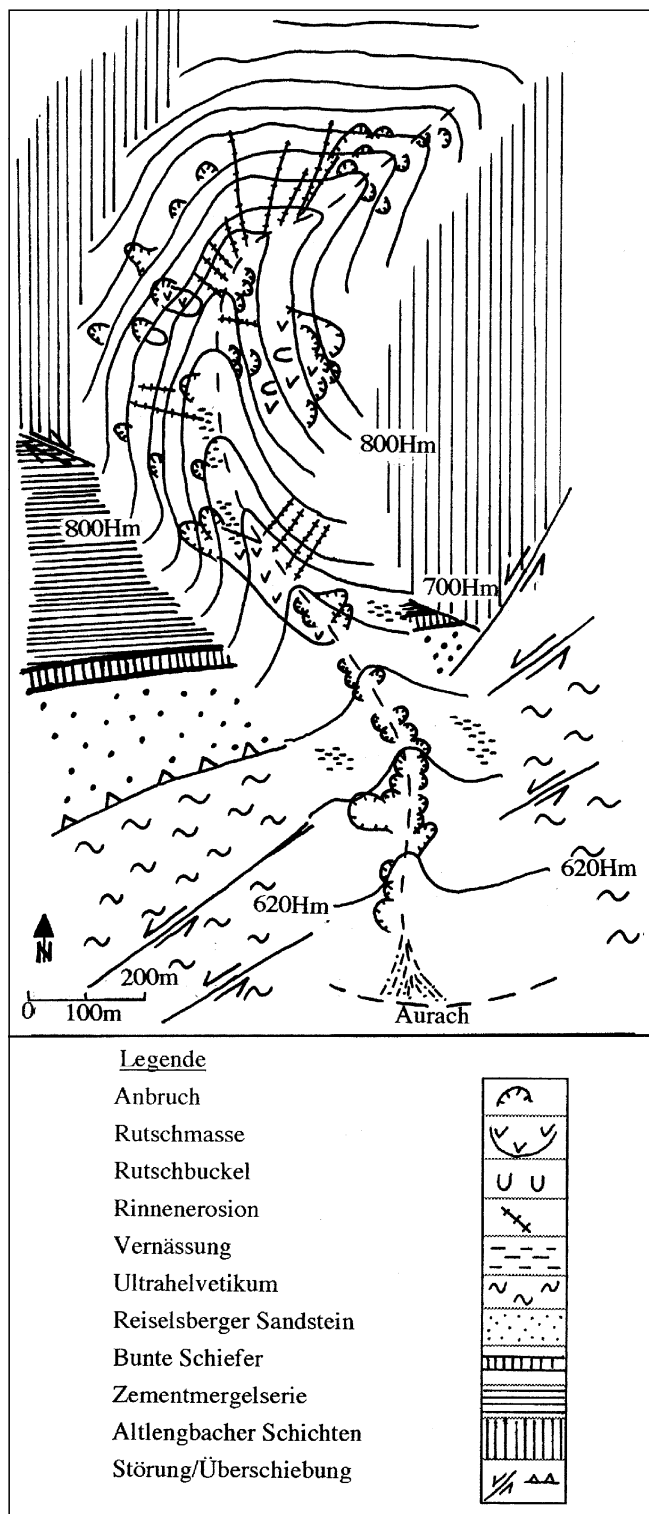
Abb. 4. Vereinfachte hangtektonische Situation des Herbstaugrabens. Man erkennt deutlich, daß im Ultrahelvetikum flache Hangneigungen und viele Rotationsrutschungen zum Bach hin auftreten. Im Flysch dagegen dominieren steilere Hänge mit Rotationsrutschungen, Erd- und Schuttströmen und Rinnenerosion.
