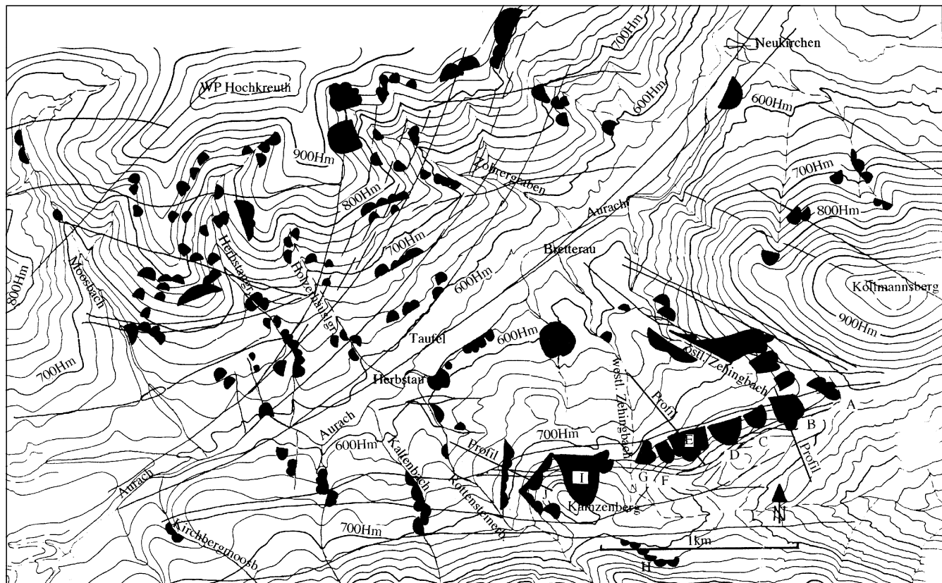
Abb. 6. Überblick über größere Massenbewegungen (Rotationsrutschungen, Erd- und Schuttströme) des Arbeitsgebietes. Auf der Abbildung wurden Störungen und Schichtgrenzen (vgl. geologische Karte Abb. 2) eingezeichnet, um Zusammenhänge zwischen Stratigraphie, Tektonik und Massenbewegungen aufzuzeigen. Deutlich ist dabei ein solcher zwischen Störungen und Massenbewegungen (v.a. im SE des Arbeitsgebietes) zu erkennen. Weiters zeigt die Abbildung, daß für Randcenoman, Ultrahelvetikum und Störungen meist eine flache Morphologie typisch ist, wogegen die Gesteine der Flyschzone meist steilere Hänge ausbilden.
