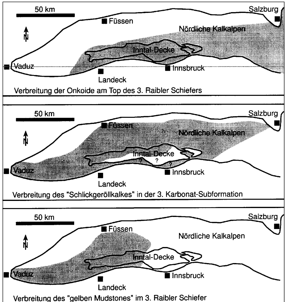
Abb. 10. Leithorizonte der Raibler Gruppe nach SCHWEIZER (1990), vereinfacht gezeichnet.
