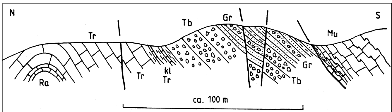
Abb. 2. Profilskizze durch die Permo-Trias des Koschuta-Zuges entlang des Forstweges im oberen Obojnkbachtal. Das Profil ist im nördlichen Drittel östlich des Obojnkbaches und in den südlichen zwei Dritteln westlich davon aufgeschlossen. Ra = Rattendorfer Schichten, Tr = Trogkofelkalk, kl Tr = klastische Trogkofelschichten, Tb = Tarviser Brekzie, Gr = Grödener Schichten, Mu = Muschelkalk, S = Schlern-Dolomit. Bellerophon-Dolomit und Werfener Schichten sind an der südlichsten Störung des Profils tektonisch ausgequetscht.
