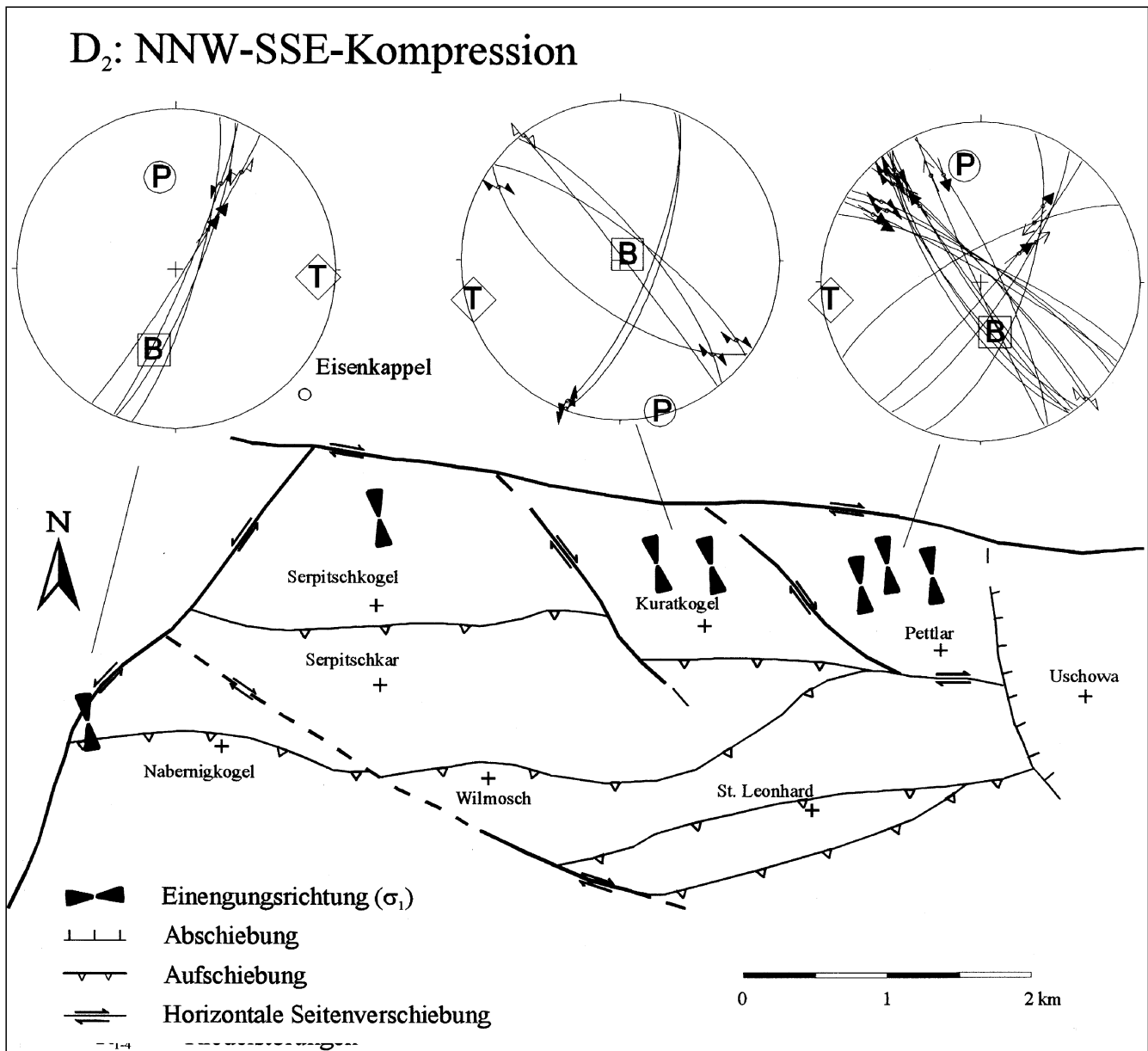
Abb. 5. Darstellung von Störungsflächendaten im Schmidtschen Netz, die eine NNW-SSE-gerichtete Kompression erkennen lassen und einer zweiten Deformationsphase zugeordnet werden können (D 2 ). P = Kompressionsachse, T = Dehnungsachse, B = neutrale Achse.
