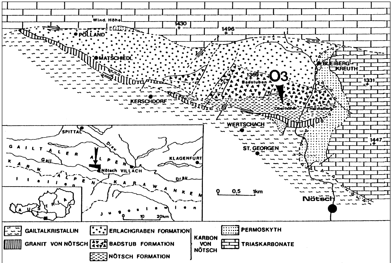
Abb. 1. Allgemeine geographische und geologische Übersicht über den Fossilfundpunkt SCHÖNLAUB 1 im Bereich des Oberhöherers bei Nötsch. Entommen und leicht verändert aus: KRAINER (1992: Abb. 1). O3 = Fundpunkt SCHÖNLAUB 1.
