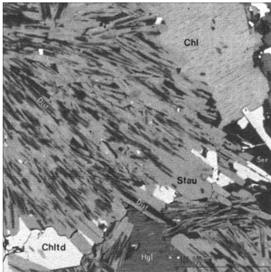
Abb. 14. Backscattered Aufnahme einer St 2 /D 1 -Pseudomorphose nach St 1 . St 2 überwächst Ky 1 , von dem noch schmale Leisten in St 2 erhalten sind. NM92/22a.
