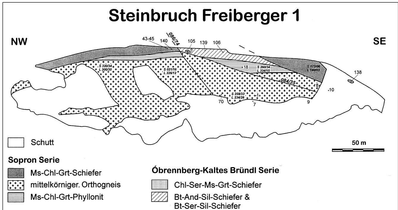
Abb. 4. Lithologische Situation im Freiburger Steinbruch mit der Lage der Probenpunkte.
