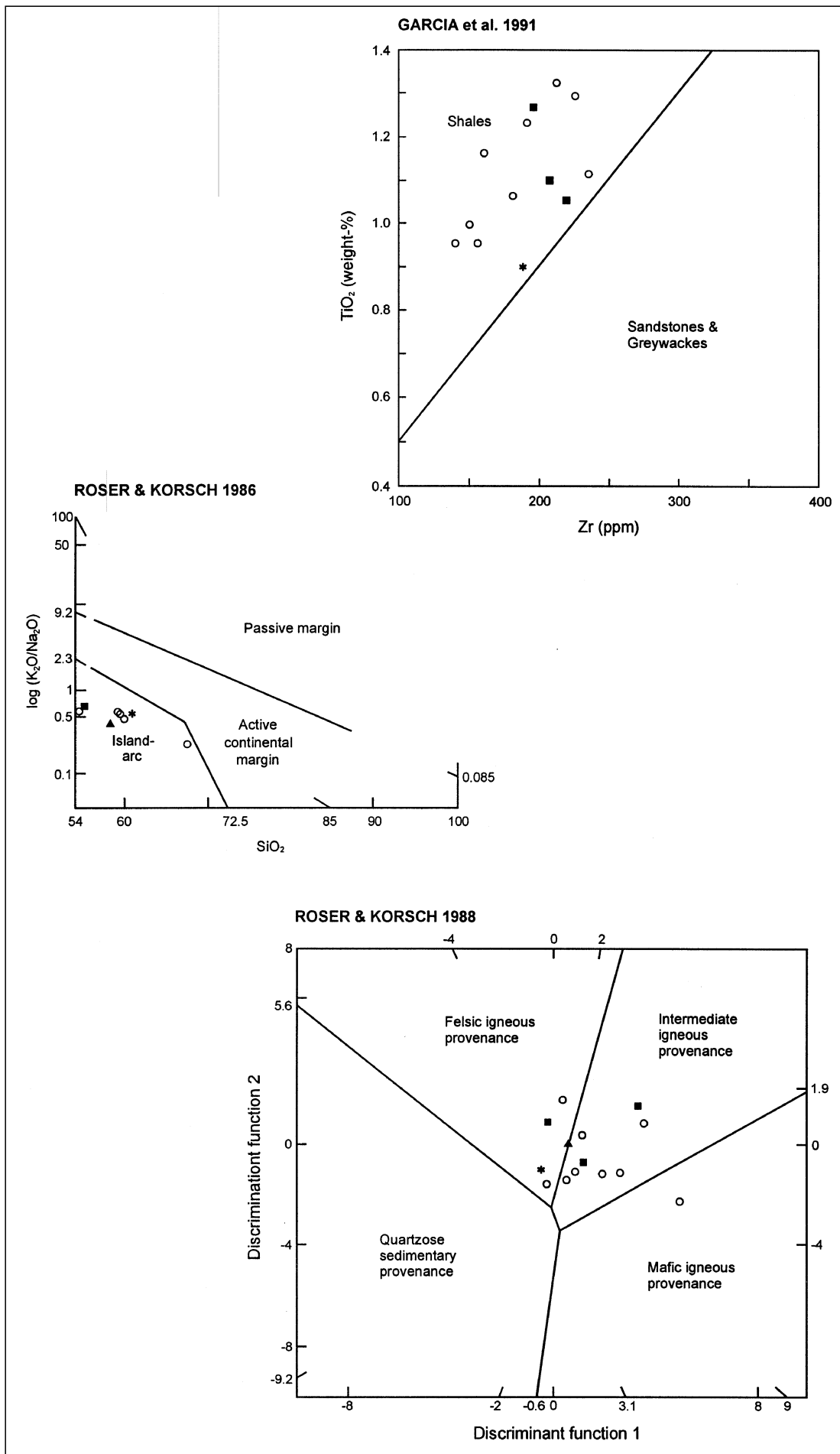
Abb. 13. Haupt- und Spurenelement-Diskriminations-Diagramme der Glimmerschiefer. ○ = Glimmerschiefer der Sopron-Serie. ★ = Biotit-Andalusit-Sillimanit-Schiefer. ▲ = Biotit-Serizit-Chloritoid-Granat-Schiefer. ■ = Chlorit-Serizit-Granat-Schiefer.
