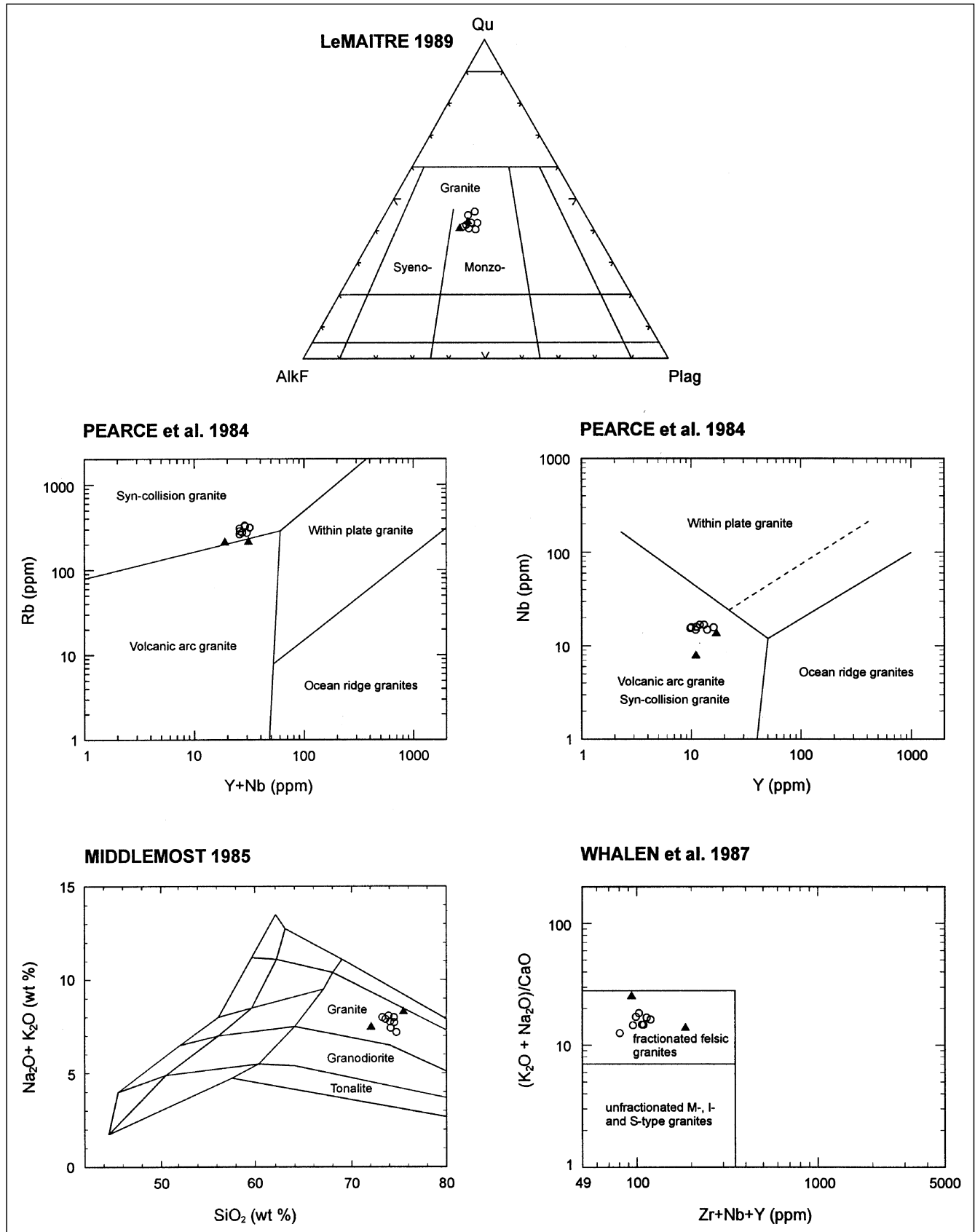
Abb. 11. Haupt- und Spurenelement-Diskriminations-Diagramme. ▲ = Grobgneis; ○ = mittelkörniger Orthogneis.
