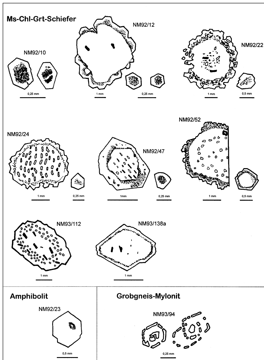
Abb. 7. Granatmorphologie. Die Granate in den Schiefen der Sopron-Serie sind durchwegs 2-phasig, mit einem einschlussarmen Kern und einer durch einen Pigmentsaum abtrennbaren, jüngeren Generation.
