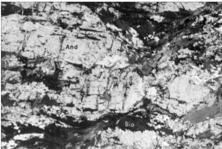
Abb. 6. Biotit-Andalusit-Sillimanit-Schiefer mit großen, porphyroblastischen Andalusiten, in deren Spaltrissen großer Hellglimmer wächst. Sillimanit findet sich bevorzugt in Scherbändern. Im Andalusit in der linken, oberen Bildhälfte sieht man einen quarzgefüllten Korrosionsschlauch. NM92/71; Bildbreite 16 mm; parallele Polarisatoren.
