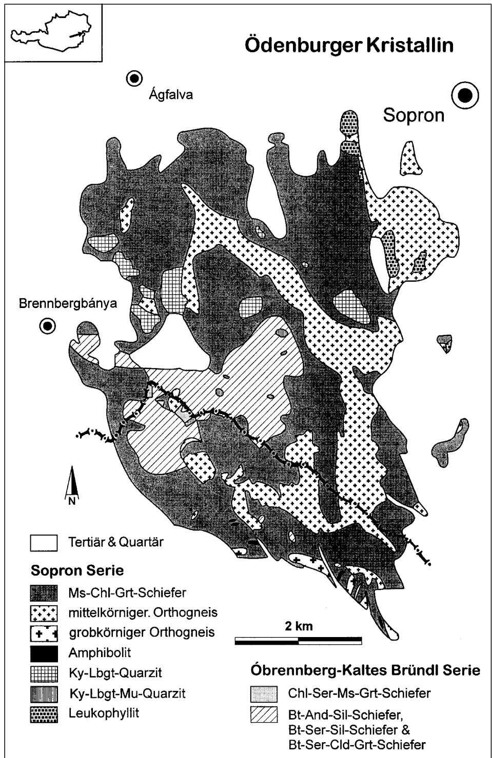
Abb. 2. Geologische Übersichtskarte des Ödenburger Kristallins nach KISHÁZI & IVANCSICS (1985) und DRAGANITS (1996).
