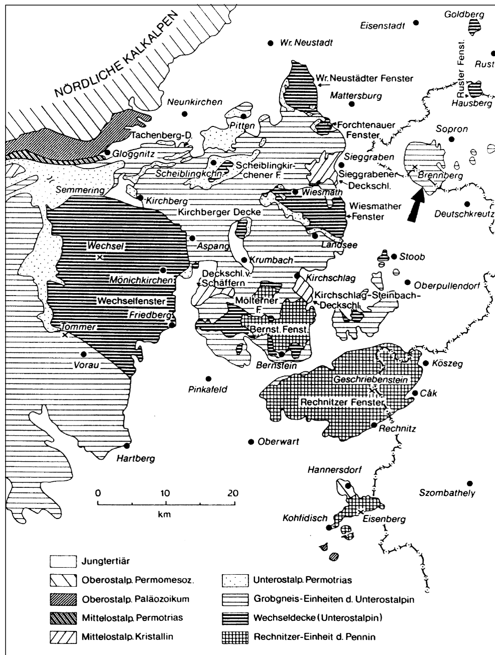
Abb. 1. Tektonische Übersicht des Nordostendes der Zentralalpen (aus HERRMANN & PAHR, 1988) mit der Lage des Kartierungsgebietes.
