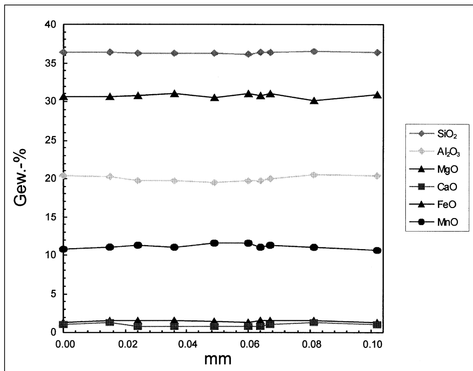
Abb. 10. Mikrosonden-Profil durch einen Granat eines Biotit-Serizit-Sillimanit-Schiefers (NM92/20b).
