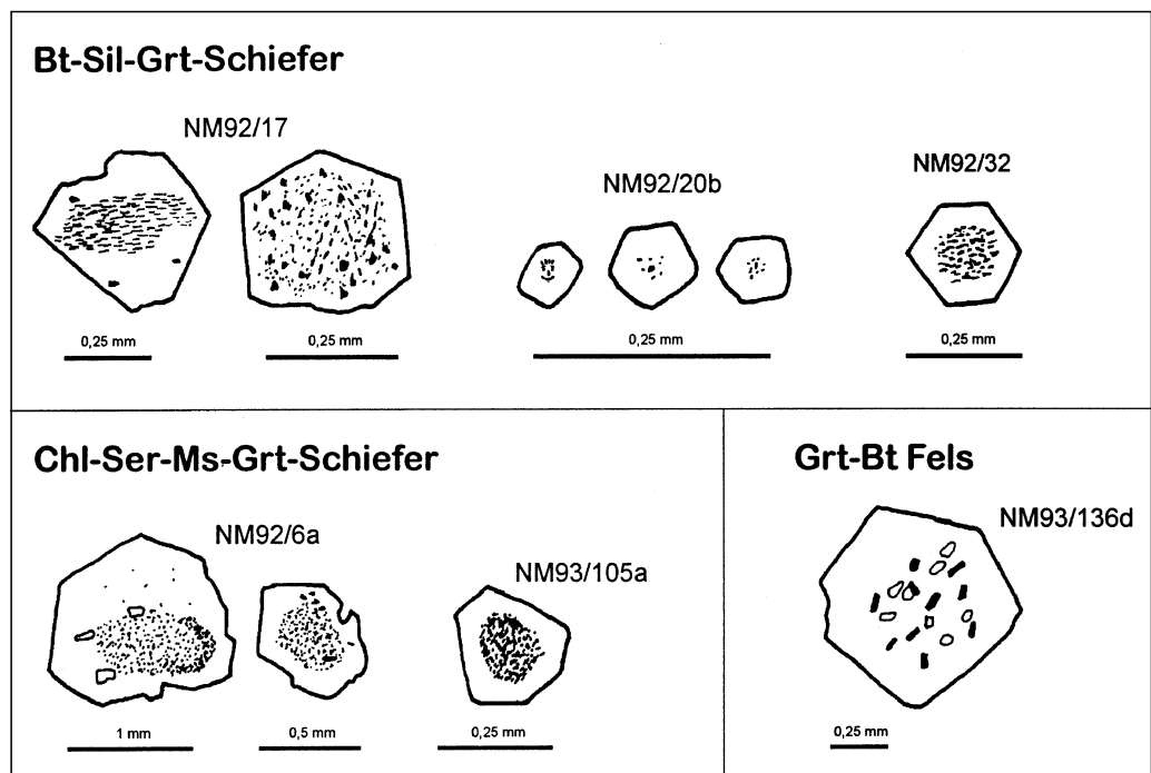
Abb. 9. Die Granate der Óbrennberg-Kaltes-Bründl-Serie sind ausschließlich 1-phasig-idioblastisch mit einschlussreichem Kern und klarem Rand und deutlich kleiner als die 2-phasigen Granate der Sopron-Serie.
