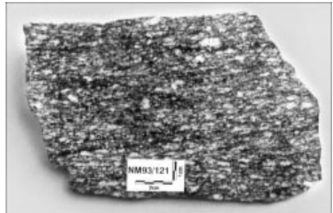
Abb. 5. Handstück eines mittelkörnigen Orthogneises („Sopron type gneiss“) mit der typisch-einheitlichen Korngröße der Kalifeldspäte. Bei genauem Hinsehen erkennt man die kleinen, idioblastischen Granate (x-z-Schnitt).
