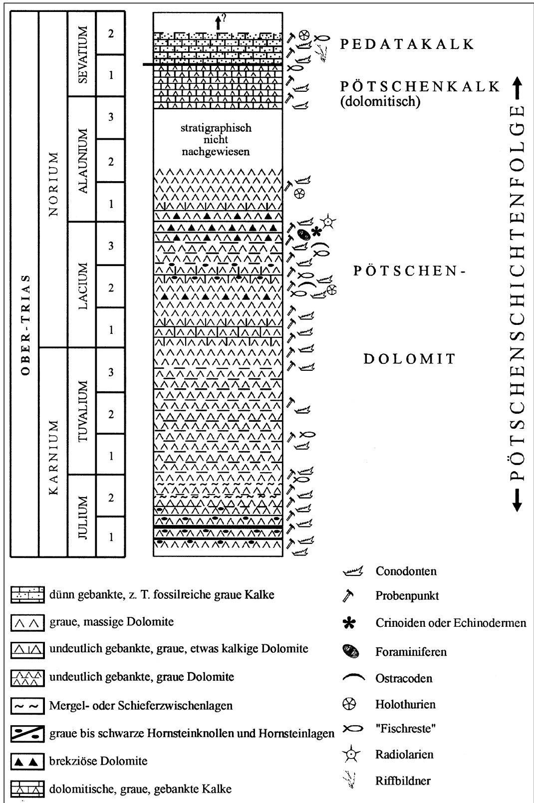
Abb. 8. Rekonstruktion der litho- faziellen und stratigraphi- schen Entwicklung der Pötschenschichtenfolge im Bereich der Lammer- egg-Südscholle aus ver- schiedenen Teilprofilen und den Ergebnissen der stratigraphischen und fa- ziellen Detailkartierung des Lammeregg-Schollen- komplexes. Belegmaterial, Proben- nummern: siehe Kap. 7.
