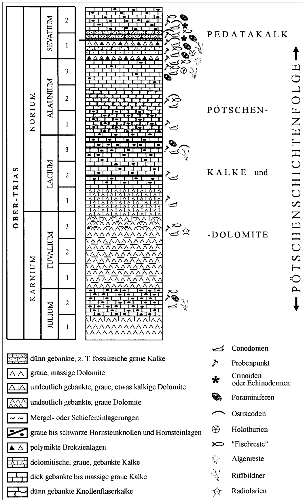
Abb. 6. Rekonstruktion der lithofaziellen und stratigraphischen Entwicklung der Pötschenschichtfolge im Bereich der Lammeregg-Nordscholle aus verschiedenen Teilprofilen und den Ergebnissen der stratigraphischen und faziellen Detailkartierung des Lammeregg-Schollenkomplexes. Belegmaterial und Probennummern siehe Kapitel 7.
