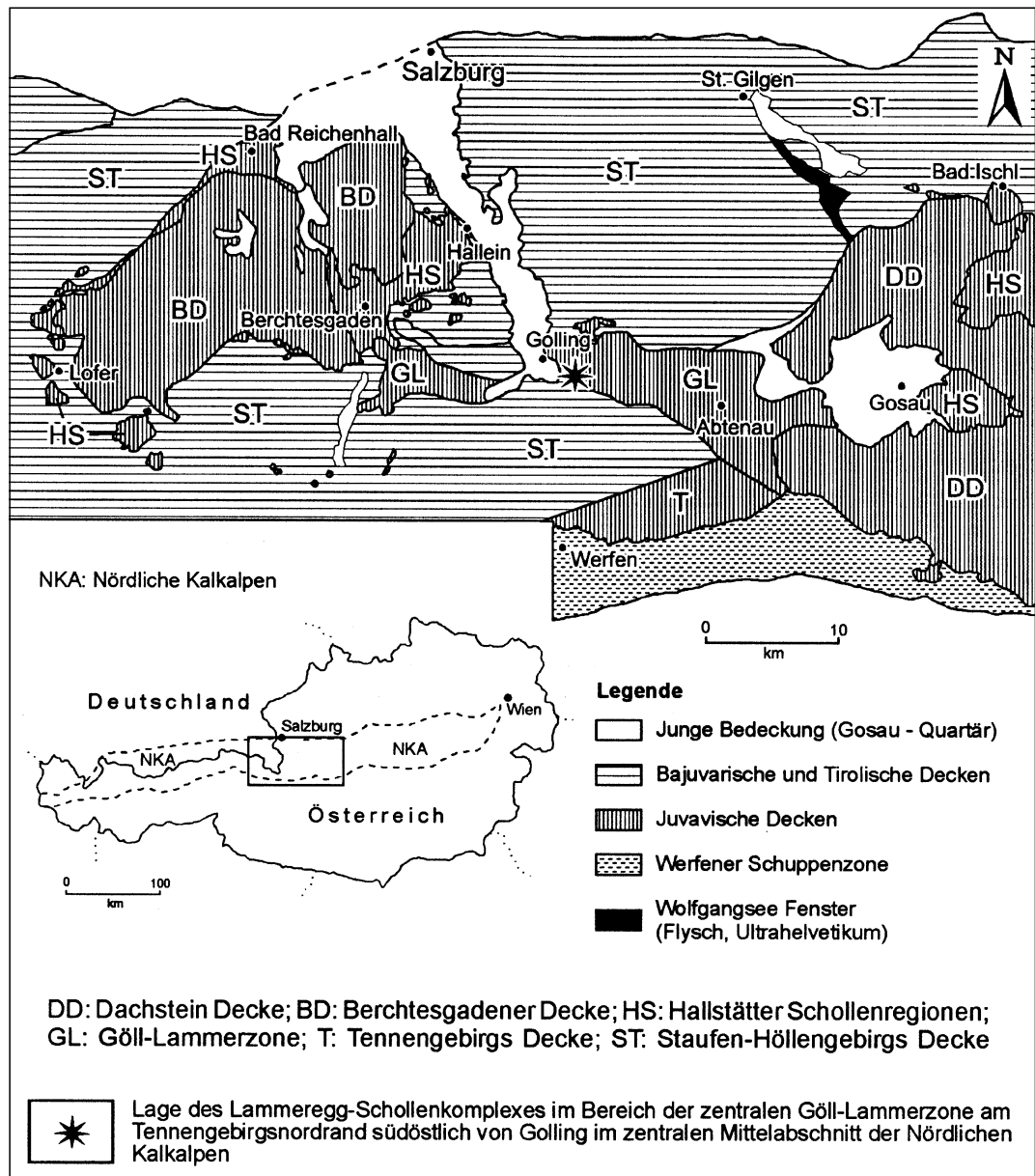
Abb. 1. Geologische und geographische Übersichtskarte des zentralen Mittelabschnittes der Nördlichen Kalkalpen und Lage des Lammeregg-Schollenkomplexes (verändert nach TOLLMANN, 1985 und GAWLICK et al., 1994).
