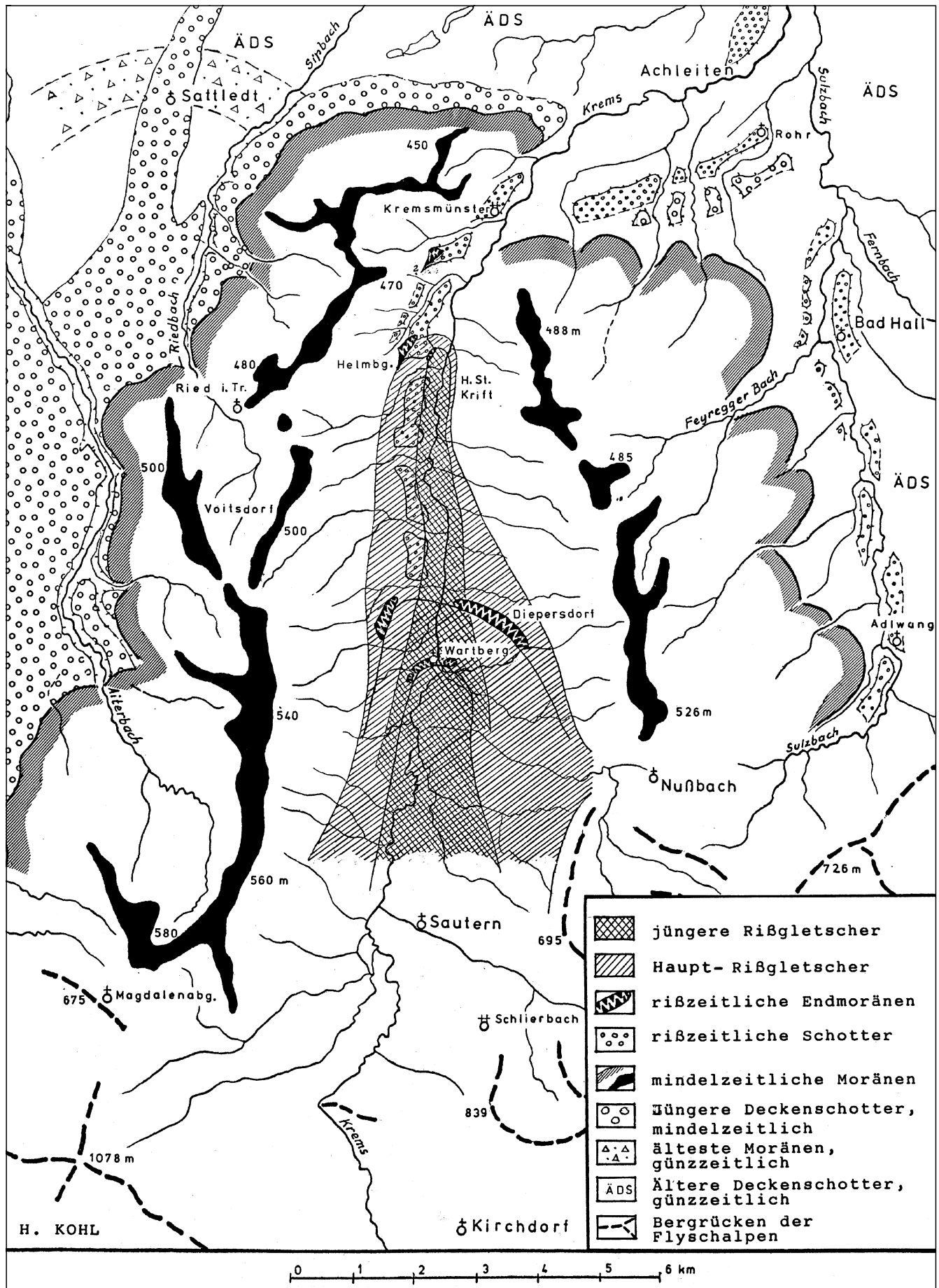
Abb. 7. Die mindel- und rißeiszeitlichen Gletscherbecken des Kremstales.
