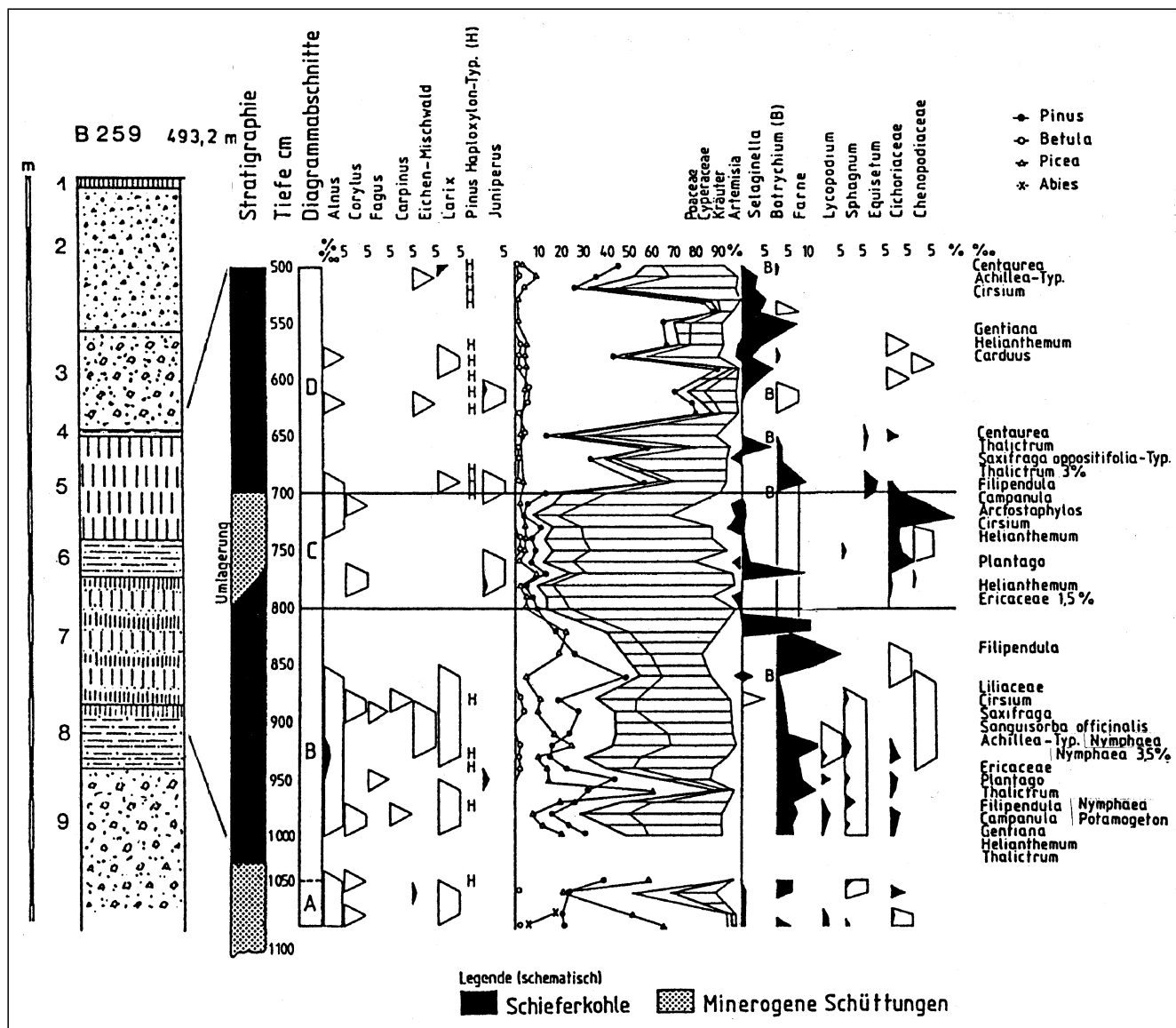
Abb. 10. Pollenprofil zwischen zwei Grundmoränen an der Wasserscheide Steyr-Kremstal bei Schön. Interstadial von Schön (Analyse von R. SCHMIDT aus H. KOHL & R. SCHMIDT, 1985).
