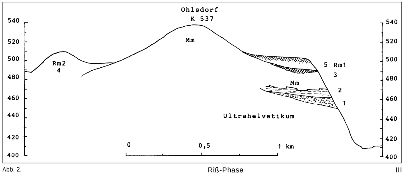
Abb. 2. Querschnitt durch die Moränenfolge im Raum Ohlsdorf N Gmunden.
