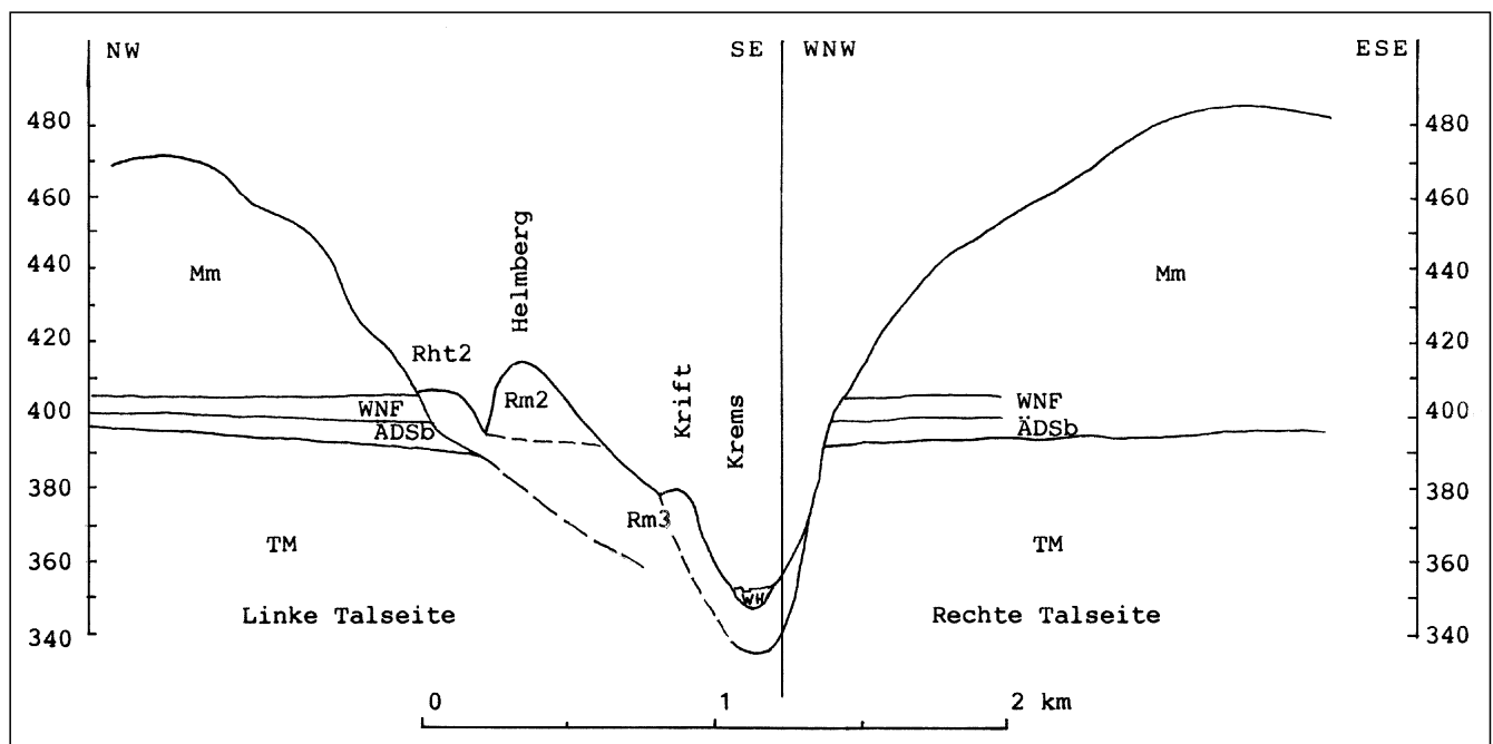
Abb. 8. Querschnitt durch das ö. Kremstal bei Helmberg-Krift, 2,75 km südlich Kremsmünster.
