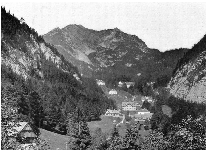
Abb. 3. Hallstätter Salzberg und Plassen vom Rudolfsturm. Aufnahme: E. KITTEL.
