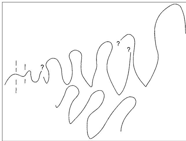
Abb. 5. Lobenlinie von Metapronorites ? sp. GEOLBA 2005/1/8, Waidegger Alm, Unter-Kasimovium, x 3,7.
