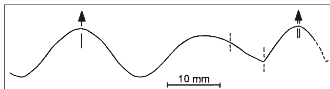
Abb. 2. Lobenlinie von Megaglossoceras schoenlaubi n. sp. Holotyp, GEOLBA 2005/1/4. Waidegger Alm, Unter-Kasimovium.
