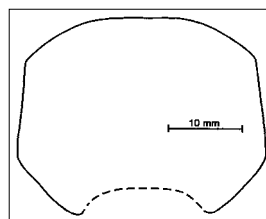
Abb. 3. Querschnitt von Megaglossoceras schoenlaubi n. sp. Holotyp, GEOLBA 2005/1/4. Waidegger Alm, Unter-Kasimovium.
