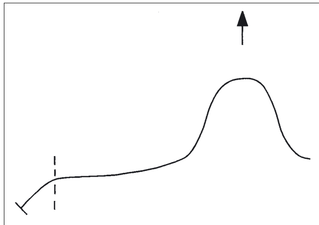
Abb. 4. Lobenlinie von Megaglossoceras sp. GEOLBA 2005/1/6 und 7, Waidegger Alm, Unter-Kasimovium, x 1,3.
