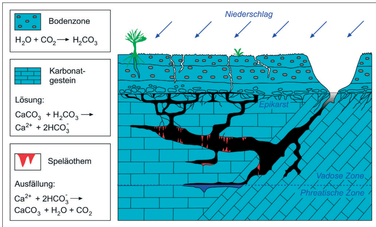
Abb. 1. Einfaches Modell der Bildung von Speläothemen in verkarsteten Karbonatgesteinen. Entwurf: I.J. FAIRCHILD
