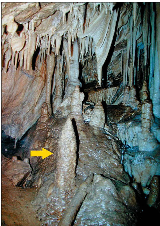
Abb. 39. Stark versinterter Teil der „Säulenhalle“ im Rassel-Bumslucke-O2J-System (Obirhöhlen). Eine U/Th-Datierung an einem Bohrkern an der Basis des Stalagmits im Vordergrund (gelber Pfeil) ergab ein Alter von ca. 300 kyr, d.h. dieser Stalagmit dürfte aus dem MIS 9 stammen. Foto: C. SPÖTL.
