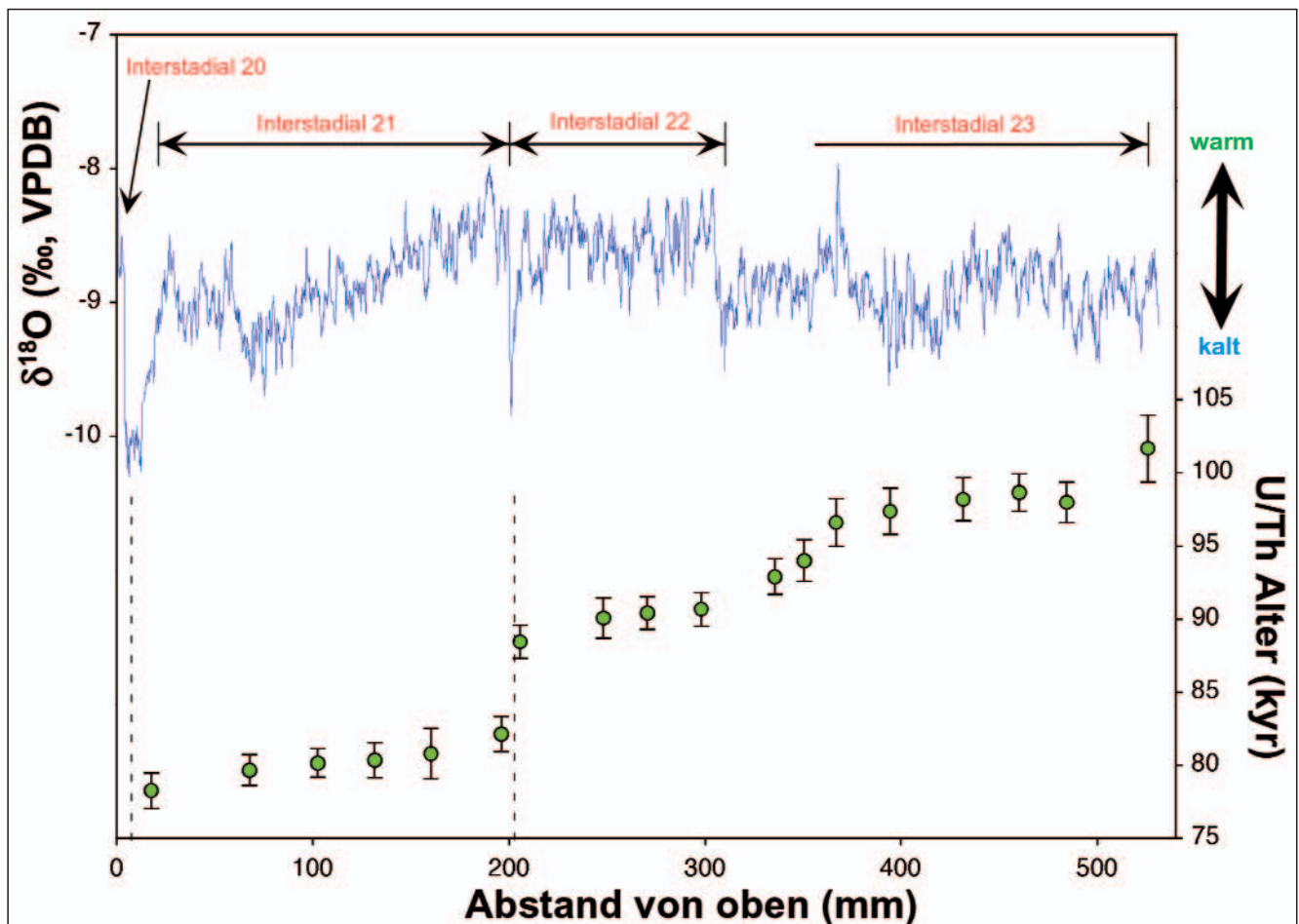
Abb. 35. Beispiel für einen detailliert untersuchten Stalagmiten aus der Gassel-Tropfsteinhöhle. Unten die hochaufgelöste U/Th-Chronologie (grün, mit 2- \sigma -Fehlerbalken) und oben die ca. 2100 Einzelmessungen umfassende O-Isotopenkurve (OFFENBECHER, 2004 und unveröff. Daten). Der Stalagmit besitzt zwei Wachstumsunterbrechungen (strichlierte Linien). Die Zuordnung zu Interstadialen (Nummerierung entsprechend dem Grönland-Eis) geschieht anhand des Verlaufs der O-Isotope sowie der U/Th Daten.
