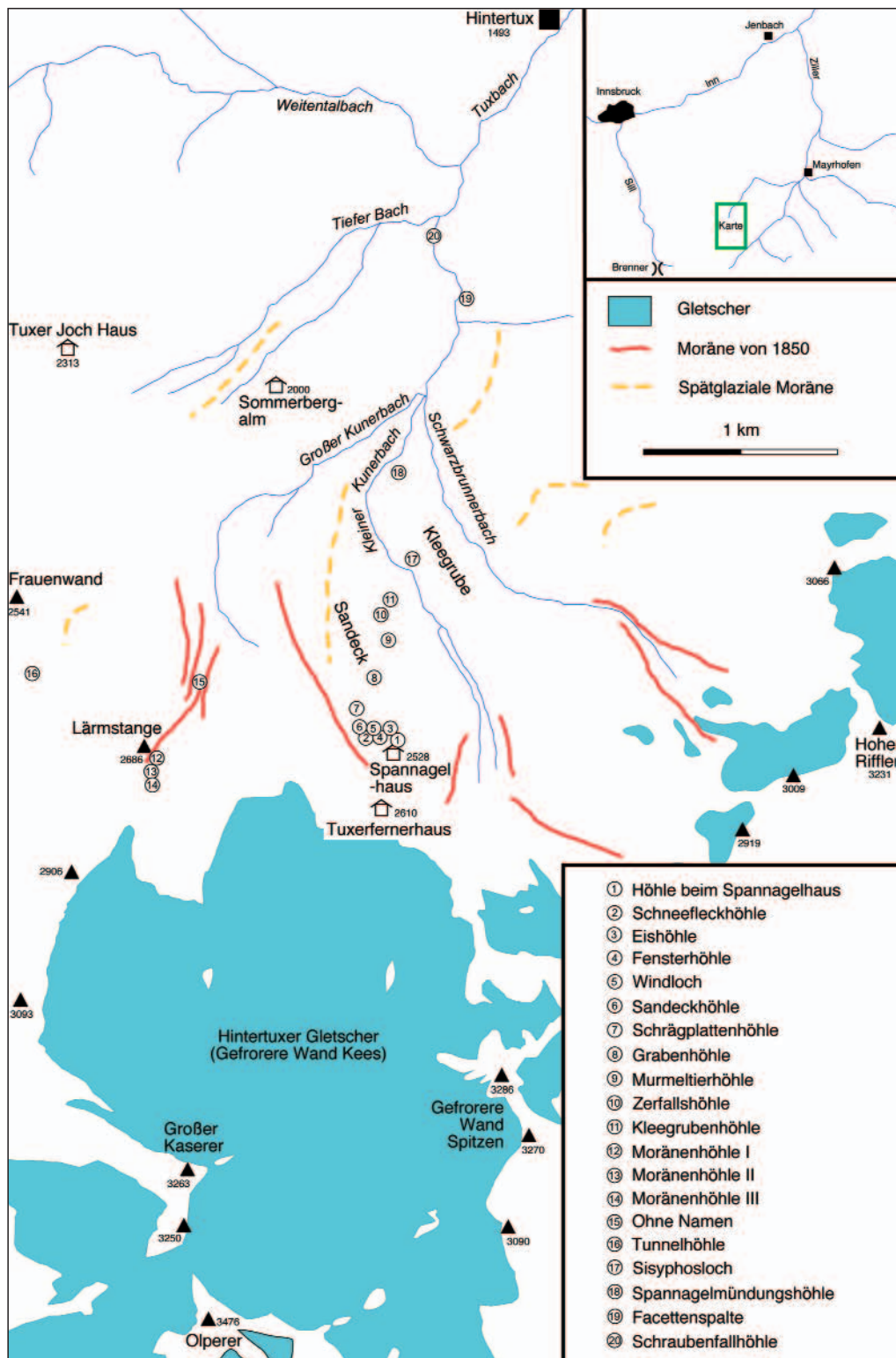
Abb. 23. Übersichtskarte des Talschlusses des Tuxer Tales mit Lage wichtiger Höhleneingänge, sowie Grenzen der heutigen Gletscherausdehnung (Stand von 1985), der Ausdehnung zum Hochstand am Ende der „Kleinen Eiszeit“ und ein reliktilsch erhaltener spätglazialer Stand.
