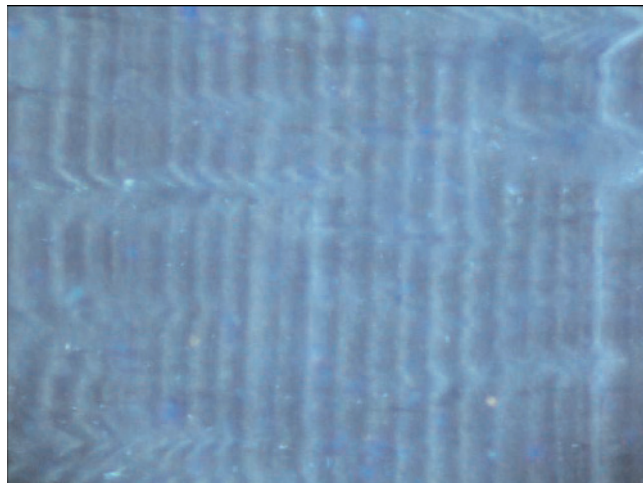
Abb. 22. Jährliche Wachstumsstruktur (Lamination) in einem Stalagmit der Wilder-Mann-Höhle (Aufnahme mit dem Epifluoreszenz-Mikroskop). Herbstliche Niederschläge reicherten vermutlich das Karstwasser mit jenen organischen Substanzen an, die die helle Fluoreszenz der Laminæ verursachen. Bildbreite 0,9 mm. Top ist links. Foto: M. MEYER.
