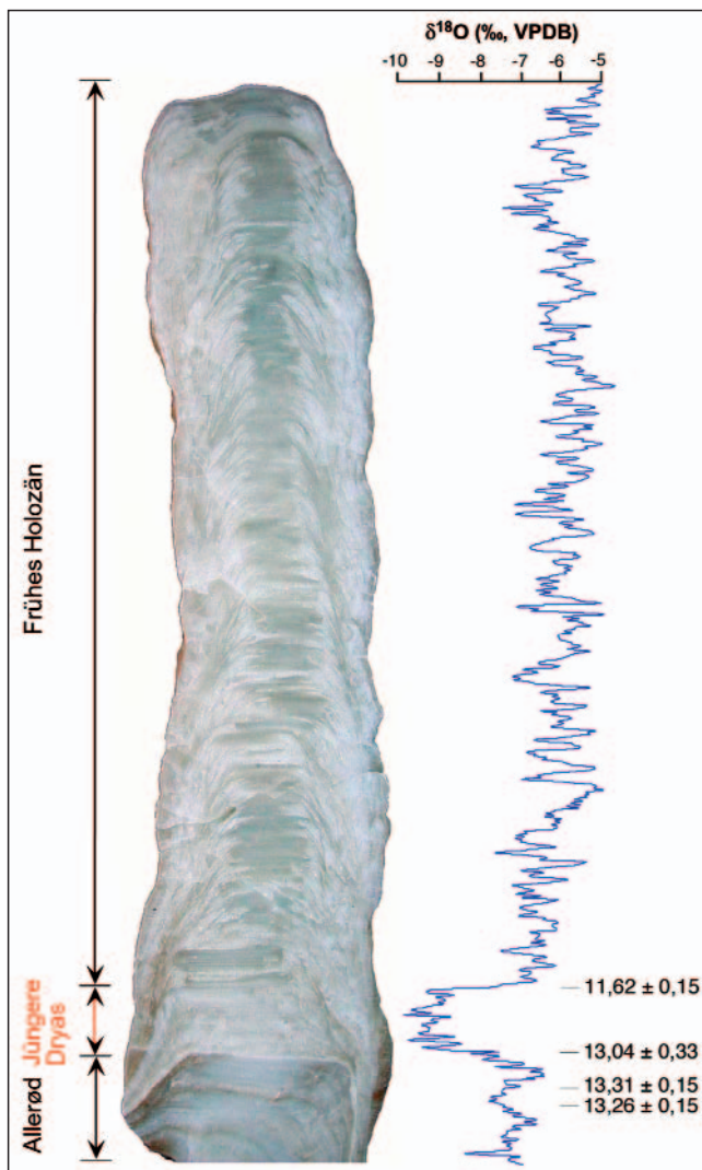
Abb. 44. Ein 36 cm hoher Stalagmit aus dem Blasloch begann sein Wachstum vor ca. 13 kyr (im Allerød) und seine O-Isotopenzusammensetzung spiegelt die markante Abkühlung während der Jüngeren Dryas deutlich wider (Altersangaben in kyr, mit 2-σ-Messfehlern). Während des frühen Holozäns wuchs der Hauptteil des Stalagmiten bei deutlich höheren Wachstumsraten.
