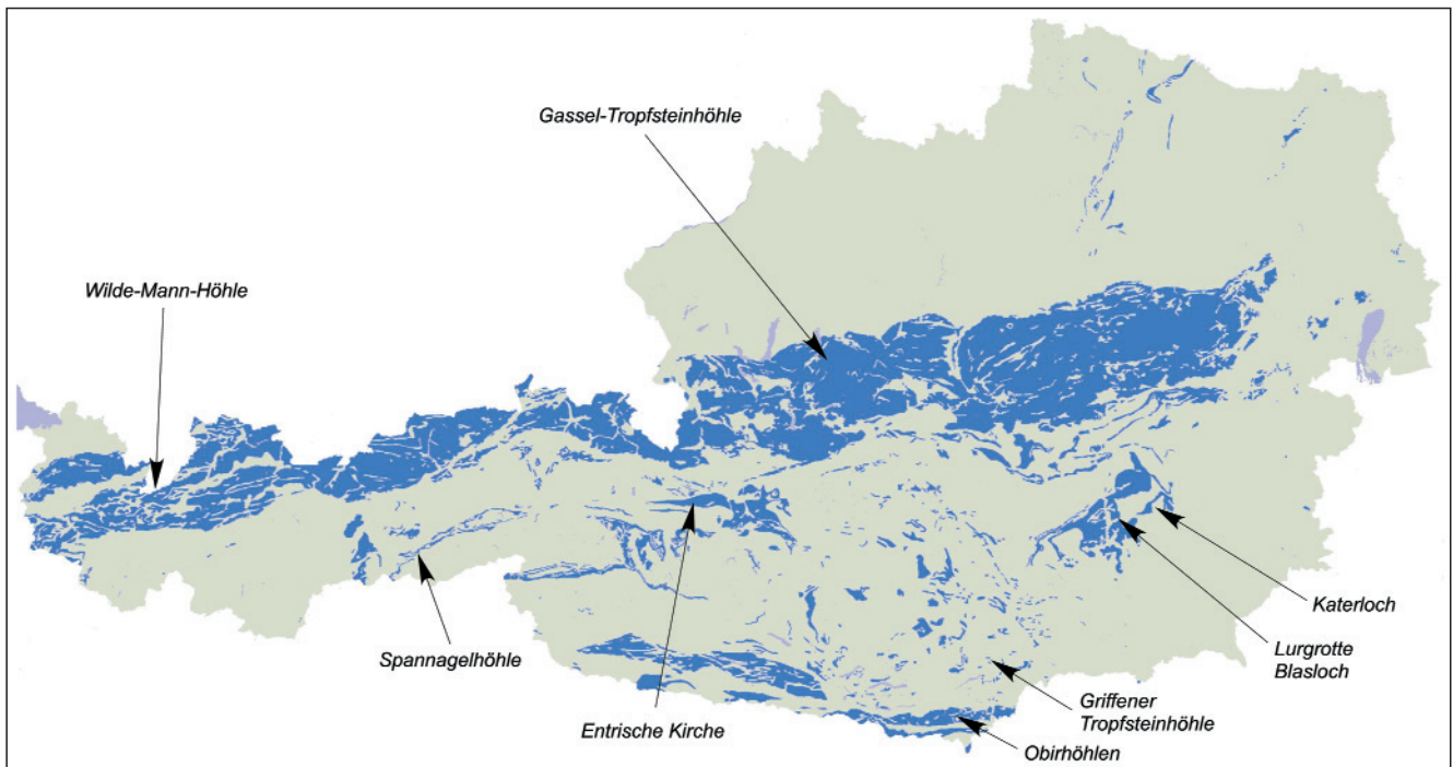
Abb. 19. Lage der Hauptuntersuchungsgebiete in Österreich. Grundlage: Verbreitung (verkarstungsfähiger) Karbonatgesteine (in Blau). Graphik: G. SCHUBERT, Geologische Bundesanstalt.
