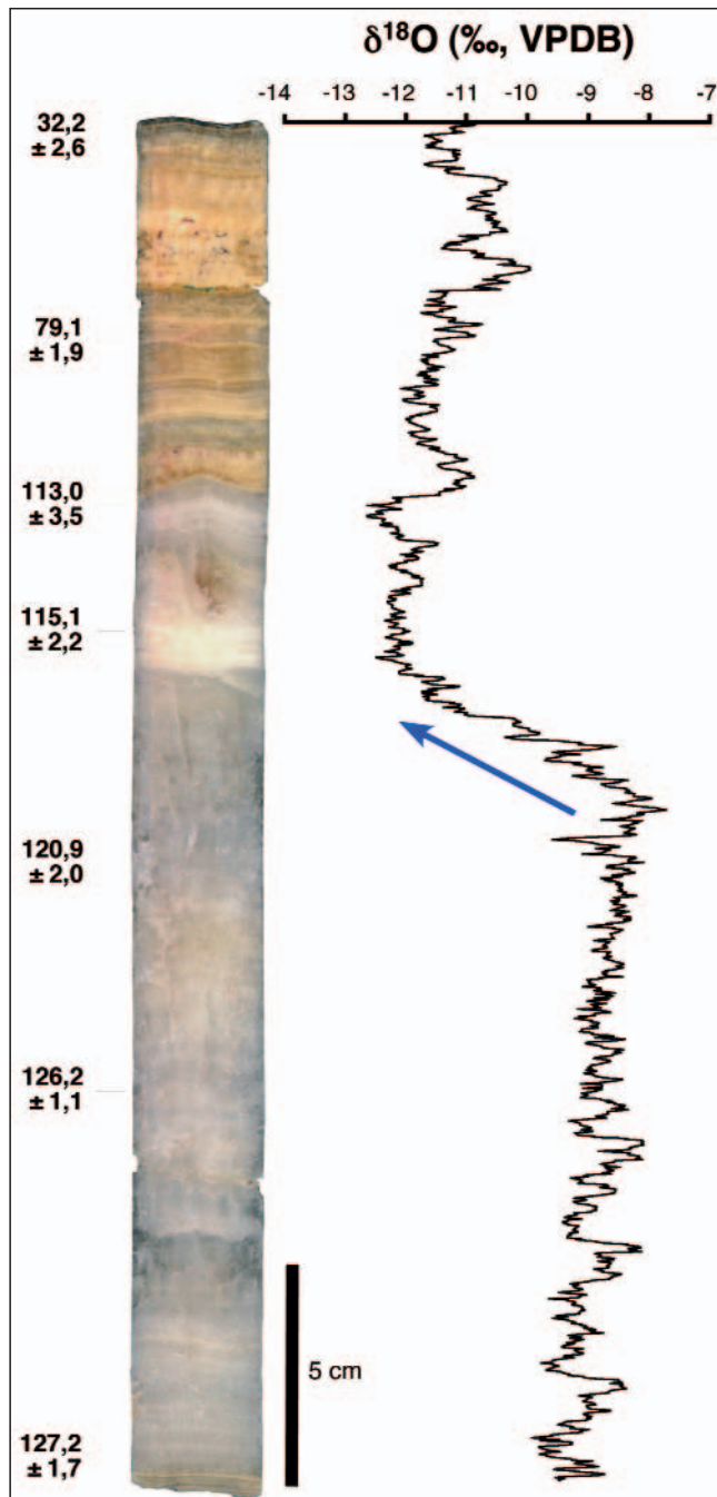
Abb. 32. Der obere Abschnitt eines Bohrkerns, entnommen aus dem Wandsinter am Fuß des „Teufelskrallenschlotes“ in der Entrischen Kirche (Top ist oben) und dessen U/Th-Alterswerte (links in kyr, mit 2σ-Fehlern) sowie die O-Isotopenwerte. Der eemzeitliche Kalzit ist weiß, porös und weist relativ hohe Isotopenwerte (–9.5 bis –7.5 ‰) auf. Das Ende des letzten Interglazials wird durch einen markanten Abstieg in den δ¹⁸O-Werten um 4 ‰ gekennzeichnet (Pfeil) und spiegelt eine massive Abkühlung wider. Der wärmzeitliche Kalzit (die obersten 70 mm des Bohrkerns) ist braun und detritusreich und stand unter dem Einfluss von glazialen und periglazialen Prozessen, welche im Einzugsgebiet dieser Höhle (ca. 2000 m Seehöhe) feinkörnigen Detritus in das Karstsystem infiltrierten.
