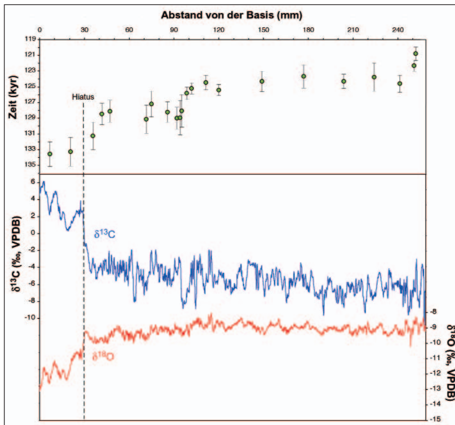
Abb. 27. Stalagmit aus der Spannagelhöhle, Bereich hinter dem „Nadelöhr“, der den Beginn der letzten Warmzeit (MIS 5.5) aufzeichnet. Die O-Isotopenwerte steigen ca. 3 cm über der Stalagmitbasis – unterbrochen durch einen Hiatus – zu hohen Werten an, die warme Lufttemperaturen indizieren. Parallel dazu nimmt der Anteil an ^{12}\text{C} , das präferentiell durch Bodenbildung (Vegetation) ins Grundwasser gelangt, stark zu (d.h. der \delta^{13}\text{C} -Wert sinkt). Im oberen Teil des Diagramms sind die einzelnen U/Th Messwerte geplottet (grün, inklusive 2- \sigma -Messfehler; HOLZKÄMPER et al., 2004, 2005).
