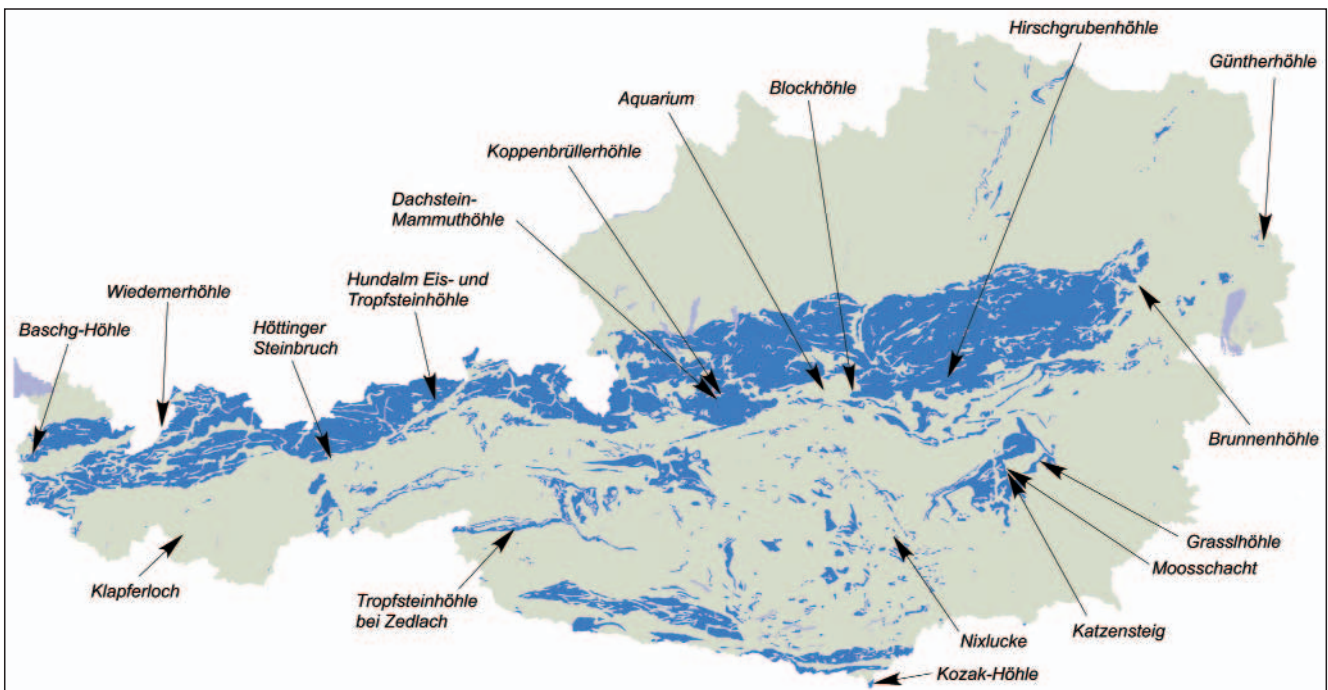
Abb. 48. Lage weiterer untersuchter Höhlen in Österreich. Grundlage: Verbreitung (verkarstungsfähiger) Karbonatgesteine (in Blau). Graphik: G. SCHUBERT (Geologische Bundesanstalt).
