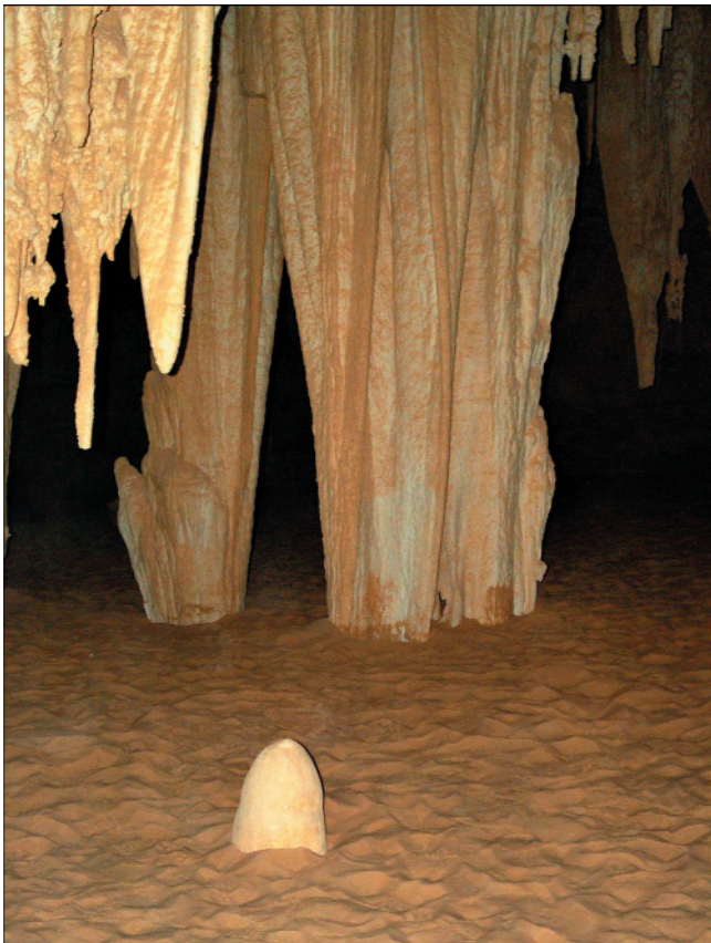
Abb. 5. Die fossilen Speläotheme der Djara-Höhle, die von hereingeblasenem Wüstensand begraben werden, zeugen von einst wesentlich feuchterem Klima des heute hyperariden Gebietes (4 mm Niederschlag pro Jahr) der ägyptischen Wüste zwischen der Fara Depression und dem Niltal. Altersbestimmungen dieser bis zu 6 m hohen und 2 m mächtigen Stalagmite und Stalaktite haben großteils Werte jenseits von ca. 400–500 kyr ergeben; spätere Feuchtphasen sind durch Sinteralter des MIS 9, 7 und 5 indiziert (BROOK et al., 2003; HOLZKÄMPER, 2004). Foto: A. MANGINI.
