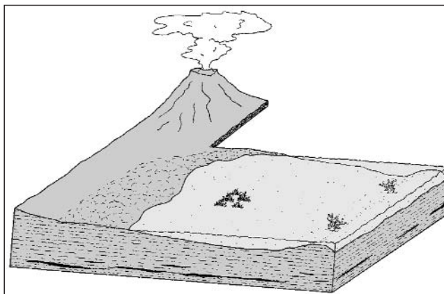
Abb. 5. Schematische Darstellung der Ablagerungsbedingungen der Flösserkogel-Formation.
