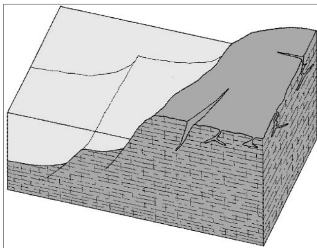
Abb. 10. Schematische Darstellung der Ablagerungsbedingungen der Sanzenkogel-Formation.
