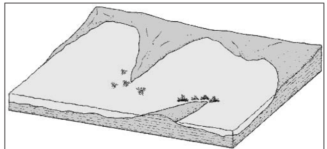
Abb. 7. Schematische Darstellung der Ablagerungsbedingungen der Mitteldevondolomite der Gaisbergsattel-Subformation.
