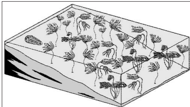
Abb. 4. Schematische Darstellung der Ablagerungsbedingungen der Parmasegg-Formation.
