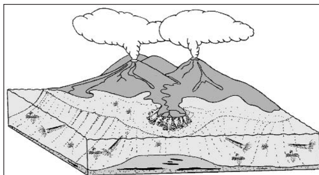
Abb. 3. Schematische Darstellung der Ablagerungsbedingungen der Kehr-Formation.
