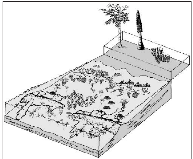
Abb. 6. Schematische Darstellung der Ablagerungsbedingungen der Plabutsch-Formation.
