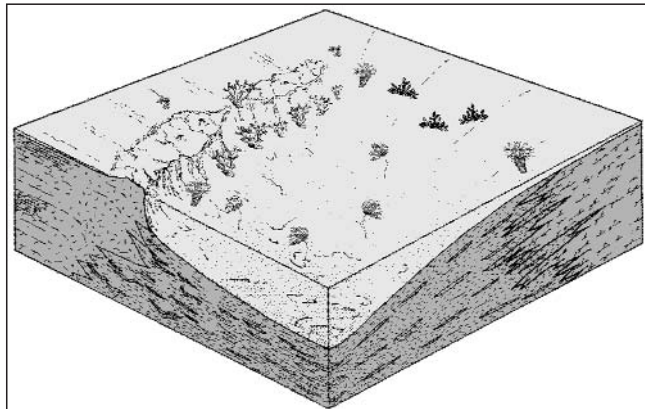
Abb. 8. Schematische Darstellung der Ablagerungsbedingungen der Kollerkogel-Formation.
