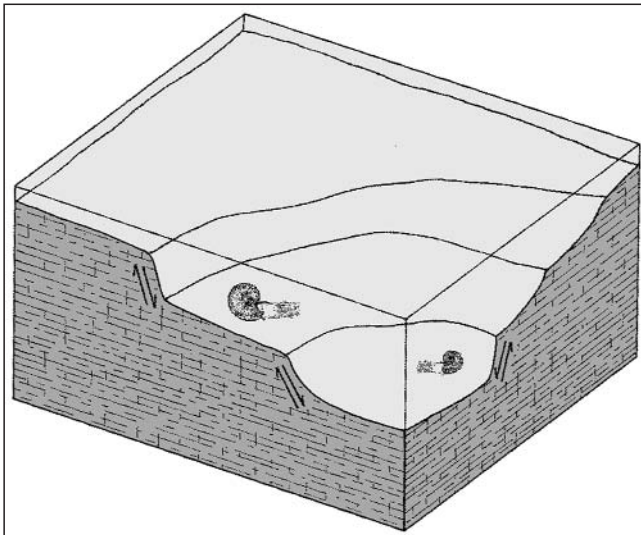
Abb. 9. Schematische Darstellung der Ablagerungsbedingungen der Steinberg-Formation.
