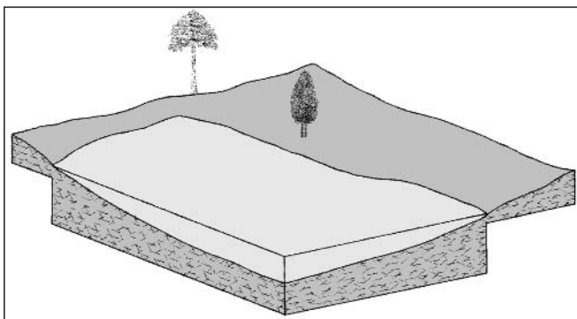
Abb. 11. Schematische Darstellung der Ablagerungsbedingungen der Hahngraben-Formation.
