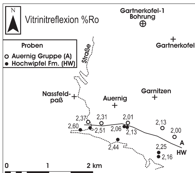
Abb. 1. Regionale Verteilung der Vitritreflexionswerte entlang des Kontaktes zwischen der Hochwipfel-Formation und der Auernig-Gruppe am Südhang des Auernig-Gipfels.
