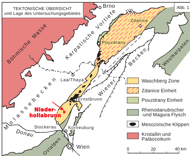
Abb. 1. Tektonische Übersichtsskizze und geographische Lage von Niederhollabrunn.
