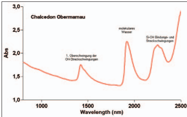
Abb. 4. Nahes-Infrarot-Spektrum des Chalcedons von Obermamau. Die Absorptionsbanden bei 2222 nm entsprechen Bindungs- und Streckschwingungen von Silanol-Gruppen. Die Bande bei 1923 nm wird durch molekulares H 2 O verursacht und die Bande bei ca. 1429 nm ist die 1. Oberschwingung der Hydroxyl-Streckschwingungen sowohl des molekularen als auch des an Silanol gebundenen Wassers. Absorptionmessung, Cary 500, RT, Probendicke 0,5 cm.
