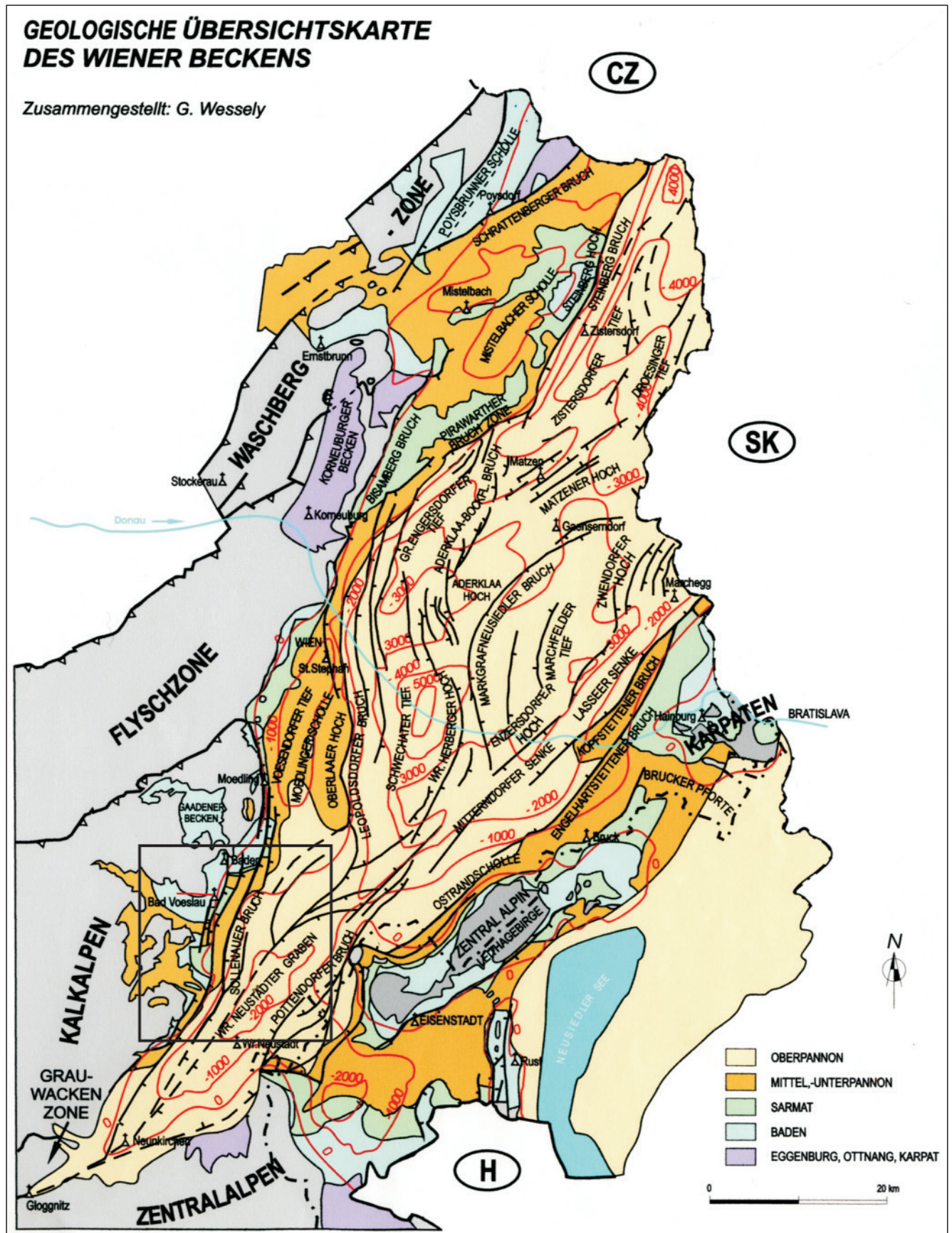
Abb. 1. Die Lage von Bad Vöslau am Westrand des Wiener Beckens.
