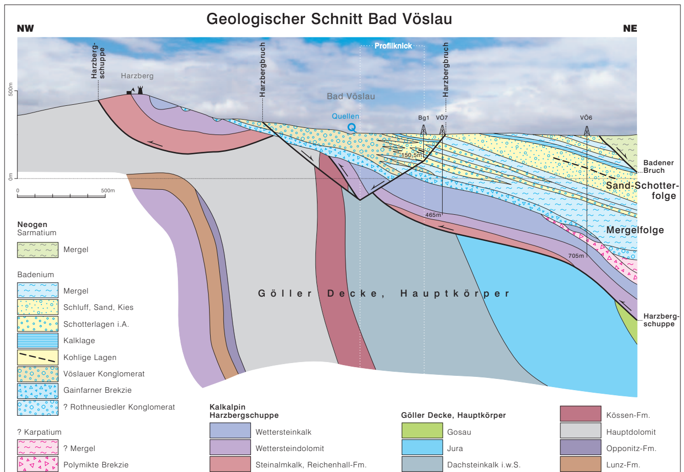
Abb. 3. Geologischer Schnitt durch Bad Vöslau.
