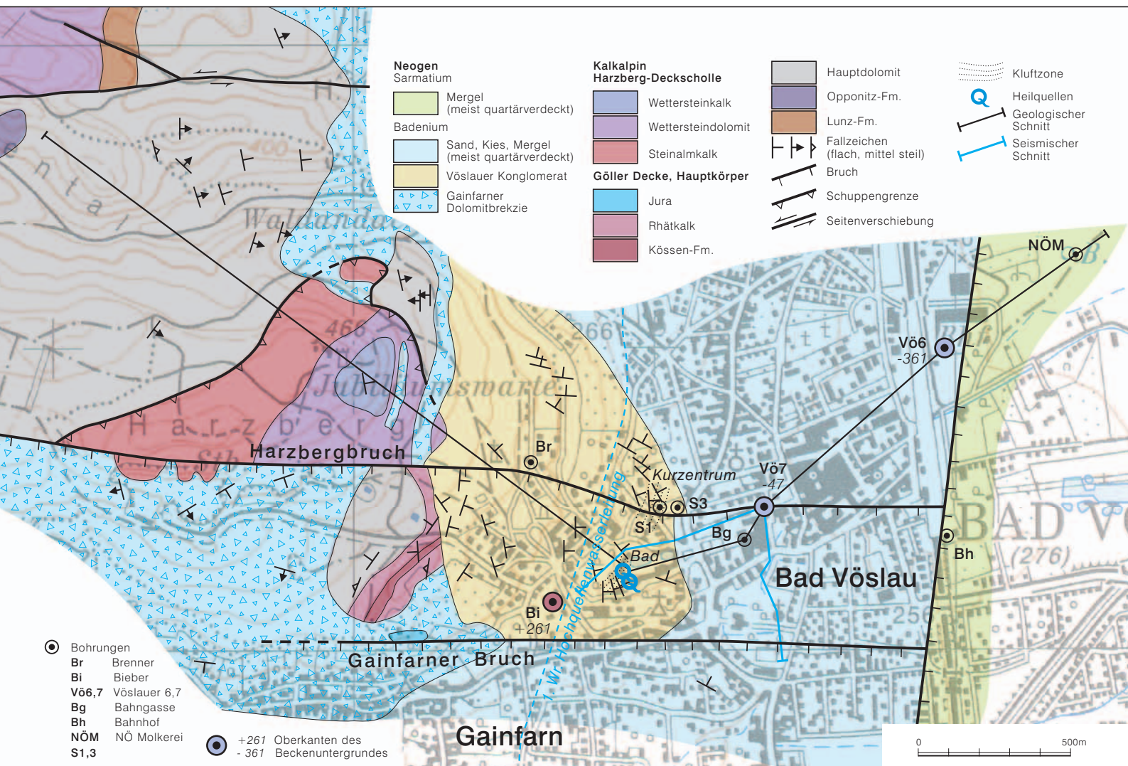
Abb. 2. Geologische Übersichtskarte von Bad Vöslau.
