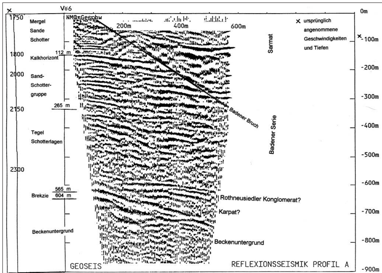
Abb. 16. Seismisches Profil von der Bohrung Vö6 ostwärts.
