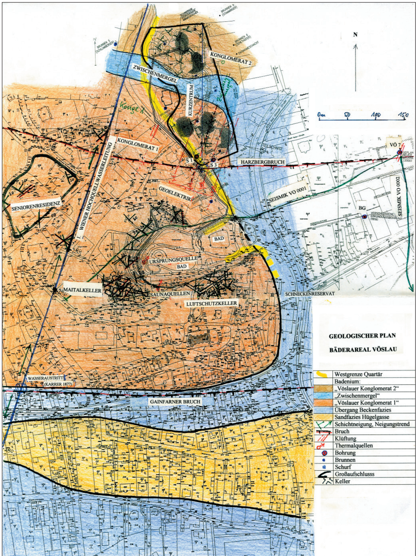
Abb. 6. Kartenskizze der Bäderareale.
