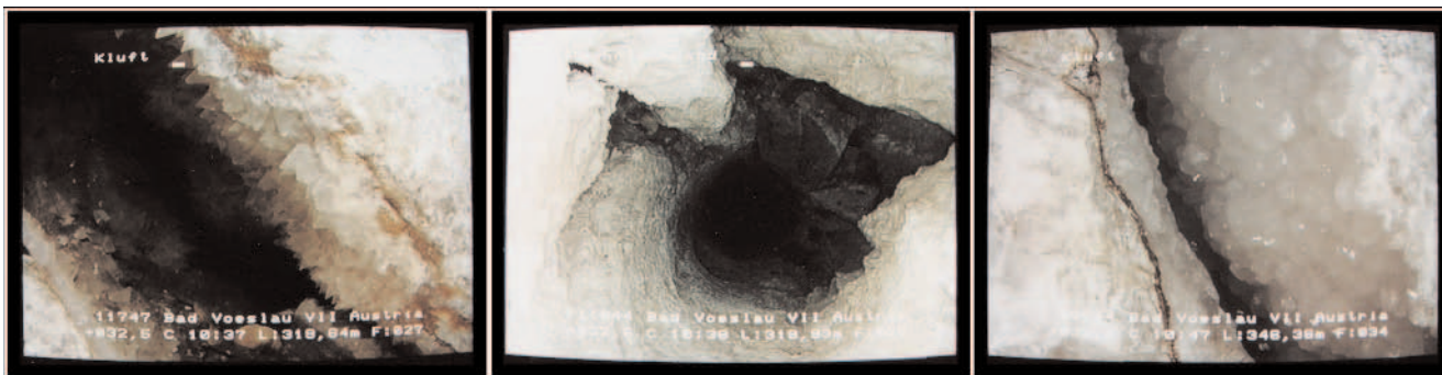
Abb. 15. Bohrung Vöslauer 7: Kalzitbesetzte Spalten als Zutrittsstellen des Thermalwassers.
