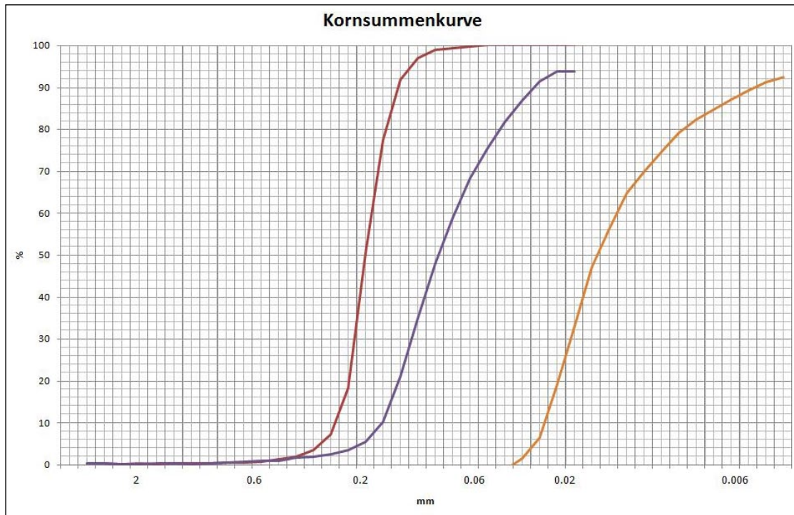
Abb. 9. Kornsummenkurven der Proben Sb 13 (Mittelsand, rot), Sb 16 (Feinsand, vio- lett) und SBT 1 (toni- ger Silt, orange).
