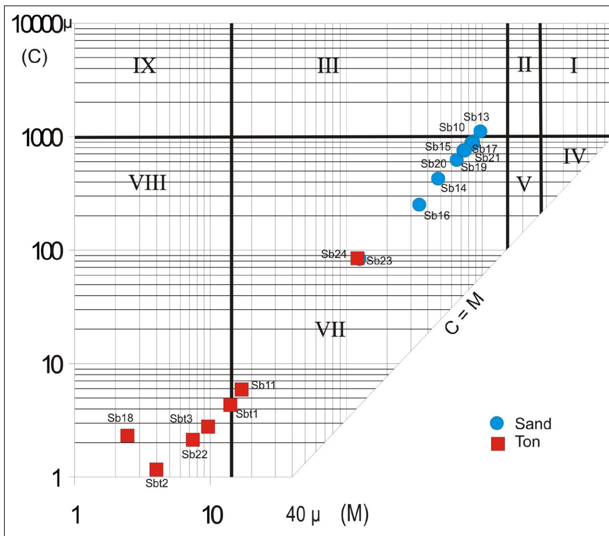
Abb. 10. Die untersuchten Proben der Sandgrube Steinbrunn im CM-Diagramm (nach PASSEGA & BYRAMJEE, 1969).
