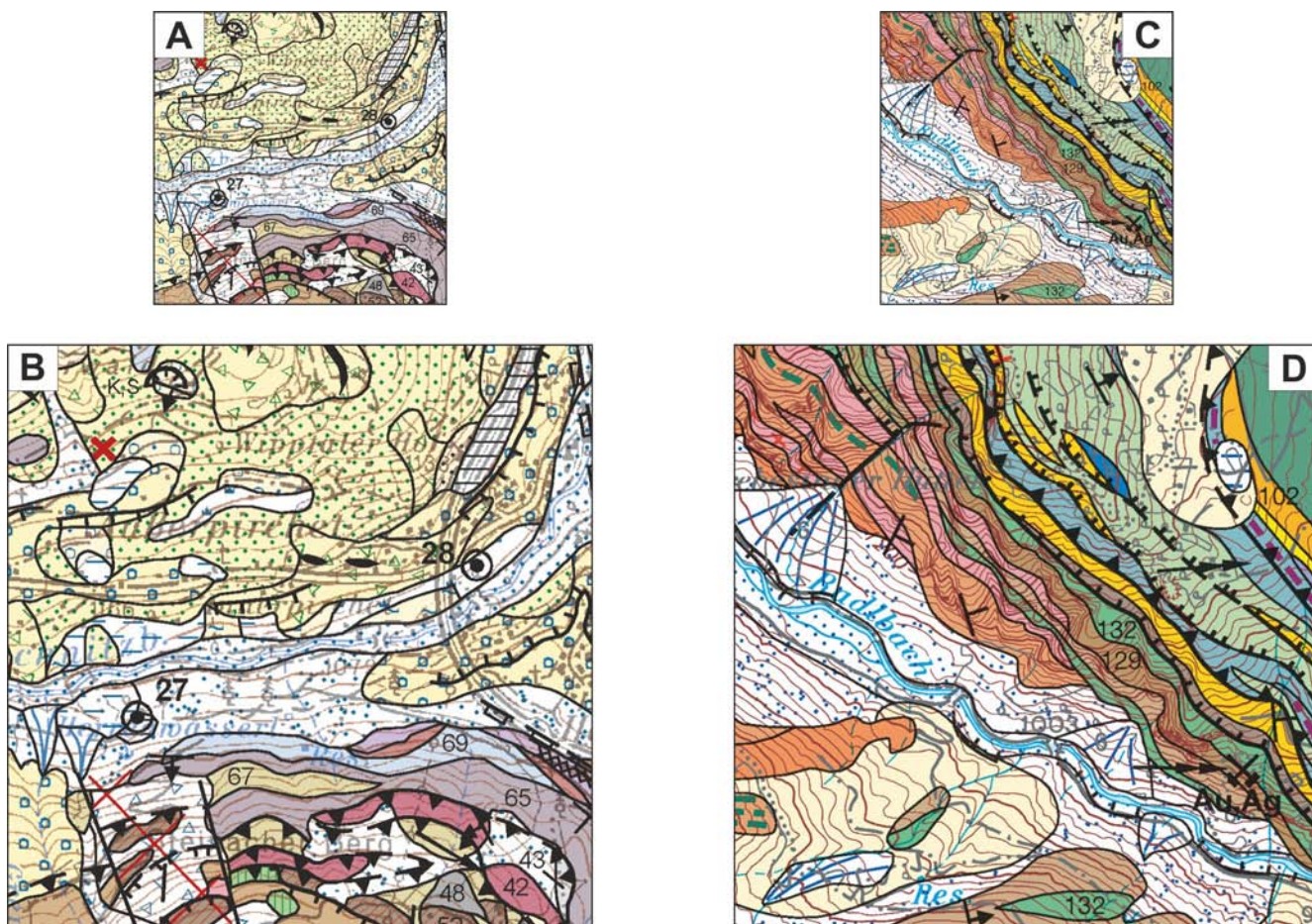
Abb. 4. Gegenüberstellung von Kartenausschnitten der GK 50 im Originalmaßstab 1:50.000 mit einer Vergrößerung dieser Ausschnitte im Maßstab 1:25.000, zwecks Demonstration der deutlich verbesserten Lesbarkeit der Karteninhalte im Maßstab 1:25.000. Die Liniendicke und das Symboldesign (z.B. der Decken- und Schuppengrenzen) wurden nicht für den Maßstab 1:25.000 angepasst, damit erklärt sich das etwas klobige Erscheinungsbild dieser grafischen Elemente in den vergrößerten Ausschnitten. Die Lesbarkeit einer „echten“ Karte 1:25.000 wäre also sogar noch besser, als hier dargestellt.
