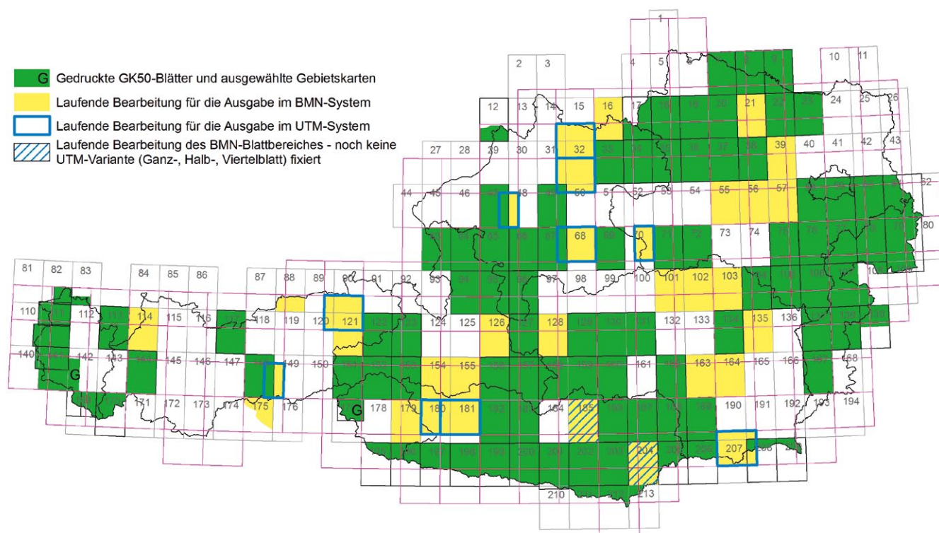
Abb. 5. Das Spezialkartenprogramm GK 50/25 der Geologischen Bundesanstalt im August 2010.
