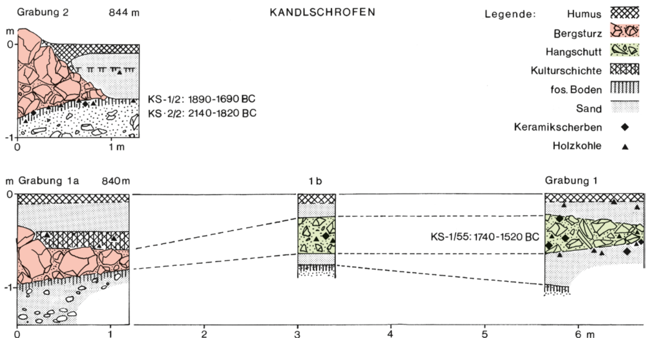
Abb. 6. Aufschlusskizze des Bergsturz-Brandungswalles am Kandlschrofen.
