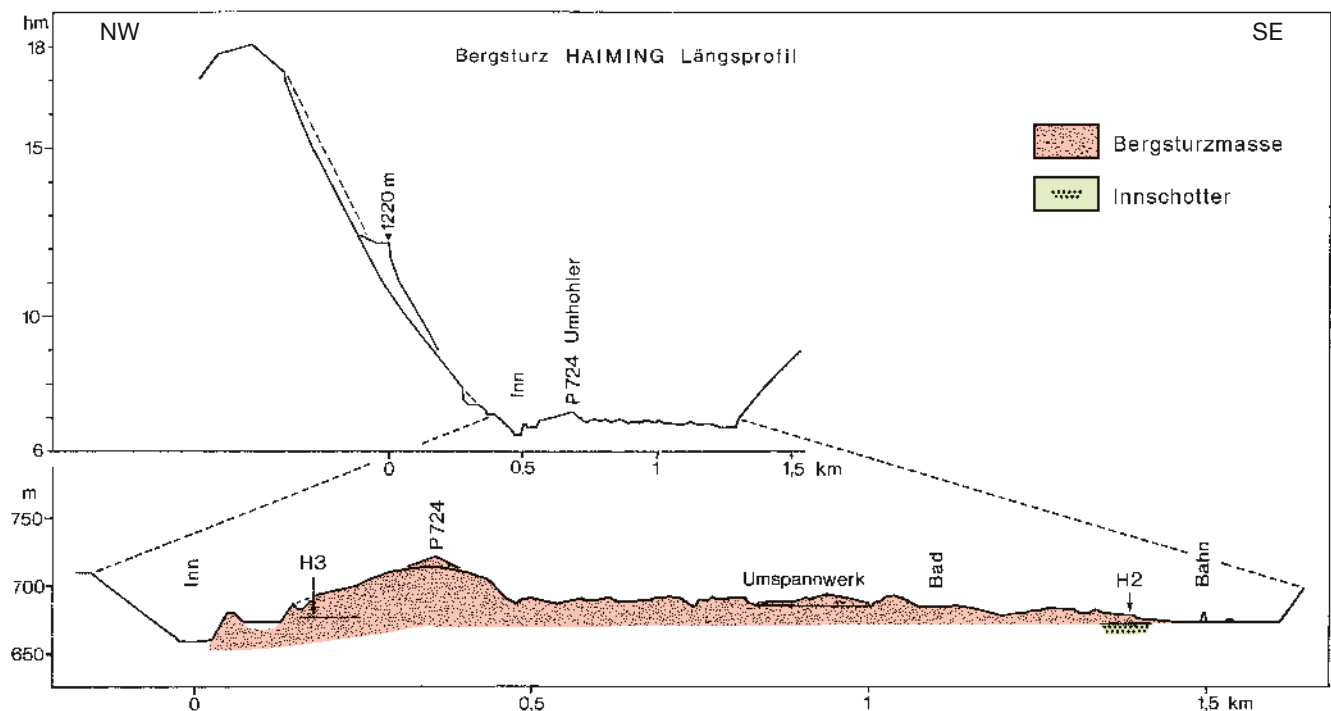
Abb. 8. Längsprofil des Bergsturzes von Haiming, 2,5-fach überhöht und vergrößerter Ausschnitt.
