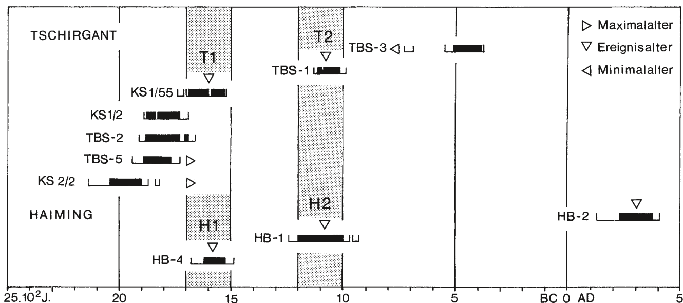
Abb. 14. Diagramm der Radiokarbonaten aus den Bergsturzgebieten vom Tschirgant und von Haiming.
