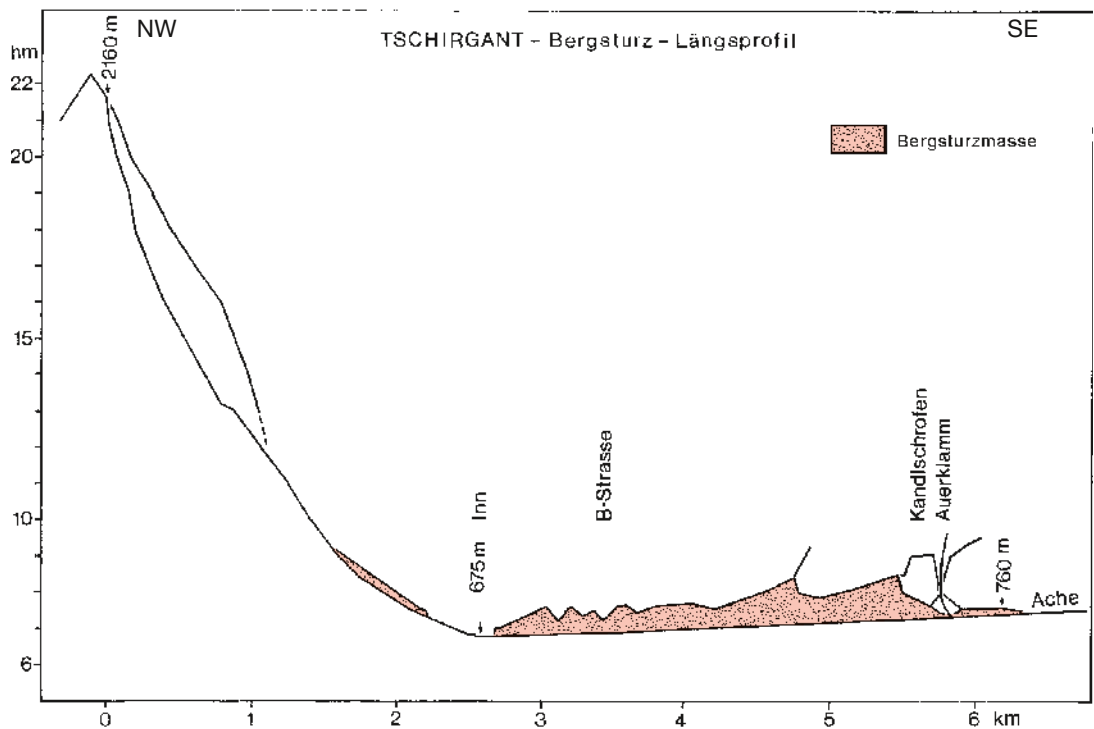
Abb. 2. Längsprofil des Bergsturzes vom Tschirgant, 2,5-fach überhöht.
