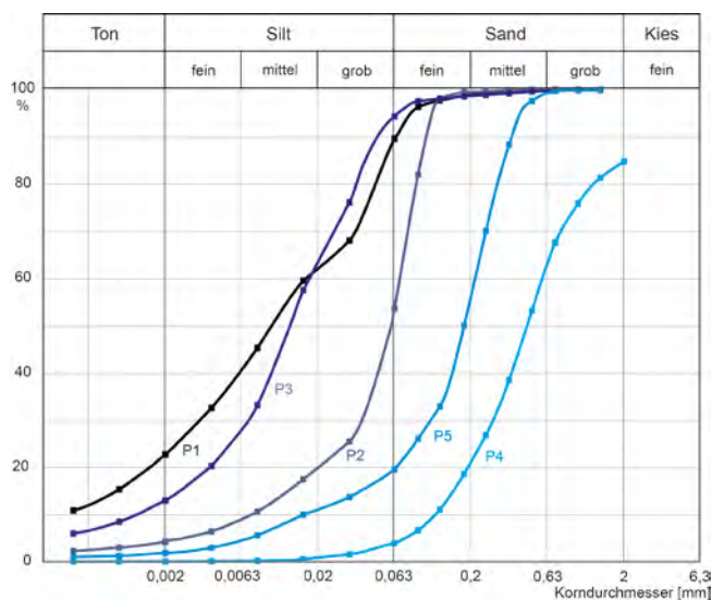
Abb. 4. Kornsummenkurven der im Typusprofil der Traisen-Formation entnommenen Proben. Die Sedimente sind als schlecht bis extrem schlecht sortierter tonig-sandiger Silt bis Sandsilt (P1–3), oder schlecht bis sehr schlecht sortierter siltyger Sand bis kiesiger Sand (P4, 5) zu benennen.
