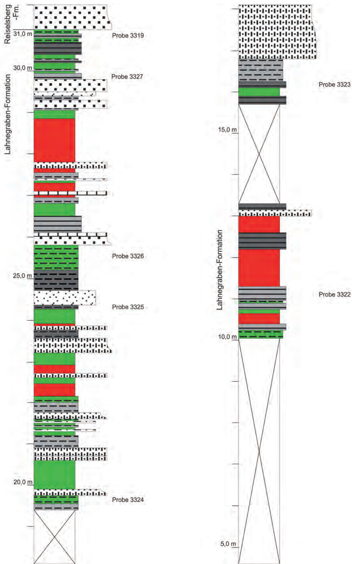
Abb. 4. Säulenprofil der Lahnegraben-Formation an der Typuslokalität.
