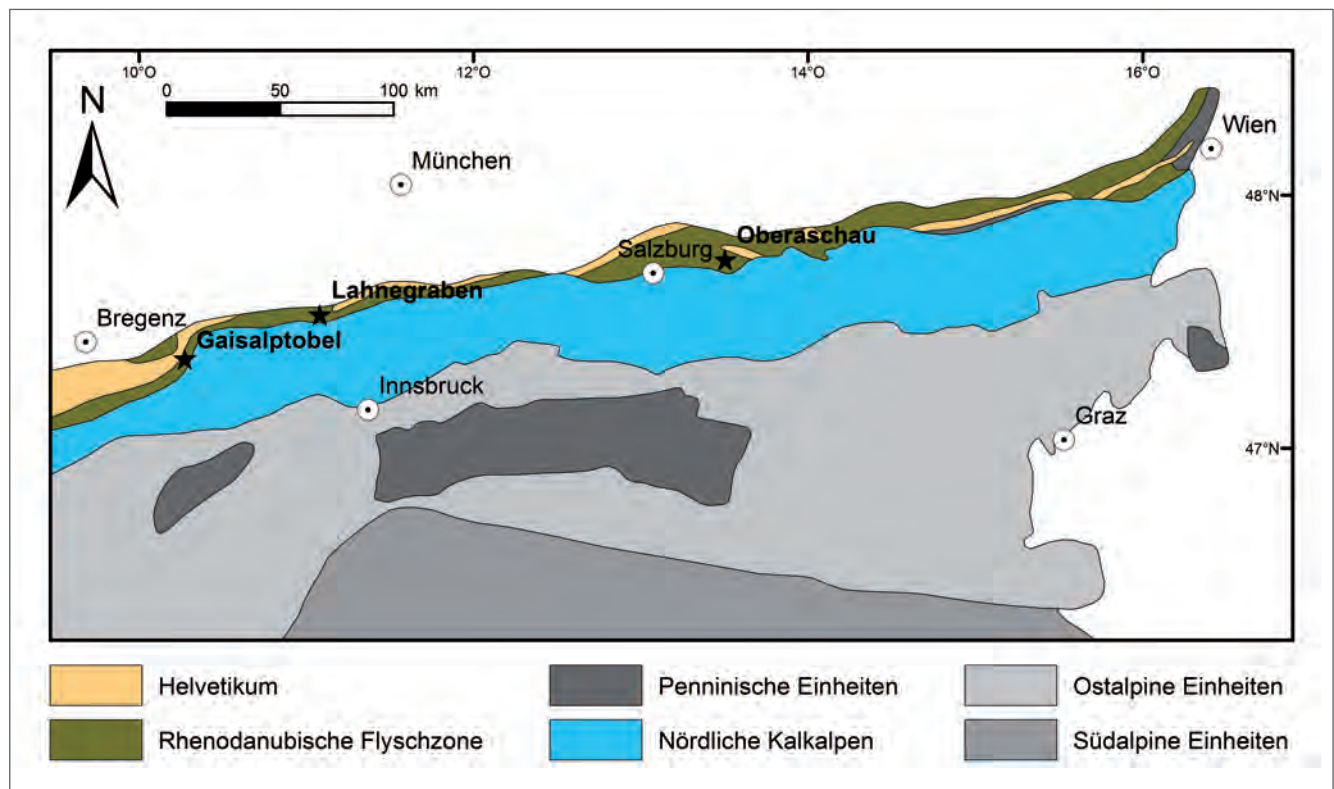
Abb. 1. Tektonische Übersichtskarte der Ostalpen mit Verbreitungsgebiet der Rhénodanubischen Flyschzone (vereinfacht nach FAUPL & WAGREICH, 2000). Ebenfalls dargestellt sind die im Text genannten Lokalitäten Lahnegraben, Gaisalptobel und Oberaschau.
