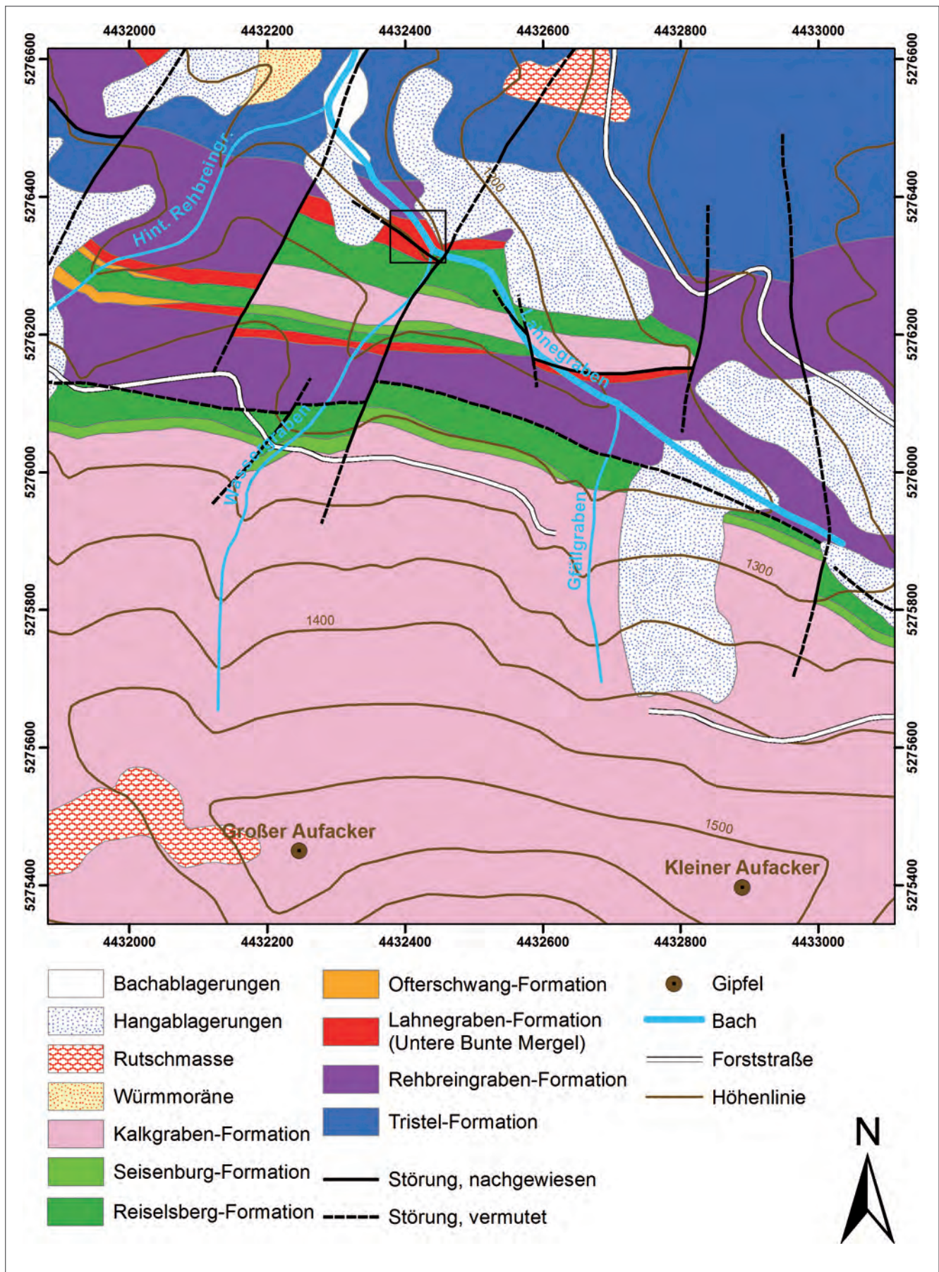
Abb. 3. Geologischer Rahmen des Typusprofils der Lahnegraben-Formation („Untere Bunte Mergel“) im oberen Lahnegraben, östlich Unterammergau/Oberbayern (Karten- rahmen mit Gauß-Krüger-Koordinaten; vereinfacht nach TEIPEL & HAHN, in Vorb.).
