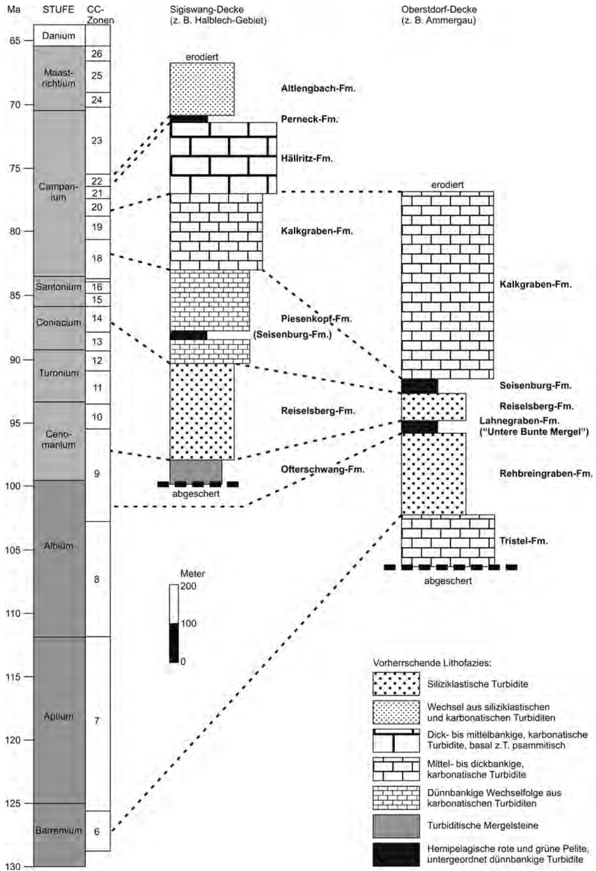
Abb. 2. Schemaprofil und Nannofossilien-Biostratigraphie der Greifenstein-Gruppe (Rhenodanubisches Deckensystem) (aus: EGGER & SCHWED (2008), unter Berücksichtigung von MATERN (1998) für die Oberstdorf-Decke, Chronostratigraphie nach GRADSTEIN et al. (2012)).
