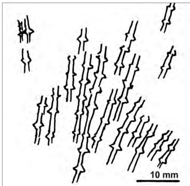
Abb. 2. Anordnung der dendroclonen Skleren in Spongiomorpha ramosa FRECH. Die Richtung der langen Achsen entsprechend der Wachstumsrichtung des Schwammes (gezeichnet aus Taf. 1/ Fig. 3).
