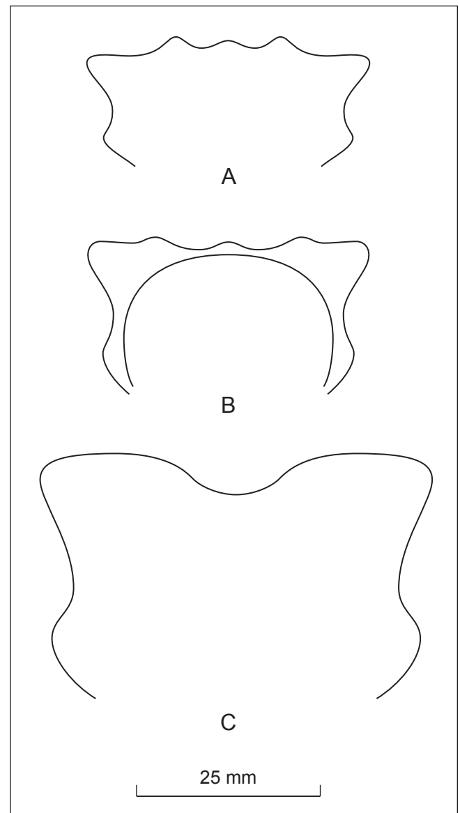
Text-Fig. 8. Cunninghamoniceras alatum (ZABORSKI, 1985). Whorl sections of A: GBA 2016/004/0038; B: GBA 2016/004/0070; C: GBA 2016/004/0071.
