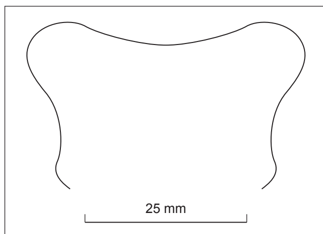
Text-Fig. 9. Cunningtoniceras alatum (ZABORSKI, 1985). Whorl section of GBA 2016/004/0072.
