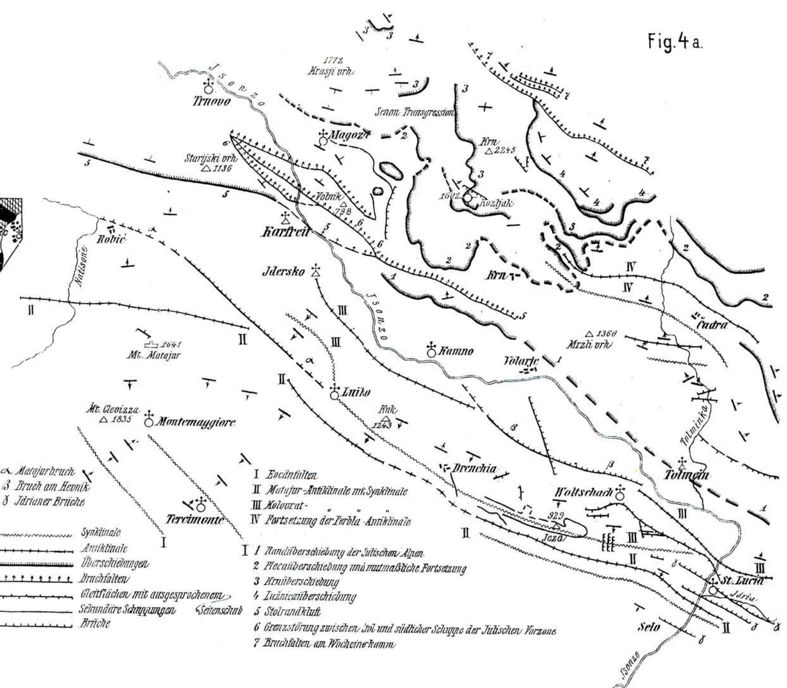
Geologische Skizze des Malajurgebietes Masstab 1:30.000. Aufgenommen im Jahre 1918.
