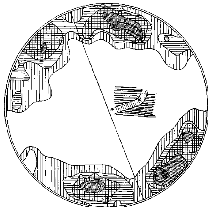
Abb. 29. Seefelder Kalzitgang, parallel s, 394 Pole der Zwillingslamellen.
