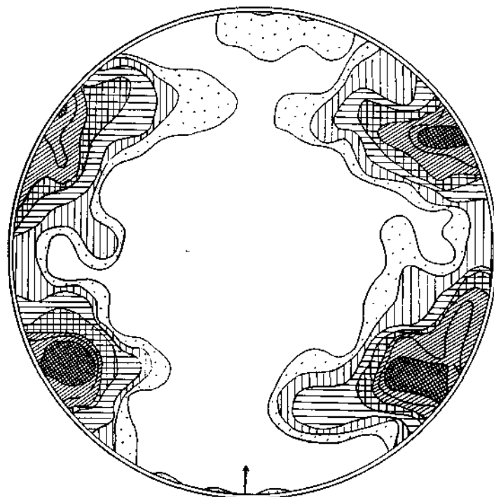
Abb. 12. Großoolith, Brunnstein, senkrecht s , 389 Kalzitlamellen. Musterung wie bei Abb. 9.
