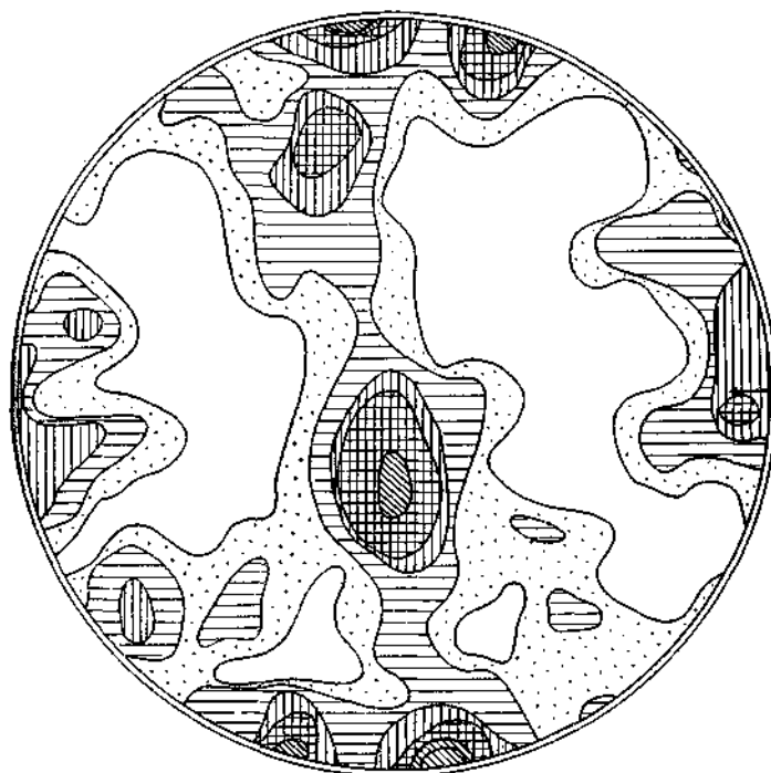
Abb. 35. Silurkalkgang, Paß Thurn, Quarze, 394 Achsenpole.
