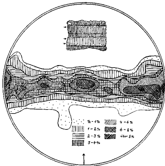
Abb. 9. Großoolith, Brunnenstein, senkrecht s, 435 Achsenpole.
