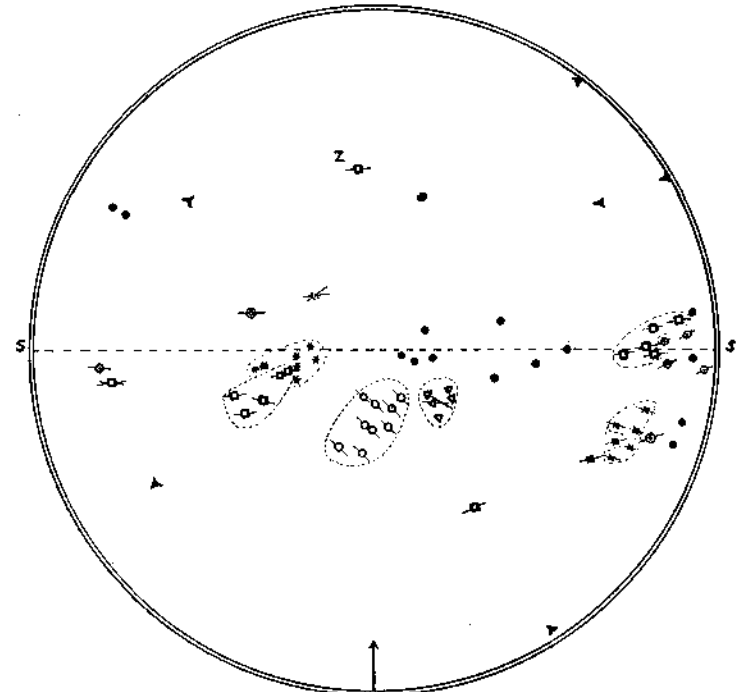
Abb. 48. Erzbergit, Achsenpole der sekundären Kalzite.
