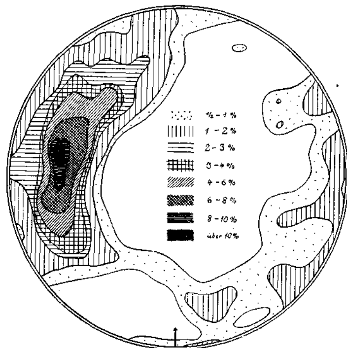
Abb. 27. Seefelder Kalzitrasen, senkrecht s Rand, 248 Pole der Zwillingslamellen. Musterung wie in Abb. 29.
