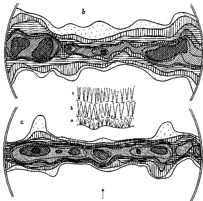
Abb. 11. Großoolith, Brunnstein, Lage b (1—3 mm von der Anwachsfläche, 230 Achsenpole) und Lage c (3—5 mm von der Anwachsfläche, 180 Achsenpole).
