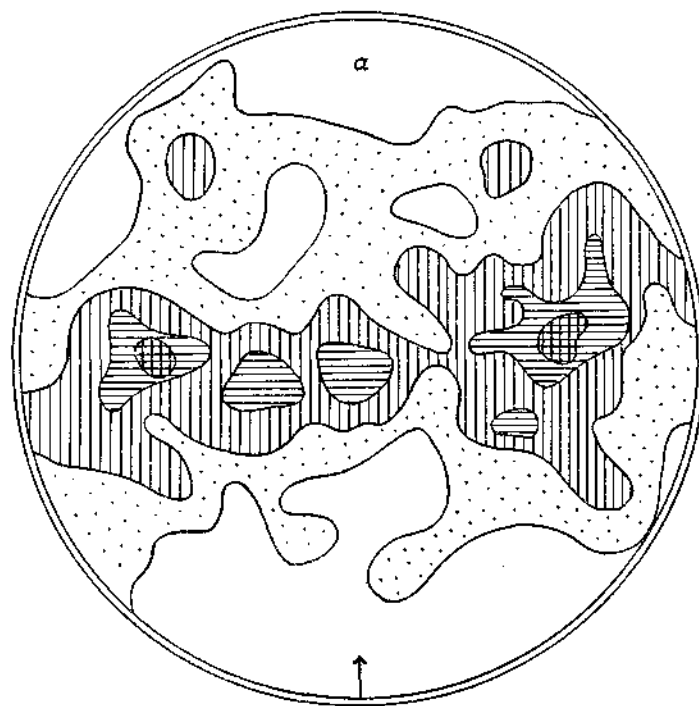
Abb. 10. Großoolith, Brunnenstein, Lage a, 0—1 mm von der Anwachfläche, 330 Achsenpole. Musterung wie in Abb. 9.
