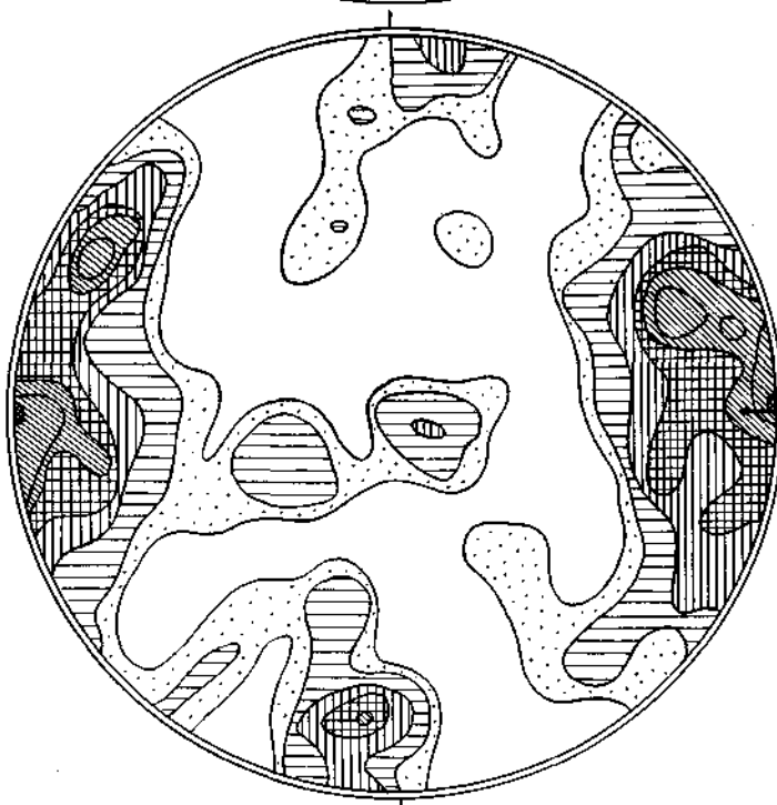
Abb. 36. Siluralkalkgang, Paß Thurn, Kalzite, 430 Achsenpole.
