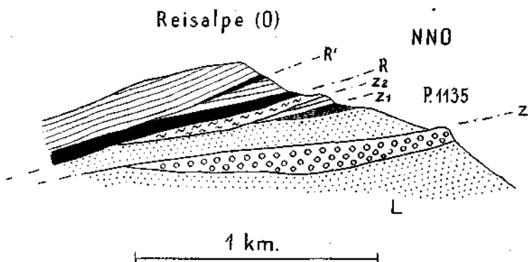
Fig. 10. Profil durch den östlichen Teil des Reisalpengipfels.
