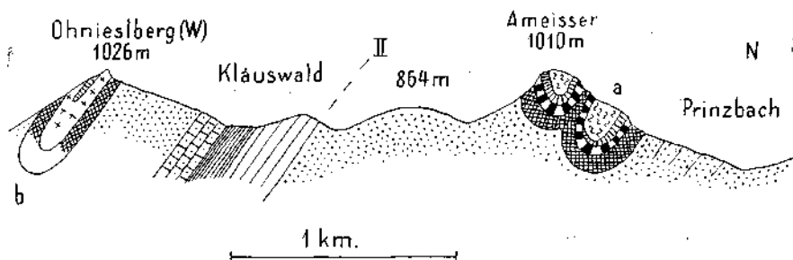
Fig. 3. Profil durch die Reitelmulde (a) und Eisensteinmulde (b).
