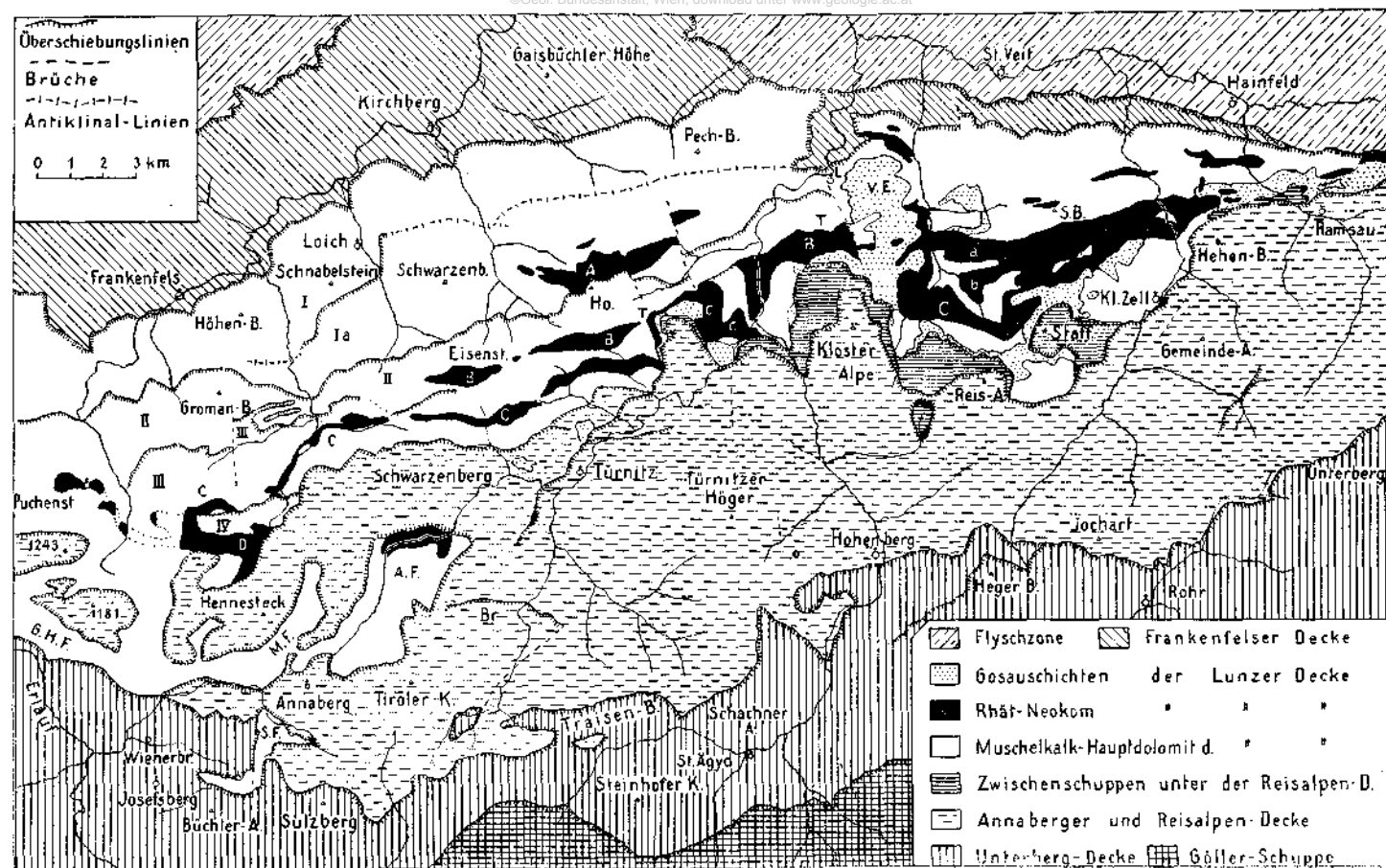
Fig. 1. Tektonische Übersichtskarte.
