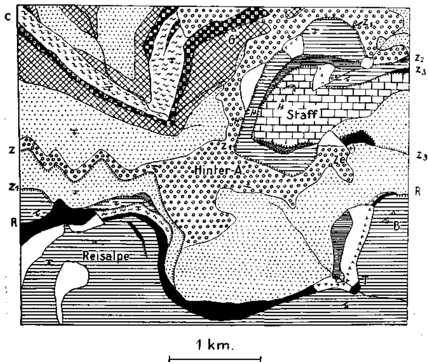
Fig. 11. Geologische Karte des Gipfelgebietes von Reisalpe und Staff.
