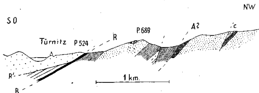
Fig. 8. Profil durch das Schuppengebiet nördlich von Türritz.
