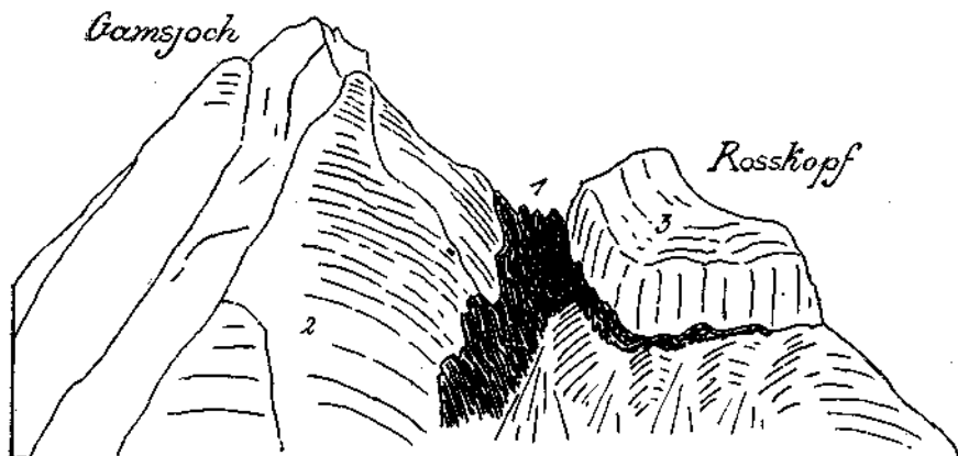
Fig. 6. Ansicht vom Phunssattel aus. 1 = Rauhwacken. 2 = Wettersteinkalk. 3 = Wahrscheinlich alte Oberflächenformen, die unter der Rauhwackenmasse begraben waren.
