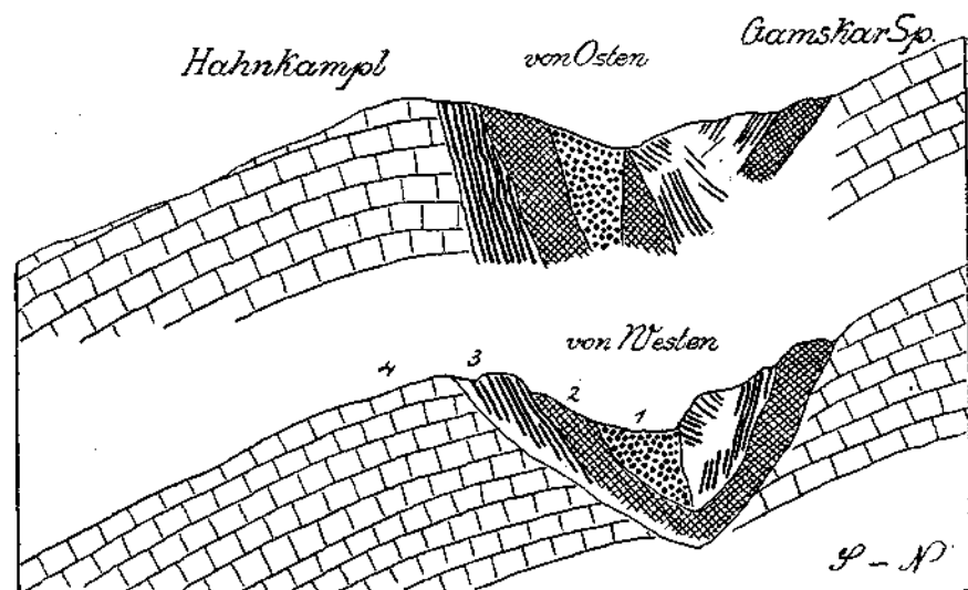
Fig. 2. 1 = Buntsandstein. 2 = Rauhwacken. 3 = Reichenhaller Kalko. 4 = Wettersteinkalk-Dolomit.
