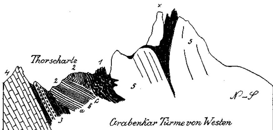
Fig. 8. 1 = Rauhwarcken und Mylonit der Reichenhaller Schichten. 2 = Muschelkalk. a = Dicke, helle Kalkbänke. b = Dünnschichtige Mergellagen mit Hornsteinknauerkalken. c = feste, lichte Kalklagen. 3 = Partnachschieben. 4 = Wohlgeschichteter Wettersteinkalk. 5 = Wenig geschichteter Wettersteinkalk. x = Große Schubscholle.
