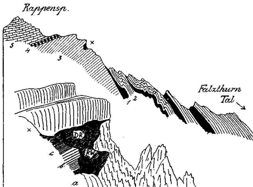
Fig. 3. 1 = Rauhacken. 2 = Reichenhaller Kalke. 3 = Wettersteindolomit. 4 = Raibler Schichten. 5 = Hauptdolomit. X = Tektonische Einschaltung. a = Wettersteindolomit. b = Dunkle Kalke. c = Dunkle Schiefer. DR = Dolomitbreccien. RW = Rauhacken.
