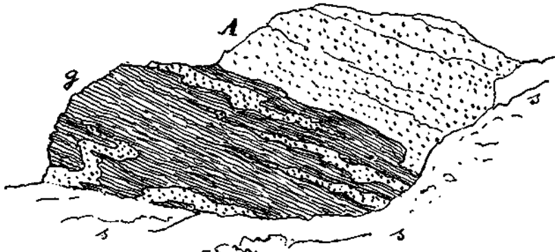
Fig. 2. Rundhöcker ober dem Rimmensee. Ansicht. A = aplitischer Granitgneiss g = feinkörniger Biotitgneiss s = Schutt.
