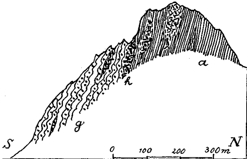
Fig. 6. Profil über die Mutterberger Seespitze (3298 m) a = hornblendereiche, dunkle Feldspatamphibolite h = Linsen und Lagen von großstrahligem Hornblendefels und Garbenamphibolit g = Perlgneis und Glimmerschiefer mit Albitknoten.
