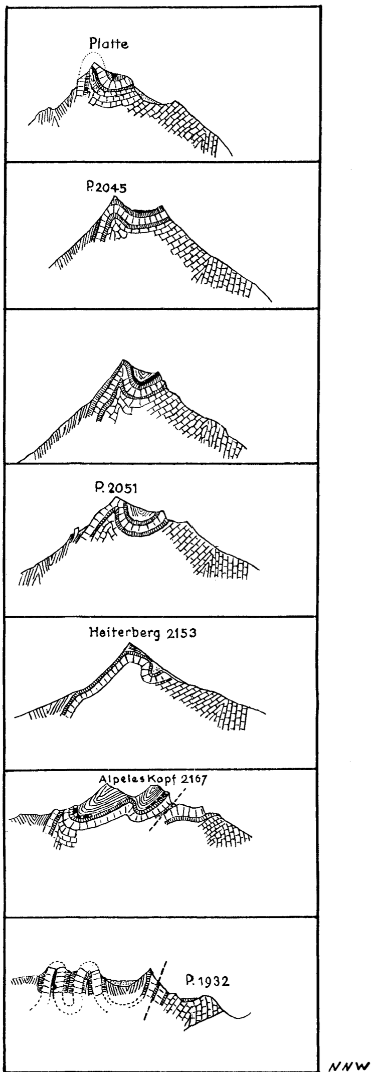
7 Querschnitte durch die Falten des Heiterbergs M. 1:25000
