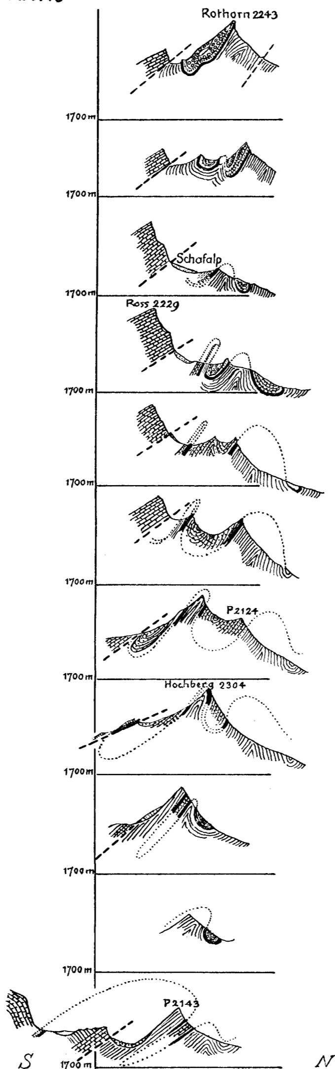
11 Querschnitte durch die Falten des Hochbergs und des Rothorns M. 1:25000
