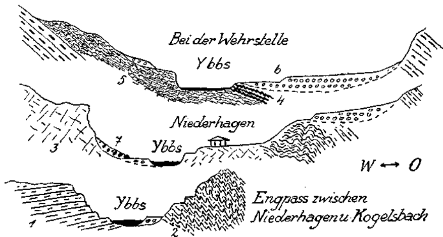
Fig. 28. 1 = Dickbankiger Muschelkalk. 2 = Dünn-schichtiger Muschelkalk. 3 = Ungeschichteter Muschelkalk. 4 = Rote Oberjura Hornsteinkalke. 5 = Graue Aptychenkalke und Neokommargel. 6 = Ybbschotter.
