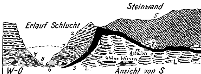
Fig. 22. 1 = Rauhacken. 2 = Muschelkalk. 3 = Lunzer Sandsteine. 4 = Schollen von Opponitzer Kalk. 5 = Mylonitischer Hauptdolomit. 6 = Rote Krinoidenkalke mit Manganerzkrusten. 7 = Neokommern. 8 = Konglomerat aus Erlaufschottern.
