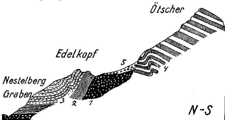
Fig. 7. 1 = Werfener Schichten, Rauhwacken, Gips, Mergel, bunt gemischt. 2 = Dünnschichtige Gutensteiner Kalk. 3 = Dickbankigere Kalk, Reifinger Kalk. 4 = Dachsteinkalk. 5 = Hangschutt.
