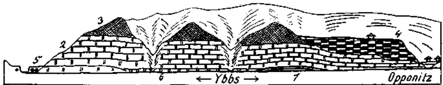
Fig. 36. 1 = Lunzer Schichten. 2 = Opponitzer Kalke. 3 = Rauhacken, bituminöser Dolomitmylonit, Anhydrit, Gips. 4 = Konglomerat aus Ybbschottern mit feineren gelblichen Mergel- und Sandsteinlagen. 5 = Konglomerat aus grobem Ybbschotter. 6 = Niedrige, unverkittete Schotterstufe.
