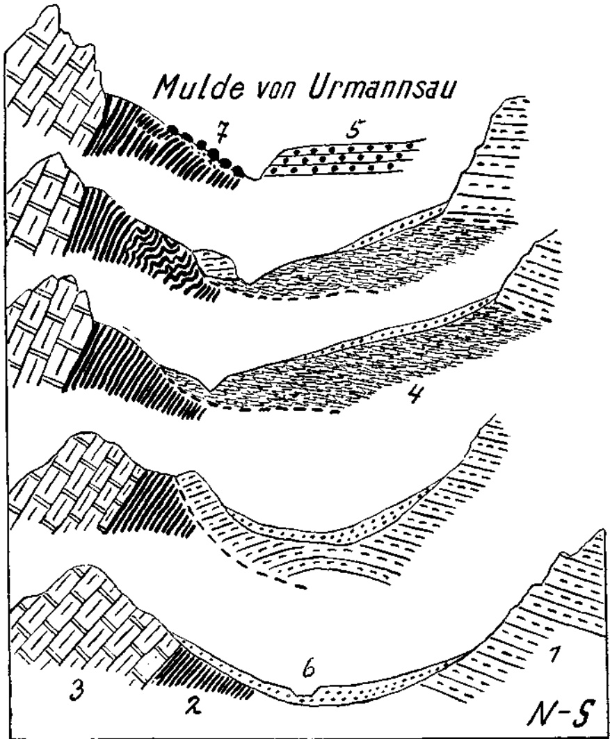
Fig. 21. 1 = Muschelkalk—Reifinger Kalk. 2 = Lunzer Sandsteine mit Kohlenflözen. 3 = Opponitzer Kälke. 4 = Neokommerngel. 5 = Konglomerat aus Erlaufschottern. 6 = Gebängeschutt. 7 = Blockwerk eines Bergsturzes.
