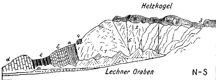
Fig. 3. 1 = Lichter, unterer Dolomit. 2 = Dachsteindolomit. 3 = Dachsteinkalk. 4 = Schollen von ungeschichtetem Dachsteinkalk (Lias ?), 5 = Steile Schußflächen. a = Gutensteiner Kalk. b = Raibler Schichten. c = Opponitzer Kalk.
