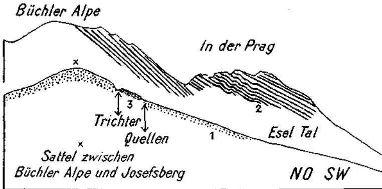
Fig. 15. 1 = Rote und grüne Werfener Schiefer, Rauhwacken. 2 = Wohlgeschichteter, stellenweise lebhaft gefalteter, dünnstiefiger Muschelkalk. 3 = Kleinstückige, schwarze, glatte Tonschieferstückchen, Reingrabner Schiefer.
