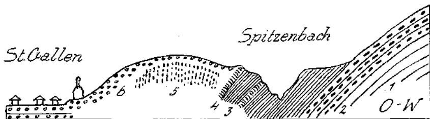
Fig. 29. 1 = Hauptdolomit. 2 = Rote Jurakalke mit roten Hornsteinen. 3 = Sehr gleichmäßige milde Neokommerngel. 4 = Festere, etwas gefleckte kalkige Lagen. 5 = Rote Mergel und Sandsteine mit bunten Geröllen — Gosauschichten. 6 = Konglomerierte Schotter.
