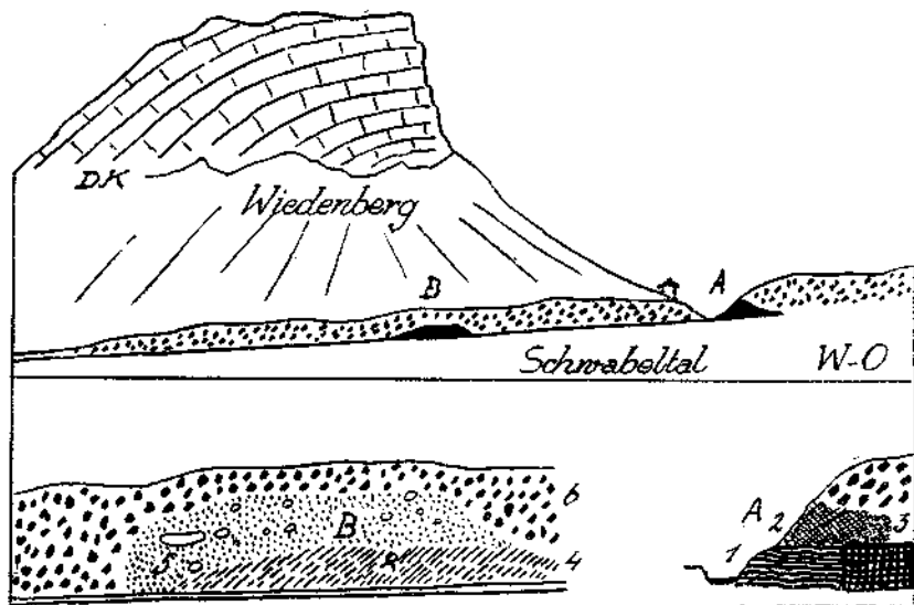
Fig. 12. DK = Dachsteinkalk. Aufschluß A: 1 = Feine, dünnblättrige, grünliche Gipstonschiefer. 2 = Gelbe Rauhwacke. 3 = Gutensteiner Kalk, zertrümmert. Aufschluß B: 4 = Blaugraue, weiche Gosaumergel. 5 = Grundmoräne mit geschliffenen Blöcken. 6 = Grobes, kantiges Kalkblockwerk, Endmoräne der Schlußeiszeit.
