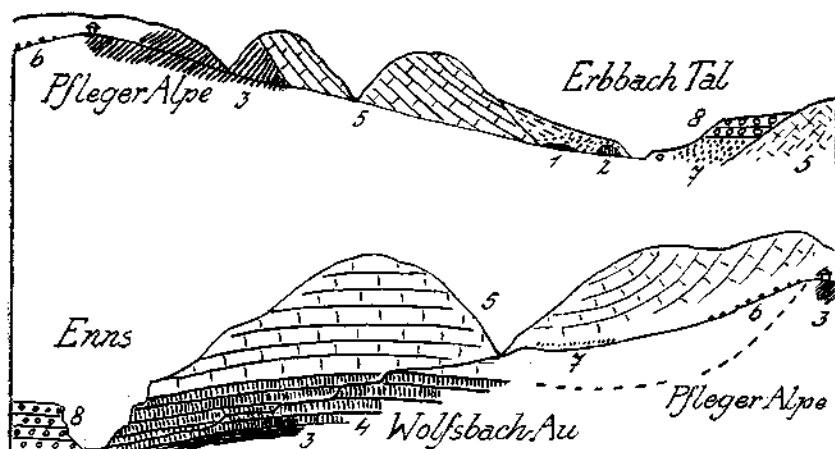
Fig. 37. 1 = Werfener Schichten. 2 = Dunkler Triaskalk. 3 = Lunzer Sandsteine, Tonschiefer, Pflanzensandsteine. 4 = Opponitzer Kalke. 5 = Hauptdolomit. 6 = Exotische Gosauergölle. 7 = Grundmoräne. 8 = Konglomerierte Schotter.
