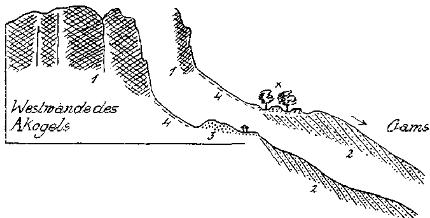
Fig. 20. 1 = Dachsteinkalk. 2 = Gosauschichten mit Pechkohlen. X = Alte Schürfruben. 3 = Endmoränenwall. 4 = Hangschutt.
