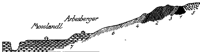
Fig. 17. 1 = Werfener Schichten. 2 = gelbe Rauhwacken. 3 = Gutensteiner Kalk. 4 = Dachsteinkalk und Liaskrinoidenkalk. 5 = Bunte, kalkreiche Gosaukonglomerate. 6 = Gosauergel und Sandsteine. 7 = Konglomerat aus bunten, groben, ungleichen Enusschottern mit einzelnen Sandlagen.
