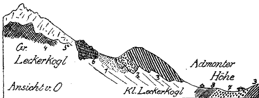
Fig. 43b. 1 = Werfener Schichten. 2 = Rauhwacken. 3 = Gutensteiner Kalke. 4 = Dachsteindolomit. 5 = Dachtseinkalk. 6 = Dickschichtiger, blaßrötlicher Liaskalk. — Gosauschichten: 7 = Konglomerate und Breccien. 8 = Sandsteine und Mergel.
