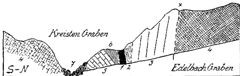
Fig. 26 b. 1 = Grüne, teigartige Werfener Schichten. 2 = Brännlicher Dolomit-Kalkschiefer-Mergel. 3 = Wettersteinkalk. 4 = Hauptdolomit. 5 = Geschichteter Hauptdolomit. 6 = Braune Mergel und Sandsteine der Gosauschichten. 7 = Grobes Blockwerk von lichtem Kalk. X = Linie, an der die Absträgung der Raibler Schichten erfolgte.
