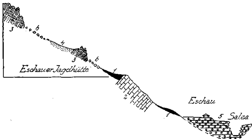
Fig. 22. 1 = Grüne Werfener Schichten mit Raubwacken und schwarzen Kalken. 2 = Hauptdolomit. 3 =LICHTER, elfenbeinfarbener Dachsteinkalk. 4 = Gelblichgraue, weiche, poröse Sandsteine der Gosauschichten. 5 = Konglomerate der Salzschotter. 6 = Blockwerk von 3.
