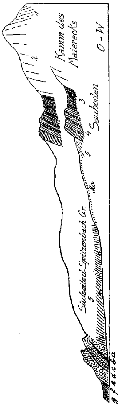
Fig. 30. 1 = Rötlicher Kalk, 2 = Wettersteinkalk, 3 = Rötlicher Schichten, 4 = Opporitzer Kalk und Dolomit, 5 = Feines Dolomitkonglomerat, Gerölle Kirschengrube, b = Mächtige, dickbankige Zementmergel, c = Feste, blaugraue Mergel und Kalksandsteine, wechsellagert mit Dolomitlebreccien, d = Dünnbankige Mergel, e = Mächtige Dolomitlebreccien, f = Zementmergel, g = Kalk, Mo = Moränenwall.
