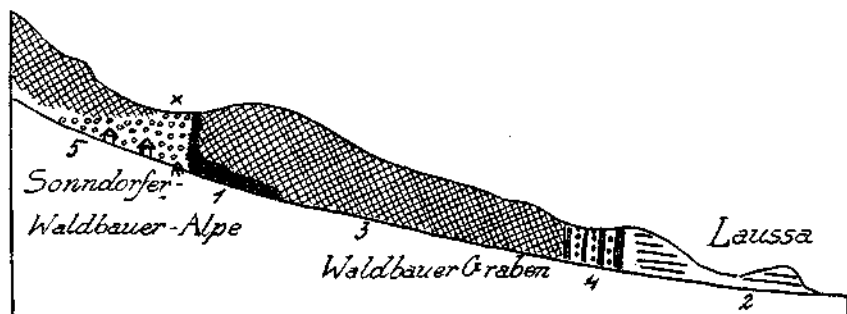
Fig. 41 b. 1 = Grüner Teig von Werfener Schichten und graue poröse Rauhwacken. 2 = Opponitzer Kalk. 3 = Mylonitischer Dolomit. 4 = rötlich zementierte Kalkbreccien und Konglomerate mit großen Brocken von Bauxit, Kalke, Mergel und Sandsteine — Gosauschichten. 5 = Zahlreiche Gerölle und Blöcke von Quarzsandsteinen, rote, grüne, violette, glimmerige Schiefer, lichte grüne Schiefer, Verrucano. x = am Sattel bunte Gesteine und Rauhwacke.
