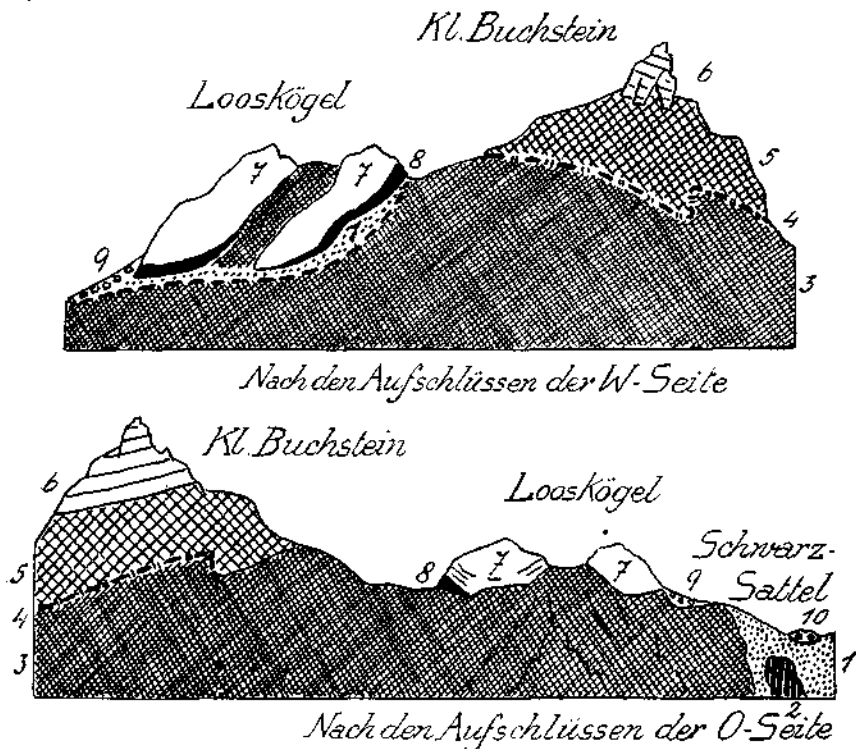
Fig. 2. 1 = Werfener Schichten. 2 = Scholle von Gutensteiner Kalk. 3 = Ramsaudoomit. 4 = Raibler Schichten. 5 = Dachsteindolomit. 6 = Dachsteinkalk. 7 = Schollen von Dachsteinkalk. 8 = Liaskalke. 9 = Gosauschichten. 10 = Blockwerk aus 6.
