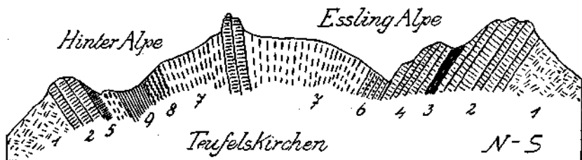
Fig. 27. 1 = Hauptdolomit. 2 = Lichte, dickbankige Kalke. 3 = Mergelige Kalke. 4 = Feste, gutgeschichtete, gelbliche Kalke. 5 = Liaskrinoidenkalke. 6 = Hornsteinkalke, sandig verwirrende streifige Kalke mit Pentakrinus und Hornsteinstückchen. 7 = Grüne Hornsteinkalke, weißliche, blaßrötliche Kalklagen. 8 = Aptychenkalke. 9 = Nockmergel mit feinen Sandsteinslagen.
