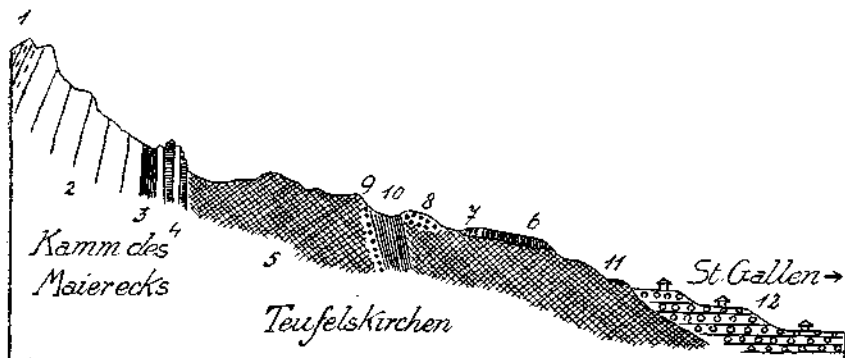
Fig. 33. 1 = Raibler Schichten. 2 = Wettersteinkalk. 3 = Opponitzer Kalk. 4 = Hauptdolomit. 5 = Rote Krimoidenkalk. 6 = Graue, gefaltete Aptychenkalk. 7 = Buntes Gosaukonglomerat. 8 = Feines Dolomitskonglomerat. 9 = Graue Gosauergel. 10 = Höchste Schotter bei 660 m. 11 = Konglomerierte Schotter, sehr viel zentralalpines Gerölle, dicker Überzug von Verwitterungslehm.
