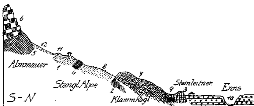
Fig. 8. 1 = Werfener Schichten, feste, grüne und rote Sandsteine und Tonschiefer. 2 = Haselgebirge. 3 = Dunkler Triaskalk. 4 = Weißer Dolomit. 5 = Dachsteindolomit. 6 = Dachsteinkalk. 7 = Dünnschichtige, stark gefaltete Aptychenkalk. 8 = Exotische Gosangerölle. 9 = Grundmoräne mit vielen großen, prachtvoll geschliffenen Blöcken; Kalk, Granatamphibolite, Granite, Quarzite, Grünschiefer, Gneise. 10 = Konglomerat aus Ennschottern. 11 = Endmoräne. 12 = Hangschutt.
