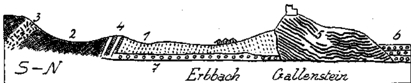
Fig. 38. 1 = Werfener Sandsteine, rötlich und grau. 2 = Tonschiefer, grauviolett. Letten. 3 = Rauh- wacken. 4 = dunkelgraue Kalke. 5 = Gutensteiner Kalke. 6 = konglomerierte Ennsschotter. 7 = Schotter des Erbbaches.
