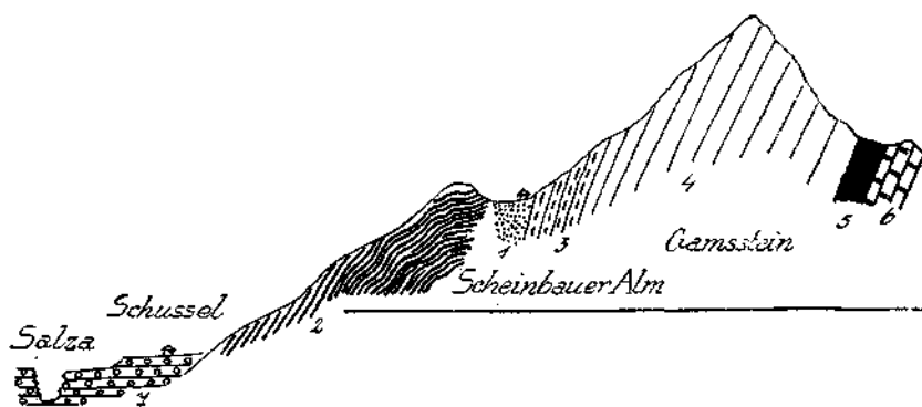
Fig. 25a. 1 = Werfener Schichten. 2 = Gutensteiner und Reiflinger Kalke. 3 = Horstein führender Wettersteinkalk. 4 = Wettersteinkalk. 5 = Raibler Schichten. 6 = Oppenitzer Kalke. 7 = Salzaschotter.
