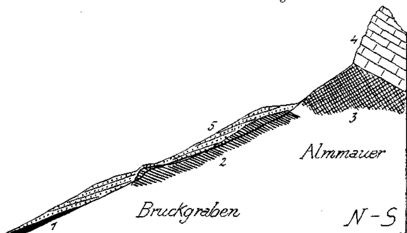
Fig. 7. 1 = Werfener Schichten. 2 = Mächtige schwarze Tonschiefer der Raibler Schichten. 3 = Dachsteindolomit. 4 = Dachsteinkalk. 5 = Große Halden von Gebügeschutt.
