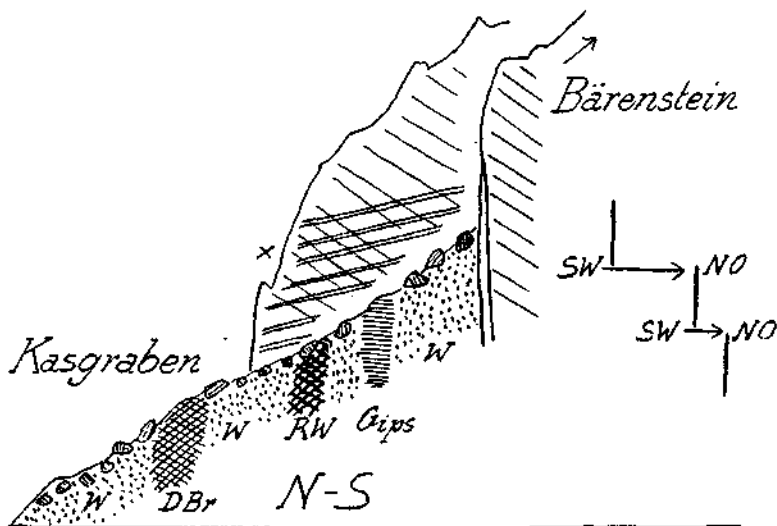
Fig. 6b. W = Werfener Schichten, grüne glimmerige Tonschiefer und Sandsteine. RW = Rauhbacken. DBr = Dunkle, aschgraue Dolomithbreccien, dunkle, dünnsschichtige Kalklagen. Gips = Gips, Gipsstone, grüne, graue Gipsdolomithbreccien. x = Die doppelten Striche bedeuten Rutschstreifen.
