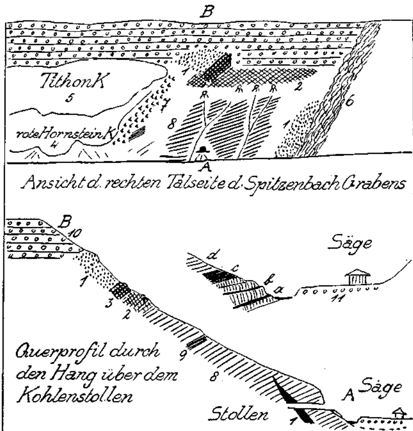
Fig. 31. 1 = Werfener Schichten. 2 = Rauhwacken. 3 = Gutensteiner Kalk. 4 = Rote Hornsteinkalke. 5 = Titthonkalke. 6 = Heftig gefaltete Aptychenkalke. 7 = Titthonkalkebreccie. 8 = Milde, dunkelgraue Gosau-mergel mit Kohlenflözen. 9 = Ziegelrote Mergel und Kalkbreccie. Aufschluß beim Kohlenstollen: a = Kohlenflöz = 2–3 dm. b = Kohlenflöz = \frac{1}{2} dm. c = Schwarze kohlige Mergel. d = Graue Gosau-mergel. 10 = Konglomerierte Schotter.
