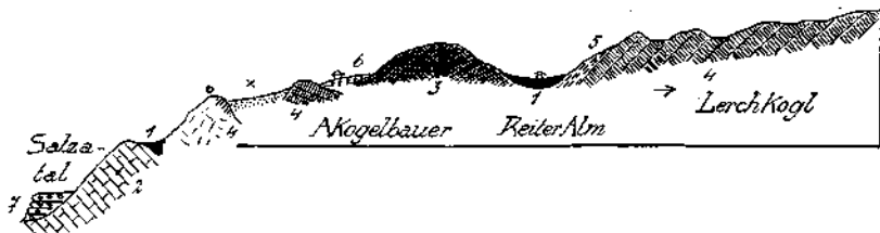
Fig. 21. 1 = Werfener Schichten. 2 = Hauptdolomit. 3 = Dachsteindolomit. 4 = Dachsteinkalk. 5 = Oberalm Kalk. 6 = Gosaubreccien. 7 = Salzschotter. o =LICHTER Kalk mit Resten von Rudisten. x = Gosausandsteine mit vereinzelt exotischen Geröllen, Porphyre, Kiesel.
