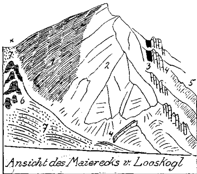
Fig. 34. 1 = Reiflinger und Gutensteiner Kalk. 2 = Wettersteinkalk. 3 = Raibler Schichten. 4 = Opponitzer Kalk. 5 = Hauptdolomit. 6 = Liaskrinoidenkalk. 7 = Gosauschichten. X = Sattel der Admonter Höhe.
