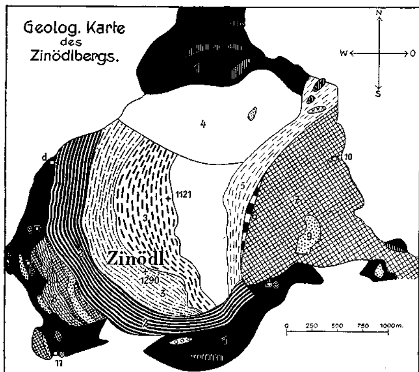
Fig. 39. 1 = Werfener Schichten. 2 = Gutensteiner Kalk. 3 = Dunkle, bituminöse Kalk, Reiflinger Kalk, Krinoidenkalk. 4 = Wettersteinkalk und Dolomit. 5 = Raibler Schichten. 6 = Opponitzer Kalk. 7 = Hauptdolomit. 8 = Jurakalk. 9 = Gosauschichten. 10 = Grundmoräne. 11 = Doline. a = Stollen. b = Rösche. c = Stollen. d = Stollen. e = Stollen. ‡ Profile dazu liefert Fig. 25.
