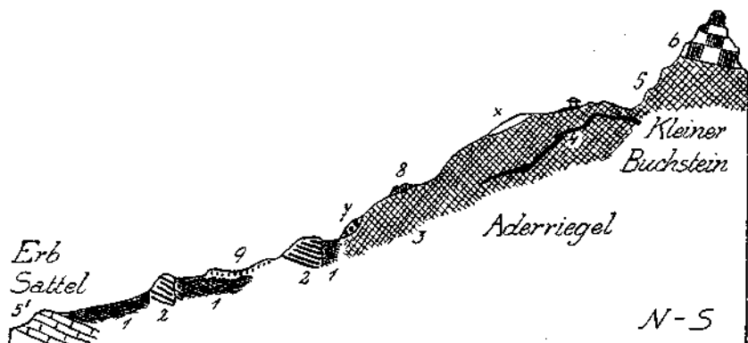
Fig. 4. 1 = Werfener Schichten. 2 = Gutensteiner Kalk. 3 = Ramsaudolomit. 4 = Raibler Schichten. 5 = Dachsteindolomit. 5' = Hauptdolomit. 6 = Dachsteinkalk. 7 = Gosauschichten. 8 = Gehängebreccie. 9 = Moränenwälle. x = Rauchwackige, graue Kalko der Raibler Schichten.
