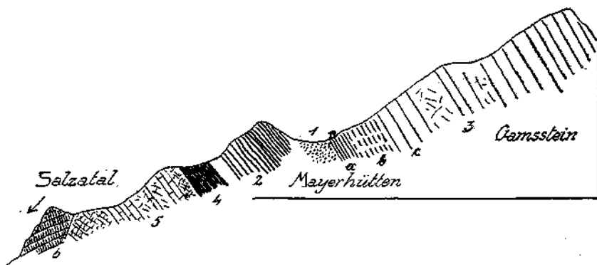
Fig. 24. 1 = Werfener Schichten. 2 = Gutensteiner Kalke, Reiflinger Kalke. a = Lichter Wettersteinkalk. b = Hornsteinlagen und Hornsteinknollenkalke. c = Ungeschichteter lichter Kalk. 3 = Wettersteinkalk. 4 = Raibler Schichten. 5 = Hauptdolomit. 6 = Dachsteinkalk.
