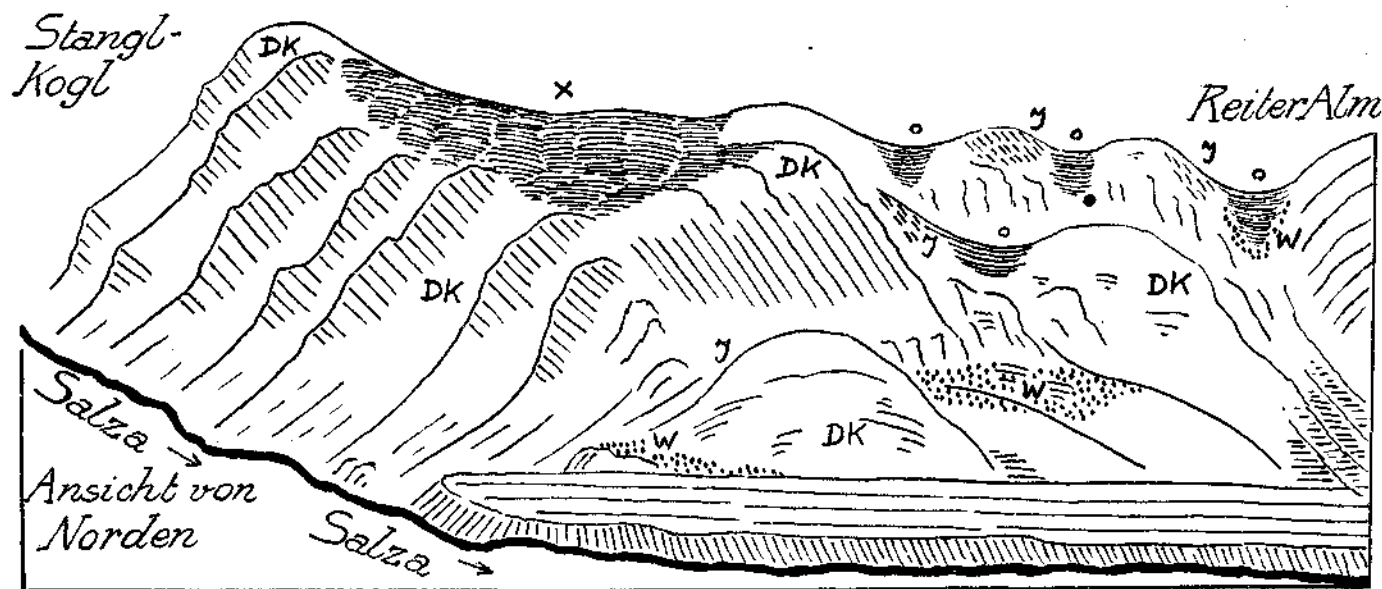
Fig. 16a. W = Worfener Schichten. DK = Dachsteinkalk. J = Oberalmer Kalk. X = Fläche der Einrundung. o = Alte Quertalfurchen. • = Quarzgerölle in der Quertalfurche. Am Fuß des Gebirges die Terrasse aus den Salzaschottern.
