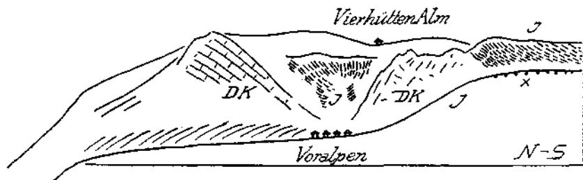
Fig. 14. DK = Dachsteinkalk. J = Oberalmer Kalke, lichte graue Kalke mit Hornsteinlagen. X = Quarzgerölle in der alten hohen Quertalfurche.
