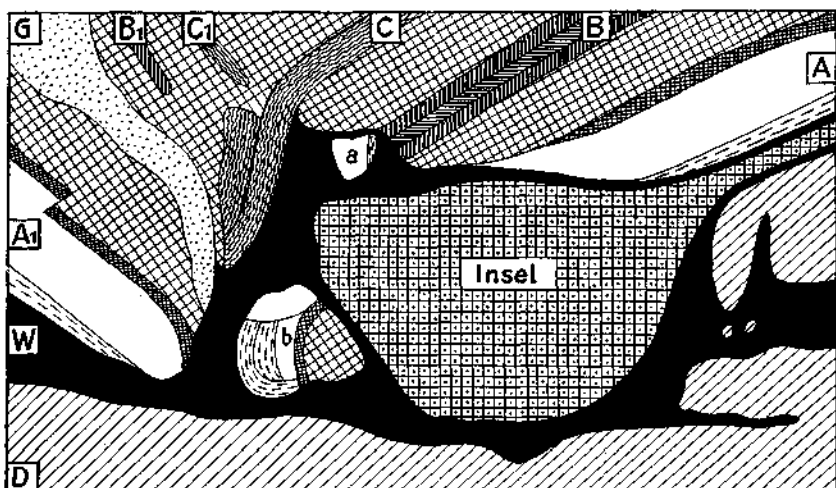
Fig. 40. D = Gebiet des vorherrschenden Dachsteinkalkes. W = Schubmasse aus Werfener Schichten und vielen Schollen. Insel = Bezeichnung für die zentrale Schubmasse. A 1 = Maierreckzug. A = Gamssteinzug. G = Großer Gosauzug. B 1 = Bodenwieszug. B = Voralpenzug. C 1 = Hochbrandzug. C = Oisbergzug. a = Scholle des Hainbachsteins. b = Scholle des Zinödl.
