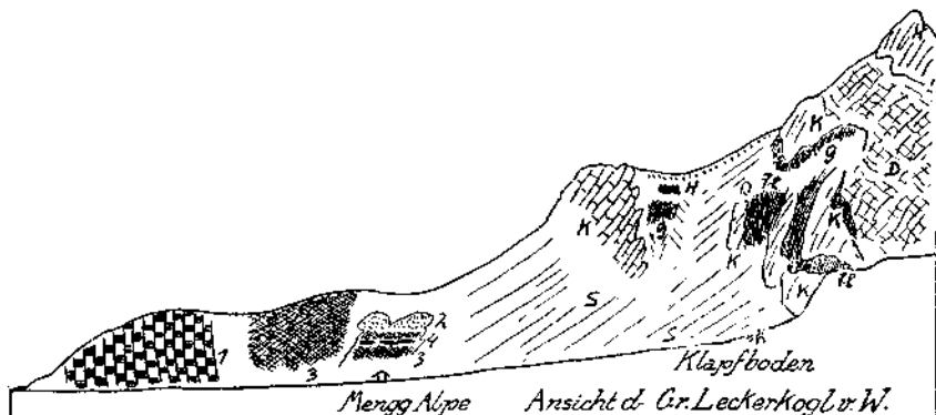
Fig. 43a. 1 = Quarzitäbanke der unteren Werfener Schichten. 2 = Grüne, rote Werfener Schichten mit Haselgebirge. 3 = Rauhwacken. 4 = Dunkle Triaskalke. D = Dachsteindolomit. K = Dachtseinkalk. H = Fleckenmergel. H = Masse von schwärzlichen und grünlichen Hornsteineu. G = Gosausandsteine mit Phyllitstückchen. S = Schutthaldeu.
