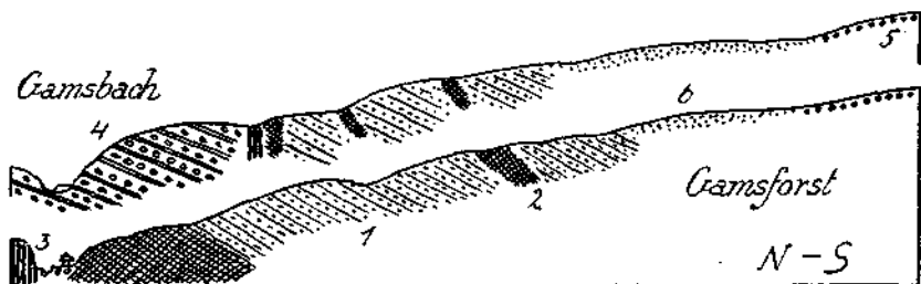
Fig. 18. 1 = Grüne Sandsteine der Werfener Schichten mit einzelnen roten Lagen. 2 = Rauhwacken. 3 = Gutensteiner Kalk. 4 = Konglomerate, Sandsteine und Mergel der Gosauschichten. 5 = Reiche exotische Gerölle der Gosauschichten. 6 = Wenig bearbeitete Grundmoränen der Schlußzeit.
