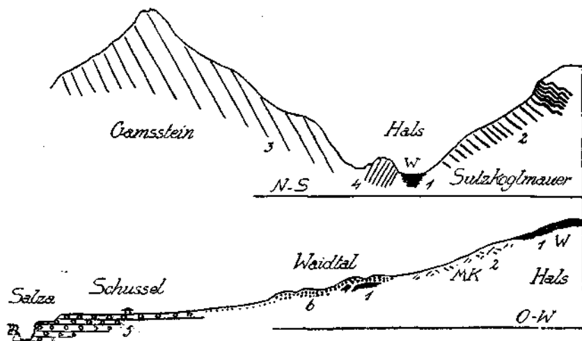
Fig. 25b. 1 = Werfener Schichten. 2 = Gutensteiner und Reiflinger Kalke. 3 = Wettersteinkalk. 4 = Scholle von hellgrauem Kalk. 5 = Konglomerierte Salzaschotter. 6 = Endmoräne der Schlußeiszeit.
