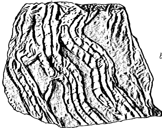
a) Dreigliedriger Ausguß einer Fährte ( Subphyllochora n. g. ). Greifensteiner Sandstein, Kollektion Toulà (zirka \frac{3}{7} nat. Gr.). b) Ausguß einer dreigliedrigen Fährte ( Subphyllochora n. g. ). Greifensteiner Sandstein, Höflein an der Donau (zirka \frac{1}{2} nat. Gr.).
