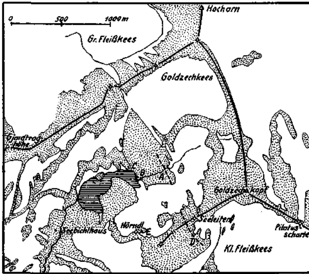
Fig. 1. Verbreitung der Ganggesteine am Zirmsee. Punktiert: Grundgebirge (Zentralgneis und Schieferhülle); weiß: Gletscher, Moränen und Gehängeschutt; unterbrochene schwarze Linien: Ganggesteine.
