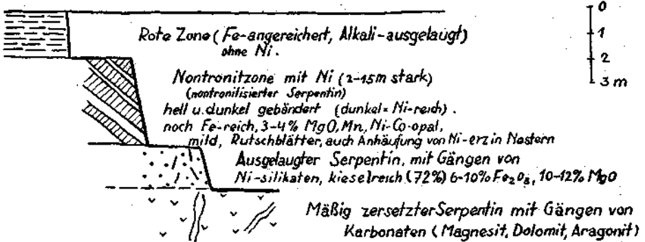
Abb. 5. Profil durch die Aidarbak-Ni-Erzlagerstätte bei Orsk (nach den Angaben der Exkursionsführung).
