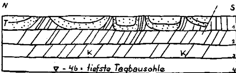
Tagbau-Längssicht-Ostseite
