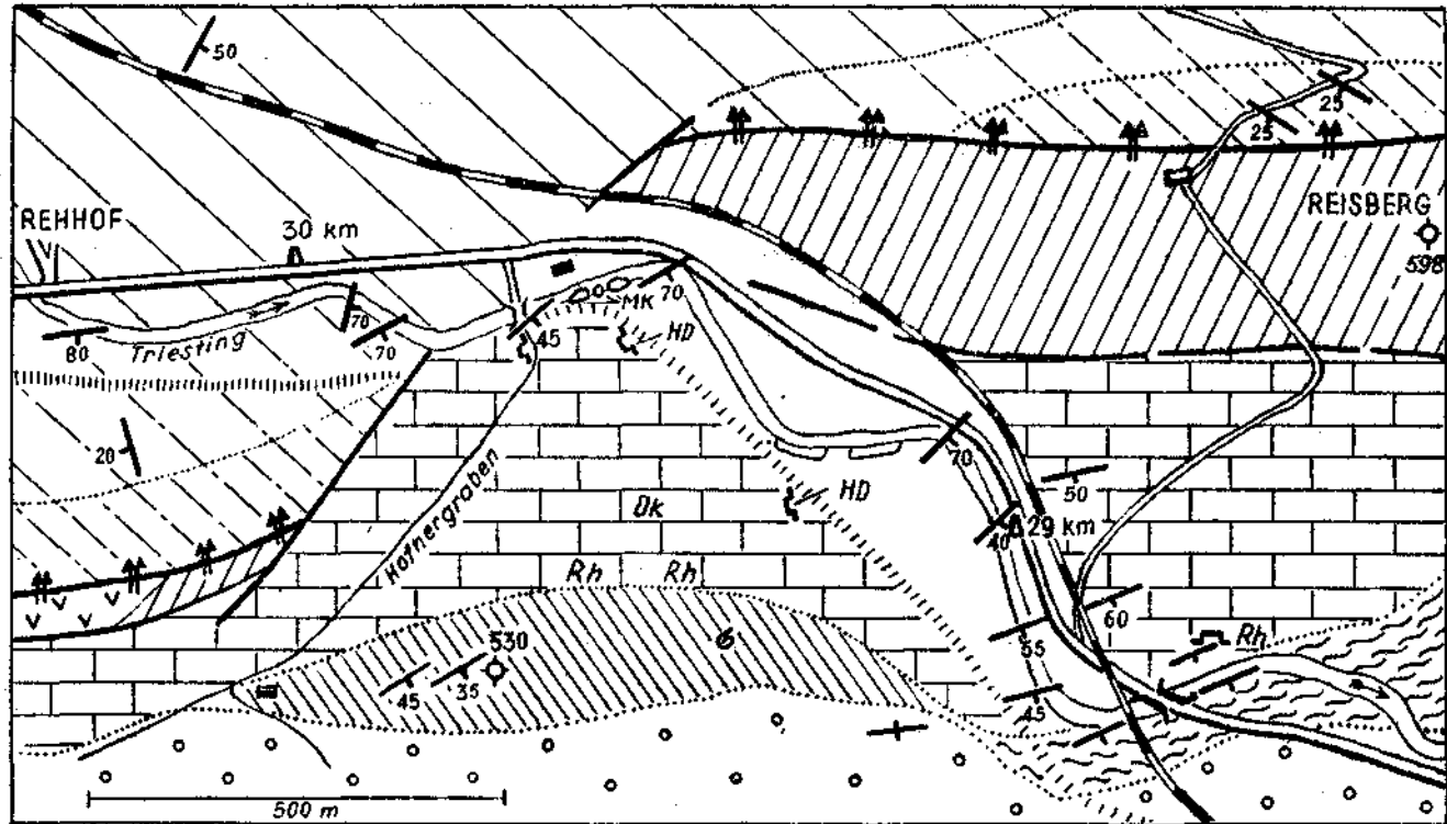
Abb. 2. Detailskizze des Triestingdurchbruches bei km 29. (Zeichenerklärung siehe Tafel 1.)
