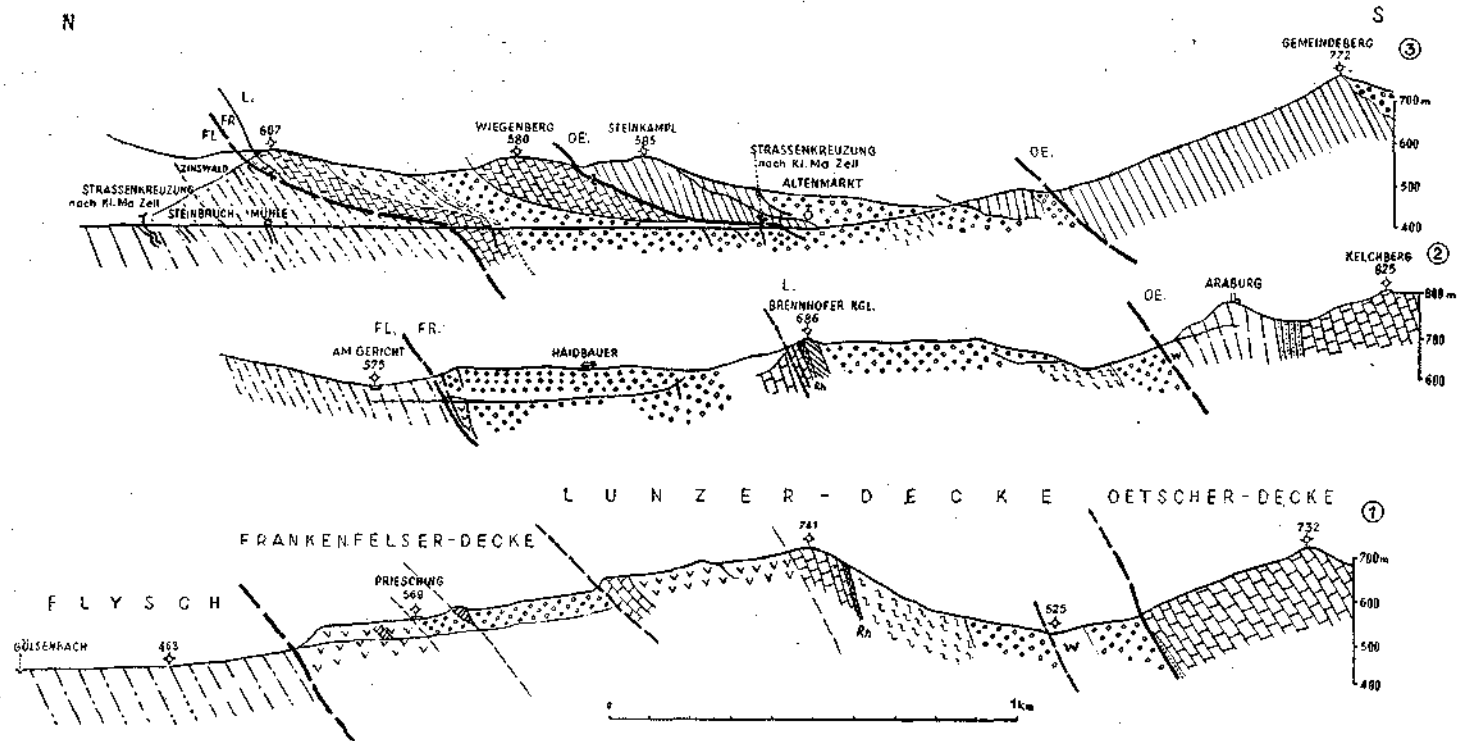
Abb. 1. Profile durch den Kalkalpenrand bei Kaumberg. (Zeichenerklärung siehe Tafel 1.)
