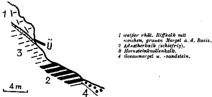
Abb. 3. Aufschlußprofil an einem Wasserriß zum Rigausbach südlich der Moosbergalm.
