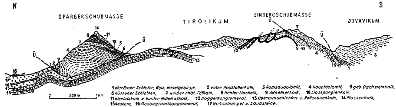
Abb. 5. Profil durch die Sparber- und Einberg-Schubmasse.
