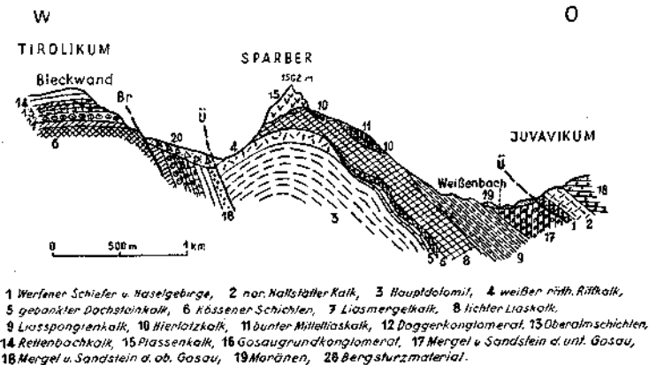
Abb. 4. Profil durch die Sparber-Schubmasse.
