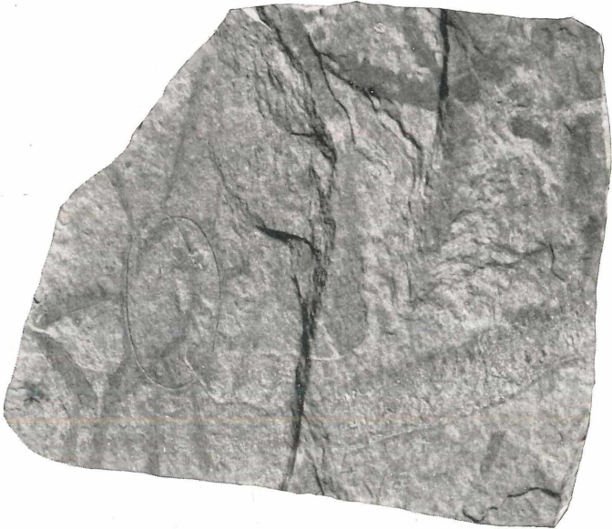
Cyrtograptus Törnquisti nov. spec. Aus dem Obersilur am Sieglitzberg bei Lobenstein.
