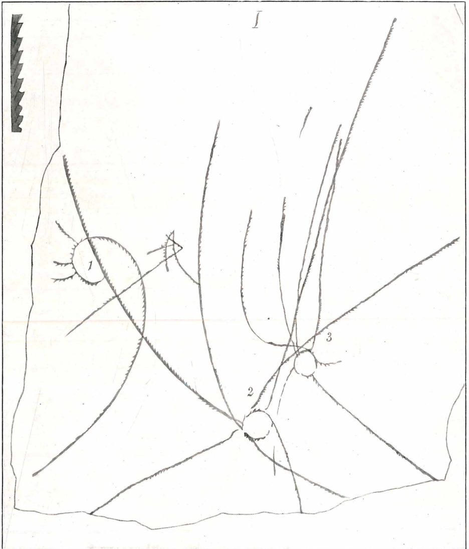
Cyrtograptus Lundgreni , Tullberg und Var. Trilleri (nov.) Eisel. (Fig. 1) (Fig. 2 und 3)
