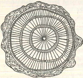
Fig. 7. Querschnitt der Dilleniacee : Doliolepis Rolandri . Schmalere Bastringe, breite Holzringe mit verbreiterten Markstrahlen. Kork ziemlich dick. Natürl. Größe.
