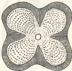
Fig. 4. Querschnitt einer Bignoniee .
