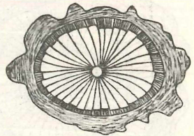
Fig. 6. Querschnitt der Composite: Mikania spec. Schwache Furchung, breite Markstrahlen, dicker Kork. Natürl. Größe.
