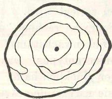
Fig. 8. Querschnitt der Polygalacee : Securidaca spec. Bast durch einfache Linien angedeutet. Wenige Anastomosen zwischen je zwei Ringen. Natürl. Größe.
