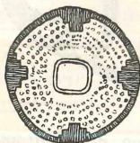
Fig. 3. Querschnitt einer Bignoniee .
