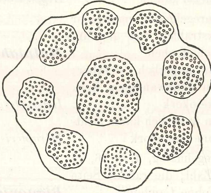
Fig. 11. Querschnitt der Sapindacee : Serjania multiflora .
