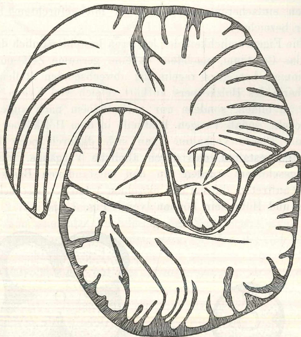
Fig. 5. Zwei ineinander gewachsene Stämme der Malpighiaceae : Tetrapteris spec. Furchung unregelmäßig und oft sehr tief. Natürl. Größe.
