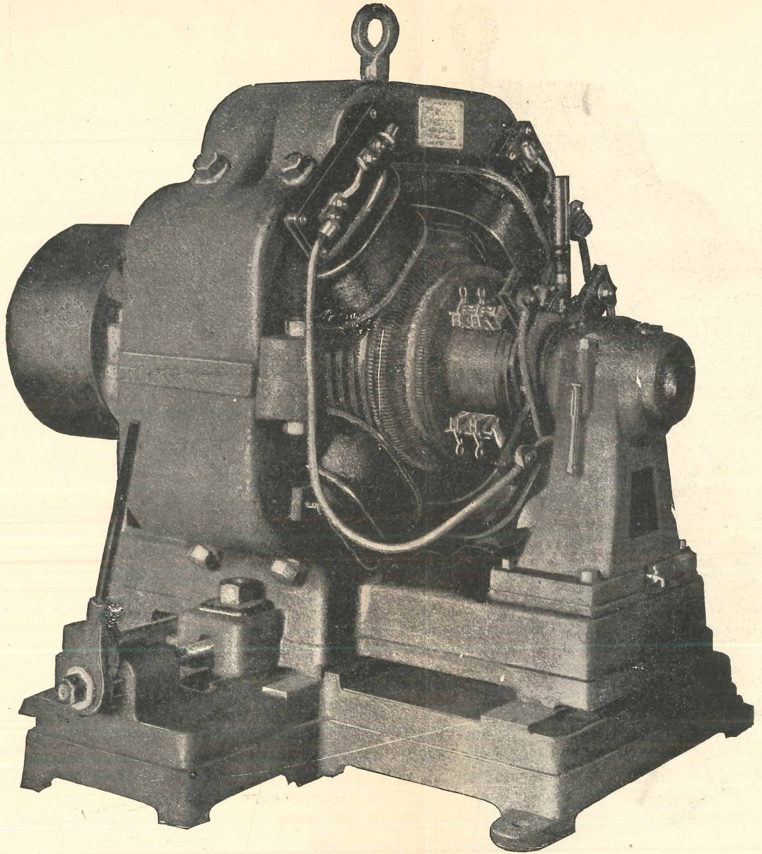
Thomson-Houston-Stromerzeuger für die Nord-Süd-Bahn, vierpolig, mit Riemenantrieb, 600 Umdrehungen, 500 Volt, 200 Ampère.
