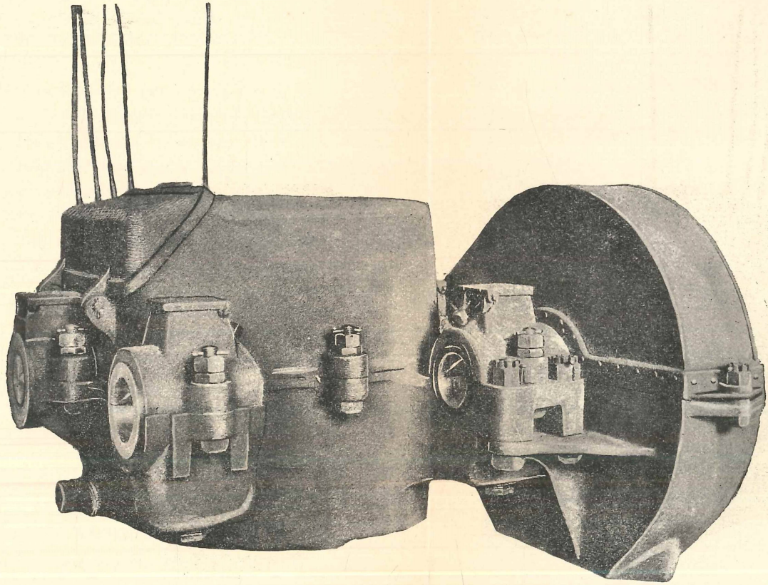
Thomson-Houston-Straßenbahnmotor, komplett mit Magnetgehäuse und Zahnradkasten, 810 kg schwer; 525 Umdrehungen bei 16 km, normal 20 P. S.
