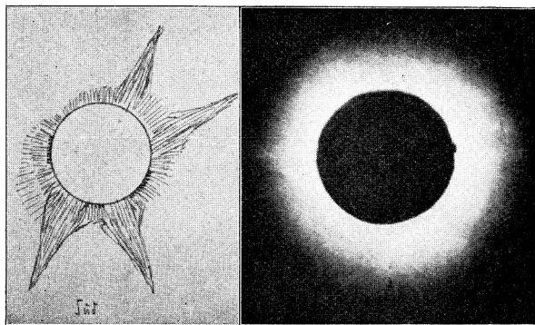
Abb. 13. Sonnencorona nach Zeichnung und Photographie.
