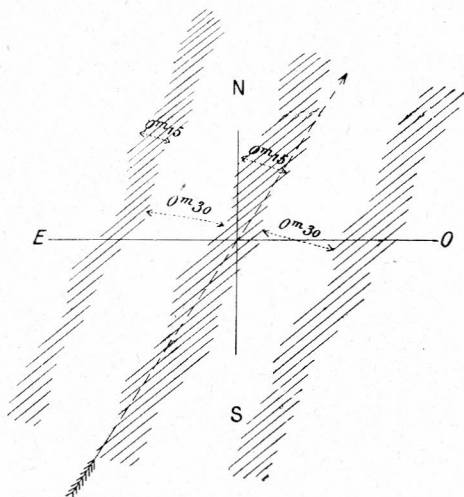
Abb. 12. Finsternisbände. (Nach G. Quignon).
