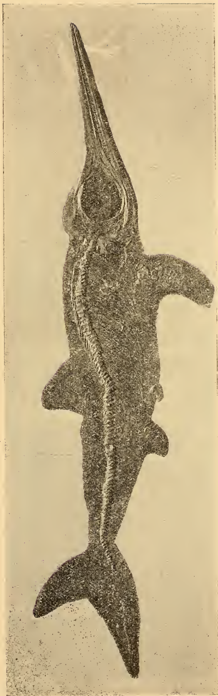
Fig 1. Ichthyosaurus quadrisissus . \frac{1}{3} nat. Gr.
