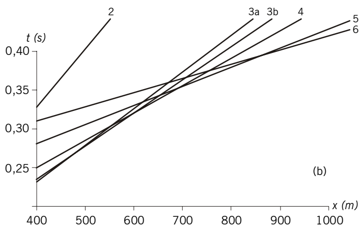
Abb. 1: Die Laufzeitkurve von SP 4 der Linie 1 über die Entfernung x und Laufzeit t . (a) Die gesamte Laufzeitkurve: Entfernung 0 bis 1080 m. Die Laufzeitäste von Horizont 3b, 4 und 5 sind als erste Einsätze mühsam unterscheidbar. (b) Etwas vergrößerte Laufzeitkurve: Entfernung 400 bis 1040 m. Alle Laufzeitäste sind als erste Einsätze erkennbar und interpretierbar.
