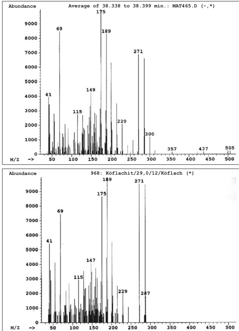
Abb. 4: Oben: Massenspektrum des Peaks mit der Retentionszeit 38,36 Minuten. Molekülmasse dieser nicht identifizierten Substanz: 286. Unten: Vergleichsspektrum einer offensichtlich identischen Substanz aus einer Probe des Köflachits (Obere Aufnahme: 25 m-Säule; untere Aufnahme: 12 m-Säule).
