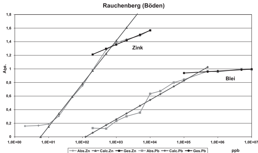
Abb. 3: Eichkurven für Pb und Zn.
