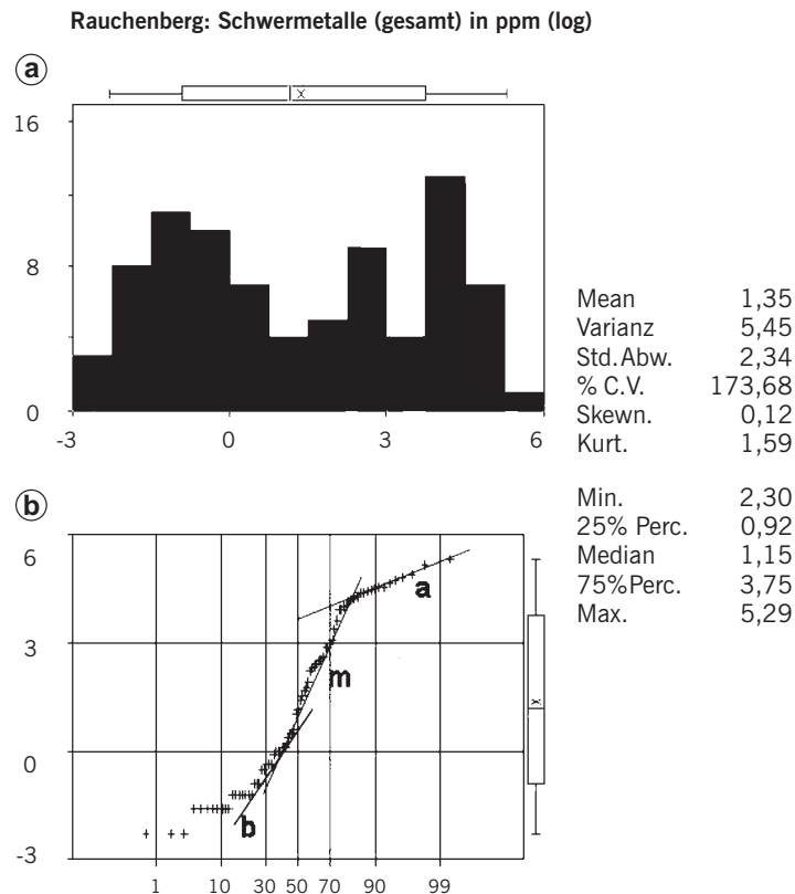
Abb. 5: a) Histogrammdarstellung der logarithmisch umgeformten Messwerte; b) Darstellung der logarithmisch umgeformten Messwerte in der Wahrscheinlichkeitsskalierung.
