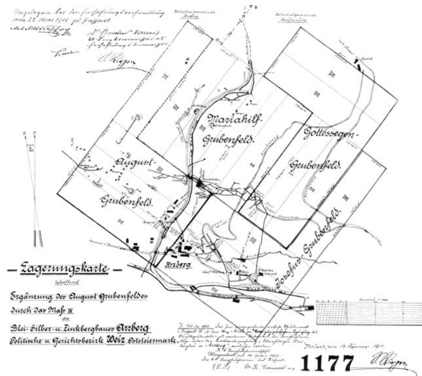
Abb. 1: Lagerungskarte des Erzberger Reviers. Die Einbaue des Rauchenberges befinden sich im „August Grubenfeld“ (Archiv Montanbehörde Süd).
