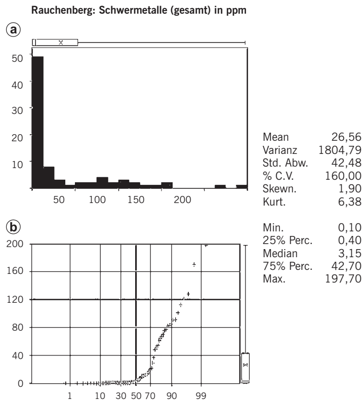
Abb. 4: a) Histogrammdarstellung der Messwerte; b) Darstellung der Messwerte in der Wahrscheinlichkeitsskalierung.
