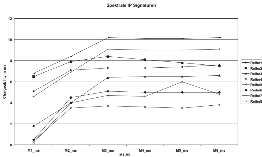
Abb. 13: Spektrale Charakteristik der IP-Anomalien am Profil Rauchenberg (2004).
