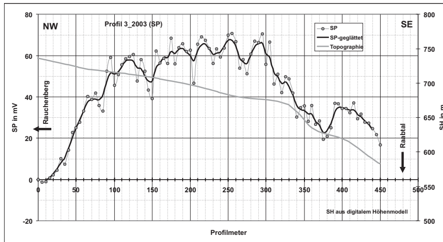
Abb. 2: Eigenpotentialmessung am Rauchenberg (Profil 3-2003) mit Topografie.
