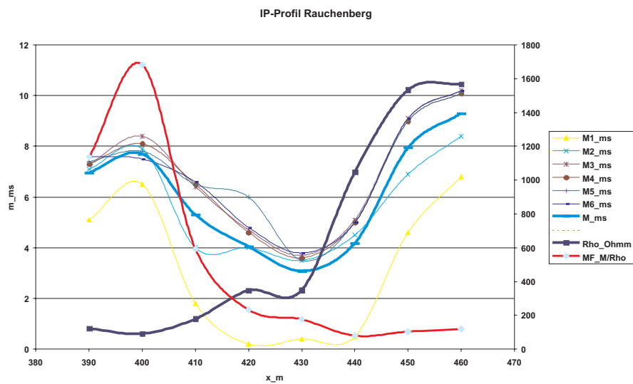
Abb. 12: IP-Profilmessungen am Fuße des Rauchenbergs. Fig. 12: IP-profile measurements at the base of the Rauchenberg.
