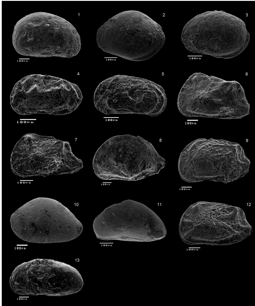
Fig. 2: 1) Xestoleberis paisi NASCIMENTO, 1989; 2) Loxoconcha stellisfera MÜLLER, 1894; 3) Loxoconcha rhomboidea (FISCHER, 1855); 4) Callistocythere oertlii NASCIMENTO, 1989; 5) Leptocythere azorica MEIRELES & GLIOZZI sp. nov.; 6) Hermanites memorans Moos subsp. vitreus Moos, 1966; 7) Hermanites dameriacensis KEU, 1958; 8) Aurila ( Euarila ) lariyensis MOYES, 1961; 9) Hemicythere sp. 1; 10) Neonesidea rochae NASCIMENTO, 1989; 11) Paracypris sp. 1; 12) Heliocythere magnei (KEU, 1953); 13) gen. et sp. indet.
