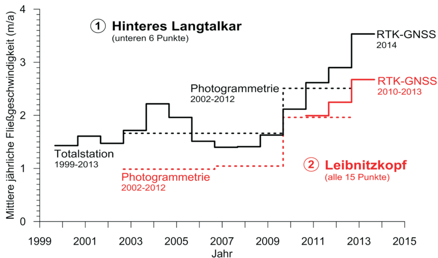
Abb. 4: Zeitlicher Verlauf der photogrammetrisch und geodätisch erfassten mittleren jährlichen Fließgeschwindigkeit markierter Punkte an der Oberfläche des Hinteren Langtalkar und des Leibnitzkopf Blockgletschers seit 1999 (basierend auf KAUFMANN 2015). Der Datenbestand wurde mit den photogrammetrischen Ergebnissen des Zeitintervalls von 2009 bis 2012 ergänzt. Fig. 4: Mean annual horizontal flow velocities of Hinteres Langtal Cirque and Leibnitzkopf rock glaciers since 1999 based on selected observation points using geodetical and photogrammetrically derived data (based on KAUFMANN 2015). The photogrammetrically derived data presented in this study covering the period 2009-2012 have been complemented.
