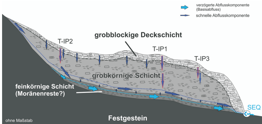
Abb. 2: Konzeptionelles Modell des reliktschen Schöneben-Blockgletschers (Längsprofil) mit einem dreischichtigen Aufbau (nicht maßstabsgetreu). T-IP1–T-IP3: Tracereingabepunkte; SEQ: Blockgletscherquelle. Längserstreckung des SRG ca. 700 m, Mächtigkeit des SRG von einigen Metern bis einige Zehnermeter (modifiziert nach WINKLER et al. 2016a).
