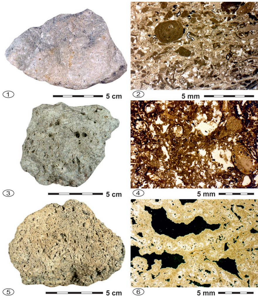
Abb. 6: „Exotische“ Bausteine und dazugehörige Dünnschliffbilder (1: Fossilschuttkalk, Leithakalk, Weissenegg-Formation; 2: Corallinaceen-Foraminiferen-Mollusken-Packstone; 3: Poröser „Sarmatkalk“ der Rollsdorf-Formation; 4: Extraklastenführender Gastropoden-Foraminiferen-Ostracoden-Rudstone; 5: Subrezenter „Kalktuff“ („Quellsinterkalk“); 6: Poröser Phytoklasten-Tuff).
