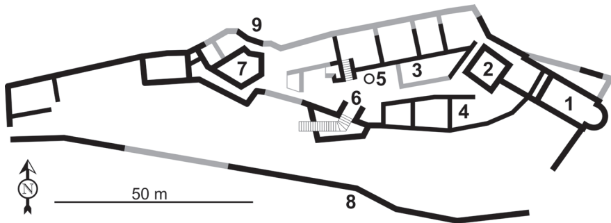
Abb. 3: Grundrissplan der Burganlage der Ruine Gösting (leicht verändert nach EBNER 1967). Zur näheren Untersuchung der Bausteine wurden die Südwestwand des ursprünglichen Palas (4) und die Südwestwand der Kapelle (1) näher aufgenommen (vgl. Abb. 7; 1: Burgkapelle; 2: Bergfried; 3: Großer Palas; 4: „Alter Palas“; 5: Zisterne; 6: „Inneres Burgtor“; 7: Fünfeckturm; 8: südliche Ringmauer; 9: nördliche Ringmauer; hellgraue Teile sind nicht mehr existent). Fig. 3: Ground plan of the Gösting castle complex (slightly modified after EBNER 1967). Mappings of building stones of the old hall (4) and the south-western front of the chapel (1) are illustrated in figure 7 (1: Castle chapel; 2: Castle keep; 3: Large hall; 4: “Old hall”; 5: Cistern; 6: “Inner castle gate”; 7: Pentagonal tower; 8: Southern curtain wall; 9: Northern curtain wall; light grey parts are no longer existent).
