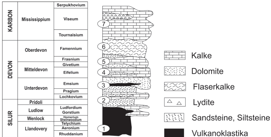
Abb. 1: Gesteinsfolge des Gebietes um die Burgruine Gösting. In einem Radius von ca. 1,5 km um den Burgenbereich treten fast alle lithostratigraphischen Einheiten der Rannach-Decke des Grazer Paläozoikums (vgl. EBNER & HUBMANN 2012) auf (1: Kehr-Formation; 2: Parmasegg-Formation; 3: Flösserkogel-Formation; 4: Plabutsch-Formation; 5: Kollerkogel-Formation; 6: Steinberg-Formation; 7: Sanzenkogel-Formation).
