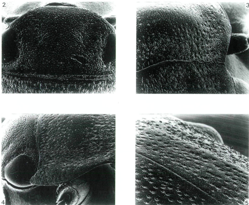
Figs. 2 - 5: Deronectes fosteri sp.n., 2) head, 3) pronotum, dorsal view, 4) pronotum, lateral view, 5) right elytron.
